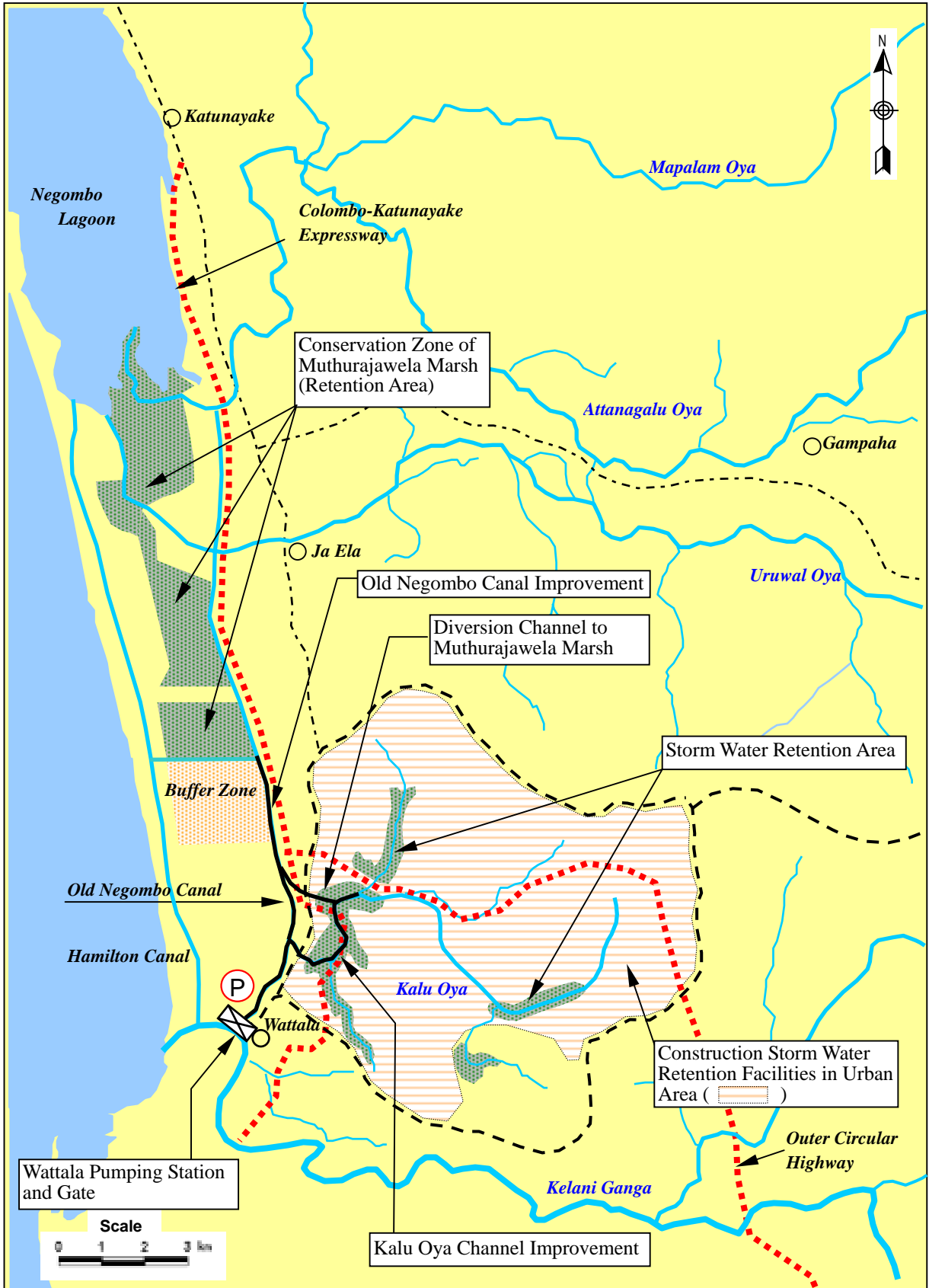
図 4.4 カルオヤ流域洪水対策案
