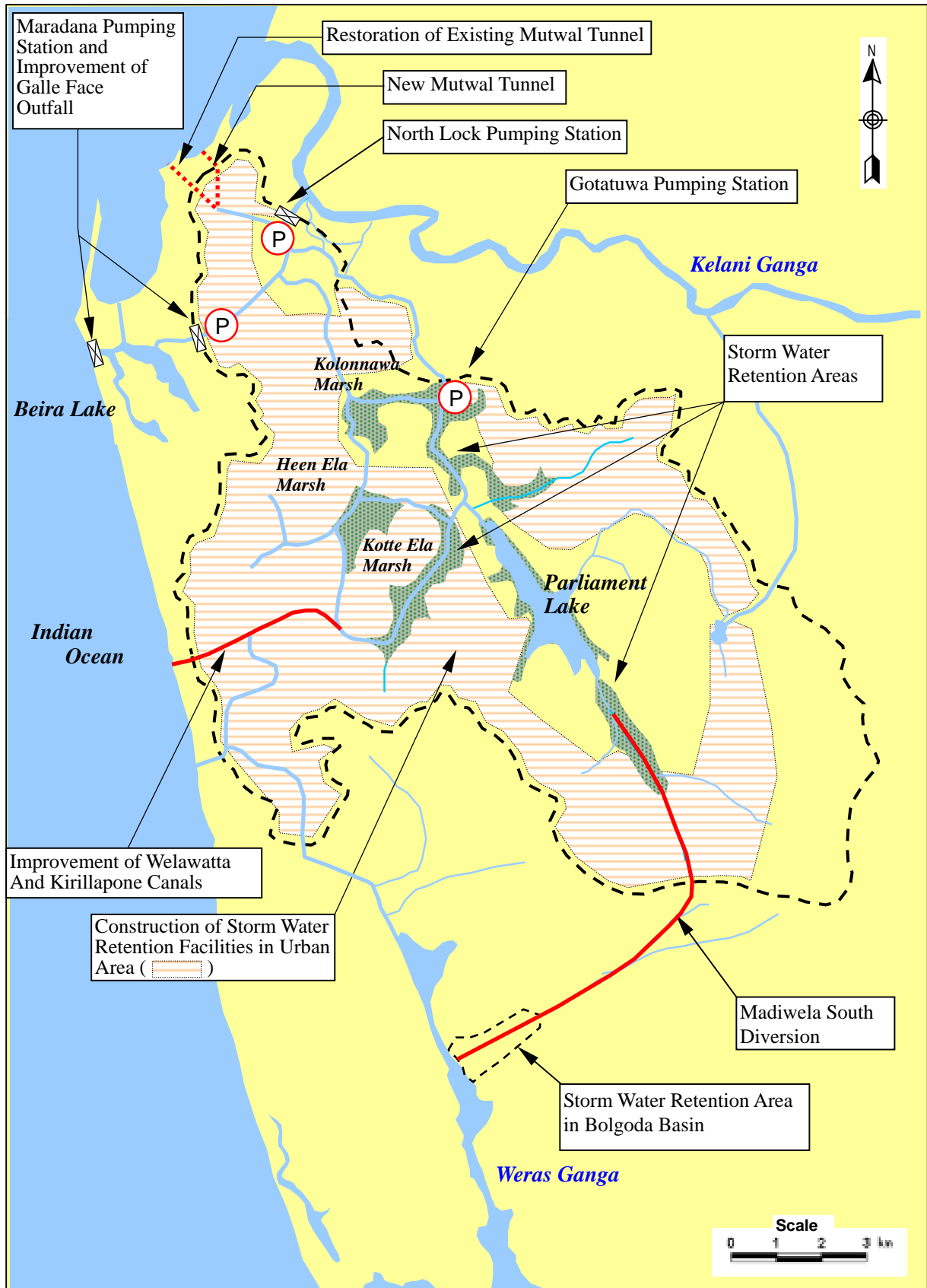
図 4.6 大コロombo流域洪水対策案
