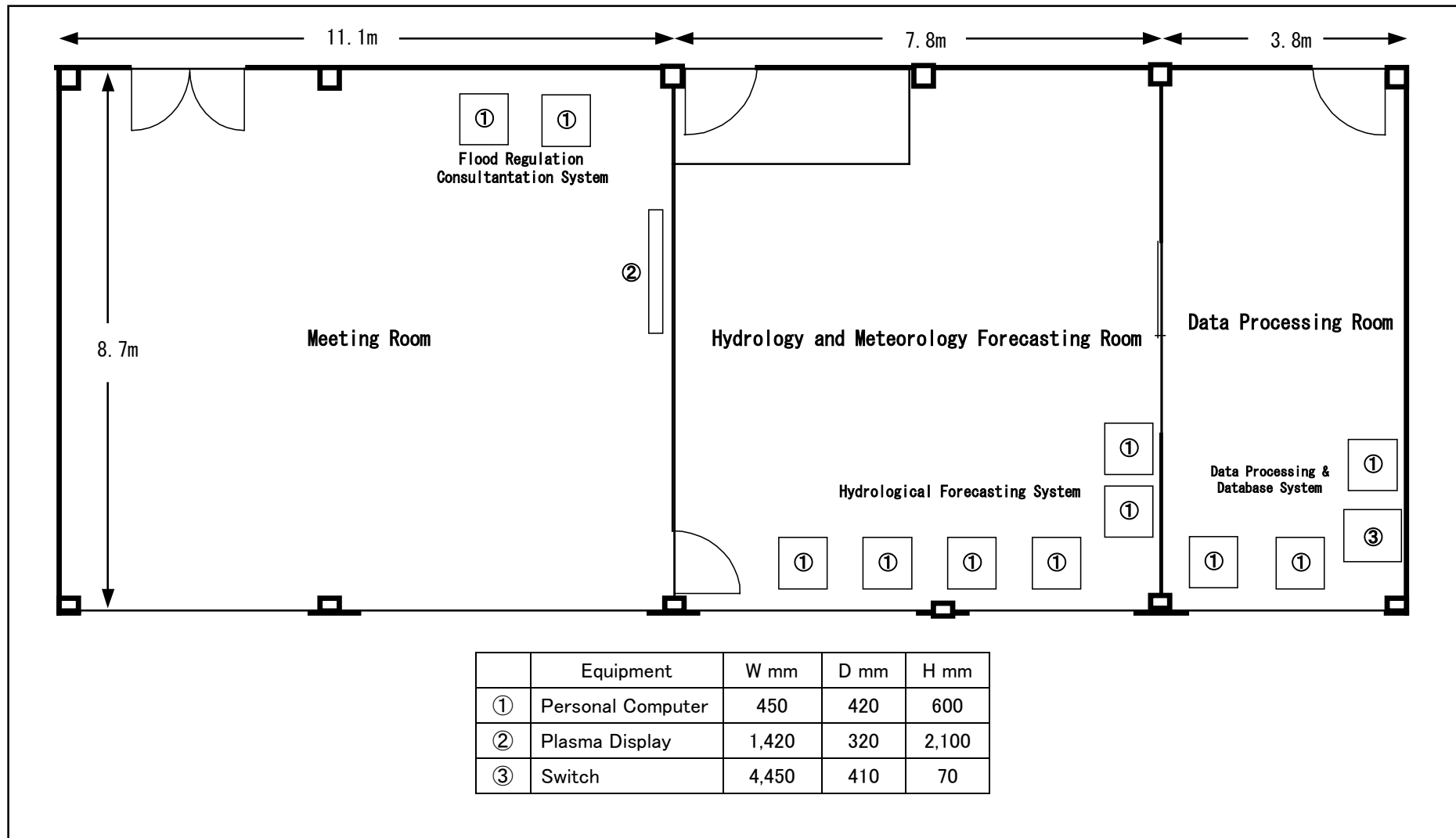
図 2-2-18 A システムコントロールセンター(中央局)16階フロアレイアウト
