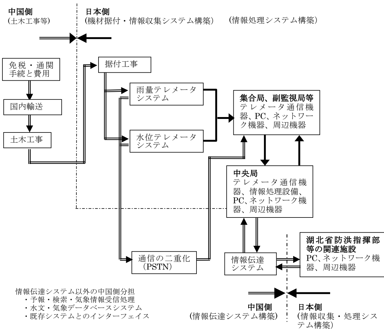
図 2-2-20 施工区分／調達・据付区分
