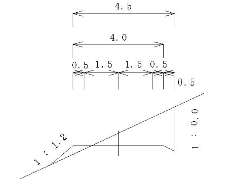
図-5 林道横断面図の一例
