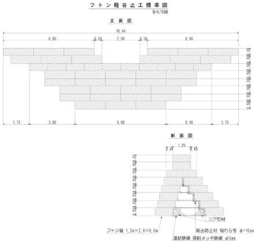
図-7 谷止工の一例
