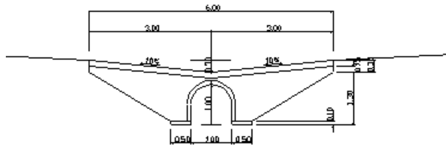
図-6 洗越の一例
