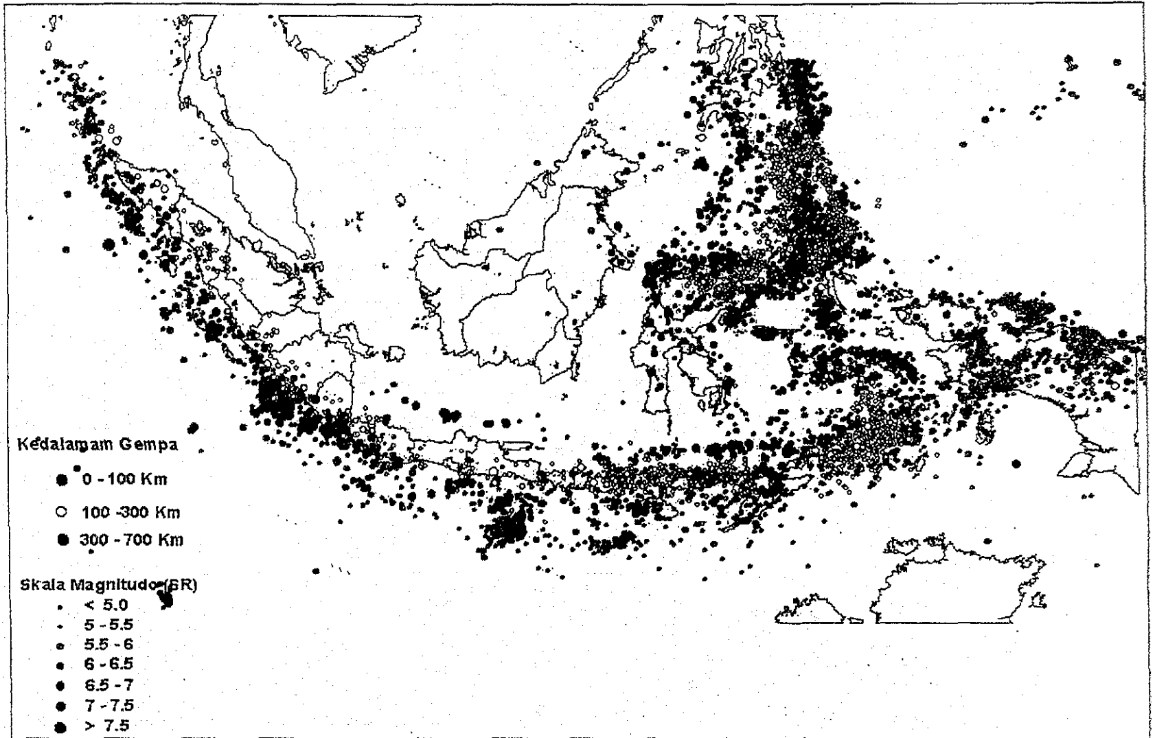
Figur 2.1.2 Peta Distribusi Gempa Bumi di Indonesia (1999-2000)
