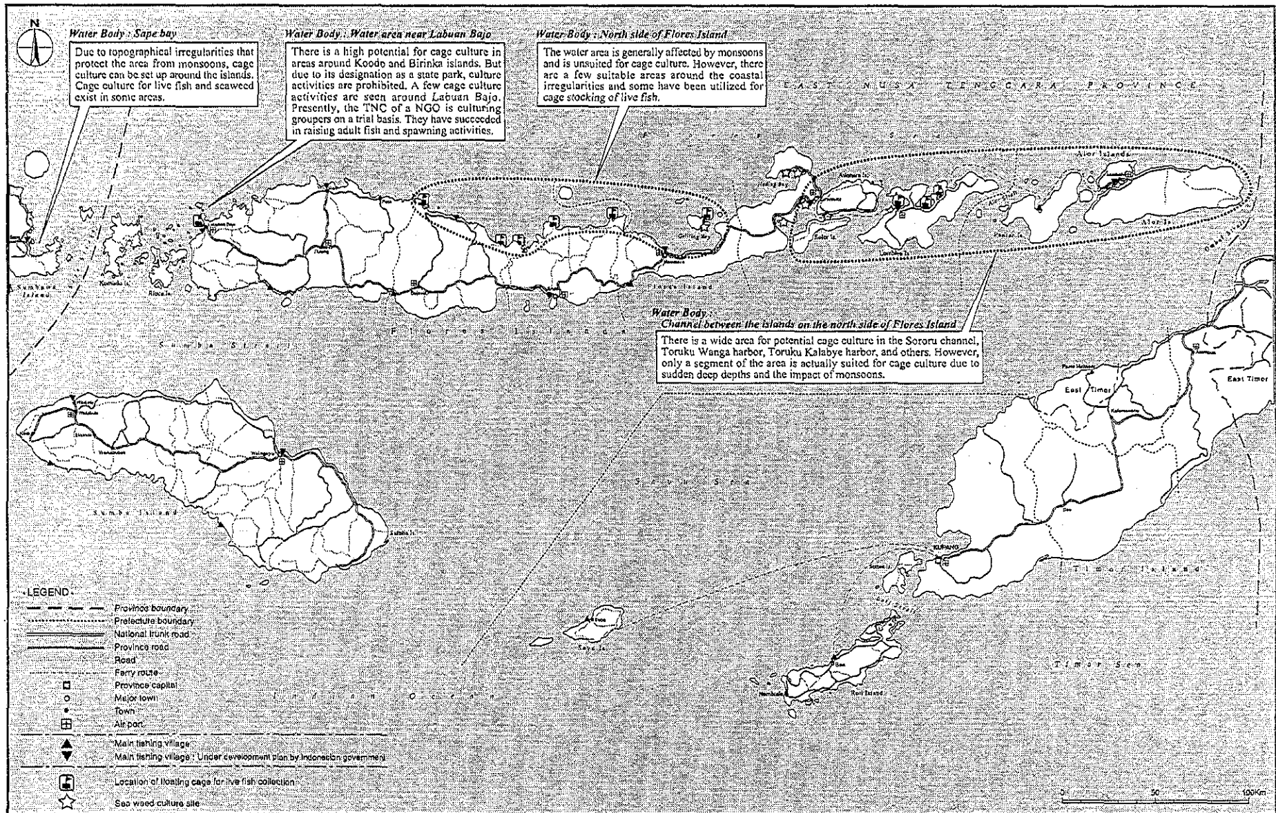
Fig. 2.5.1 Peta Potensi Budidaya Laut (Zona Timur)
