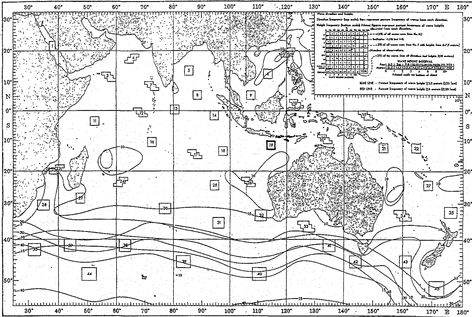
Figur 2.1.1 (1) TitikObservasi Ombak di Samudera Indian
