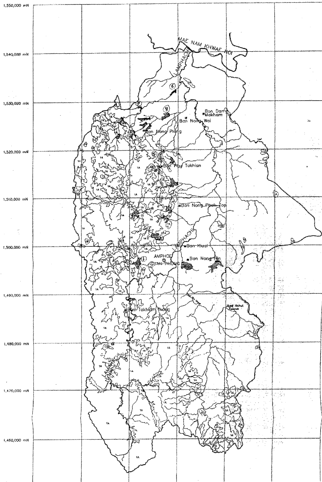
图 5 - 3 中規模貯水池計画位置図
