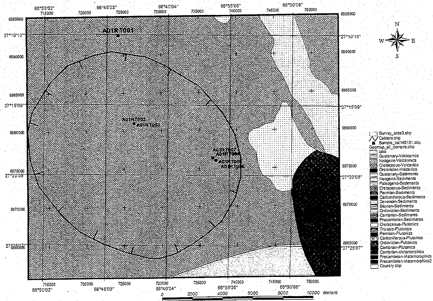
Fig.A-1-31 Sample point of Bajo de la Alumbraera deposit and Bajo El Durazno mineral showing
