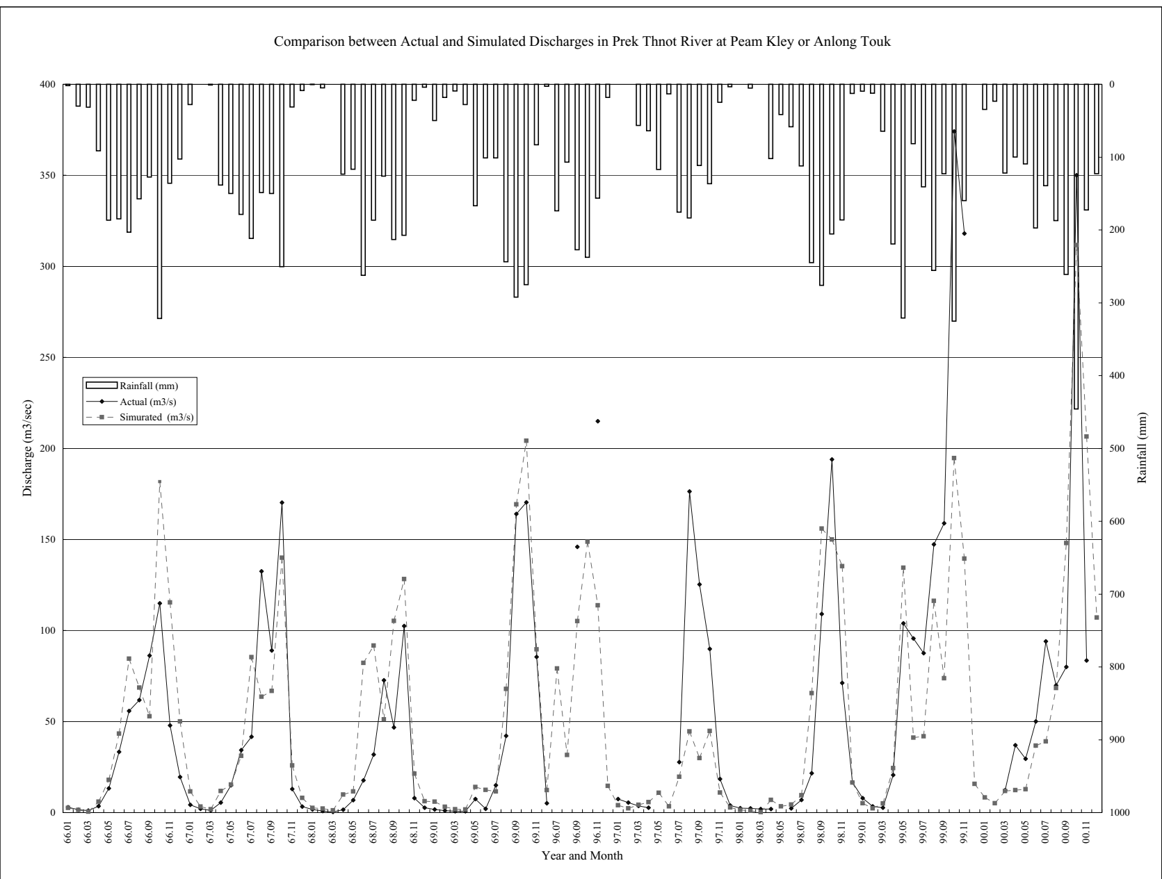
図 II-1.3.2 Prek Thnot 川の 実測流量とシミュレーション 流量との比較
