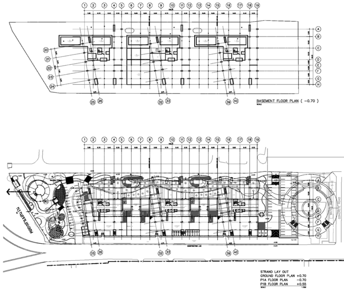
Strand Layout Plan (Basement ~ P1B)
