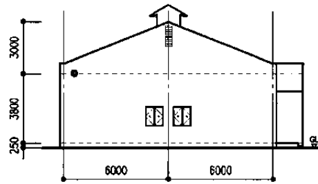
西立面図
