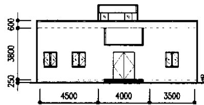
北立面図
