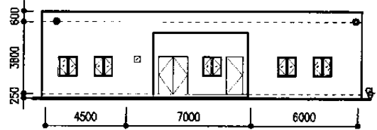
南立面図
