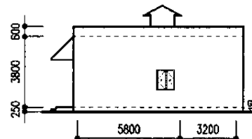
南立面図
