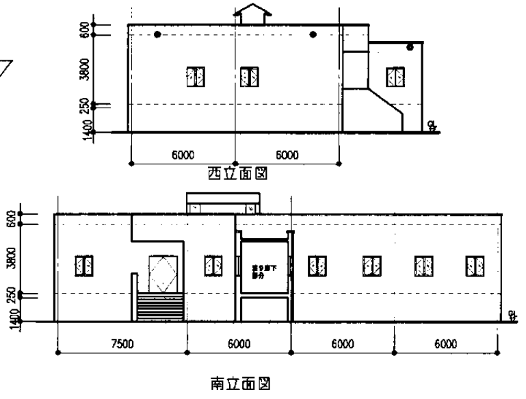
配置図 1/1000 立面図 1/300
