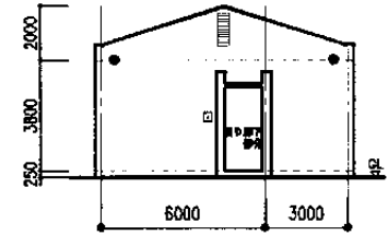
東立面図
