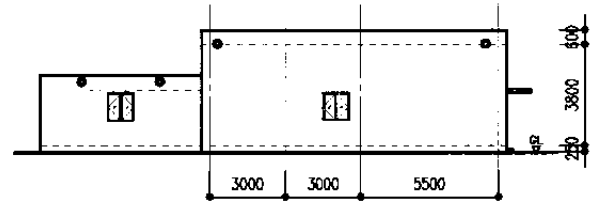
西立面図
