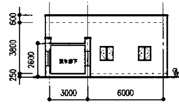
西立面図
