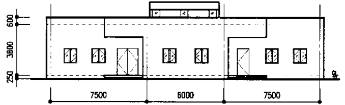
南立面図
