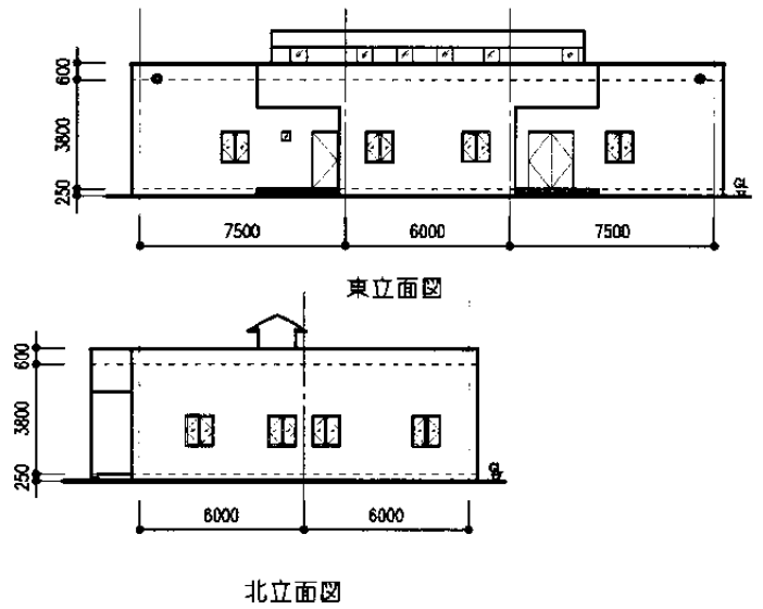
配置図 1/1000 立面図 1/300
