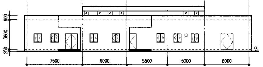
東立面図
