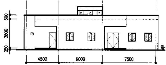
東立面図
