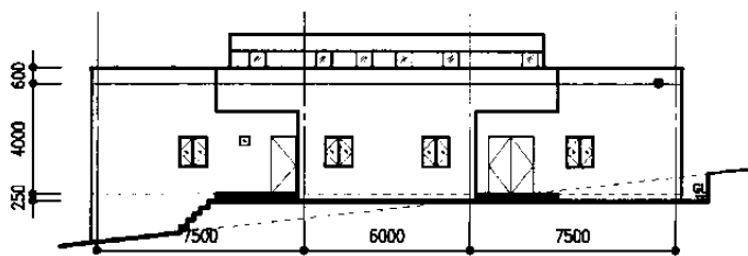
西立面図
