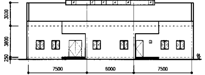
南立面図
