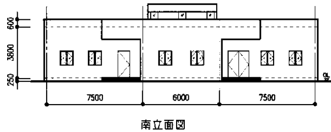
配置図 1/1000 立面図 1/300
