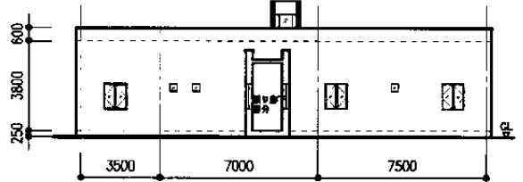
西立面図
