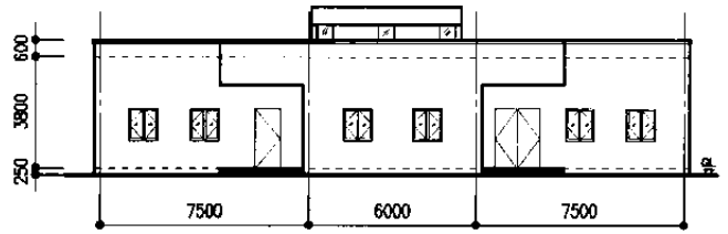
北立面図
