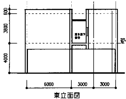
東立面図
