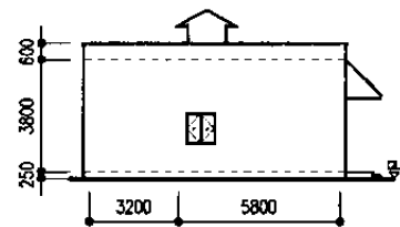
東立面図
