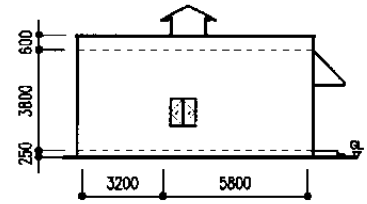
東立面図
