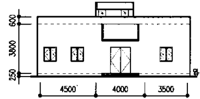
北立面図
