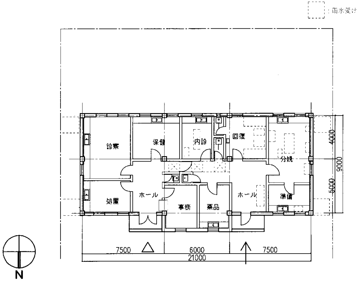
平面図 1/200 No.17 ティサリン保健センター (Tighsline)
