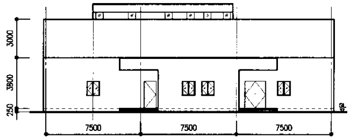
西立面図
