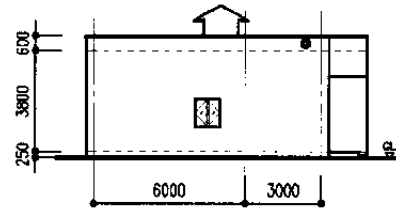
西立面図
