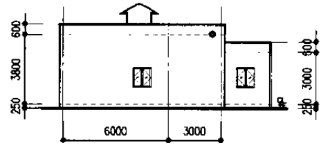
西立面図
