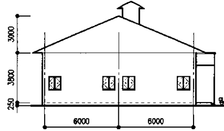
北立面図
