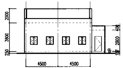
南立面図
