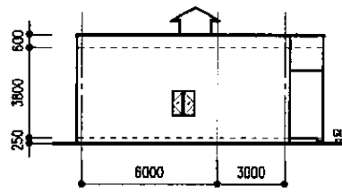
東立面図
