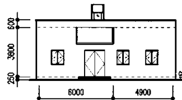
西立面図
