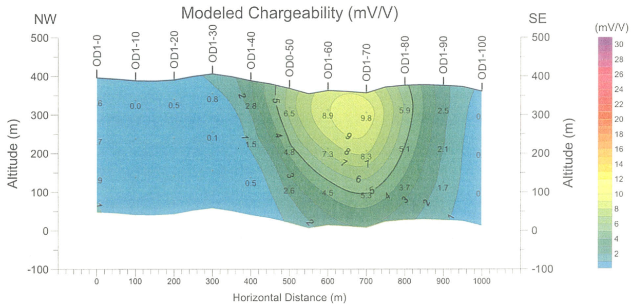
图 98 比抵抗・分極率シミュレーション断面図 (測線 OD1)
