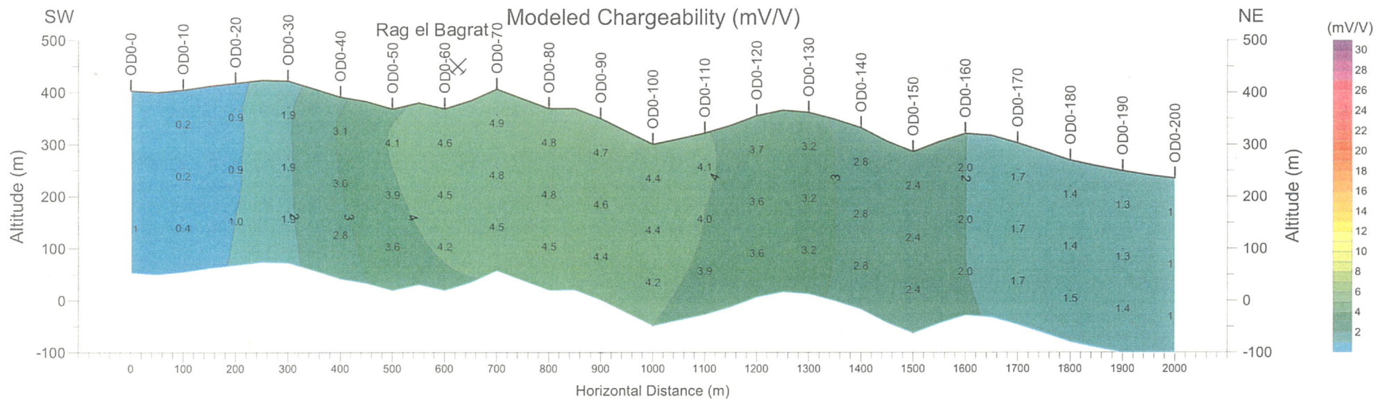
図 97 比抵抗・分極率シミュレーション断面図 (基線 ODO)
