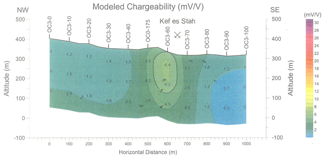
図 95 比抵抗・分極率シミュレーション断面図 (測線 OC3)
