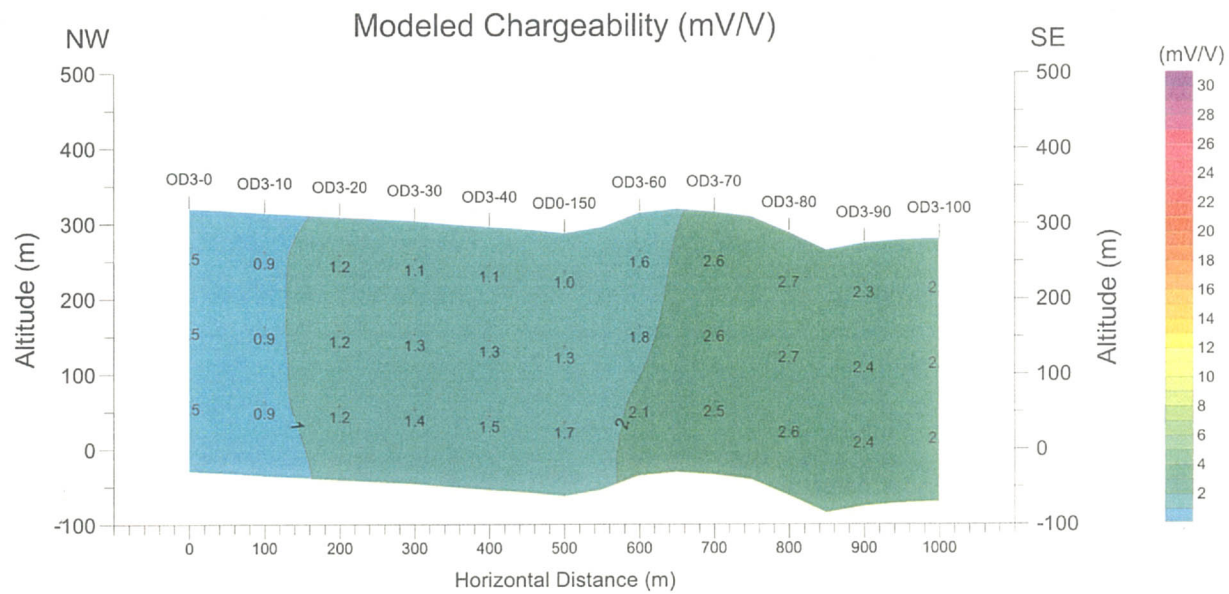
図 100 比抵抗・分極率シミュレーション断面図（測線 OD3）
