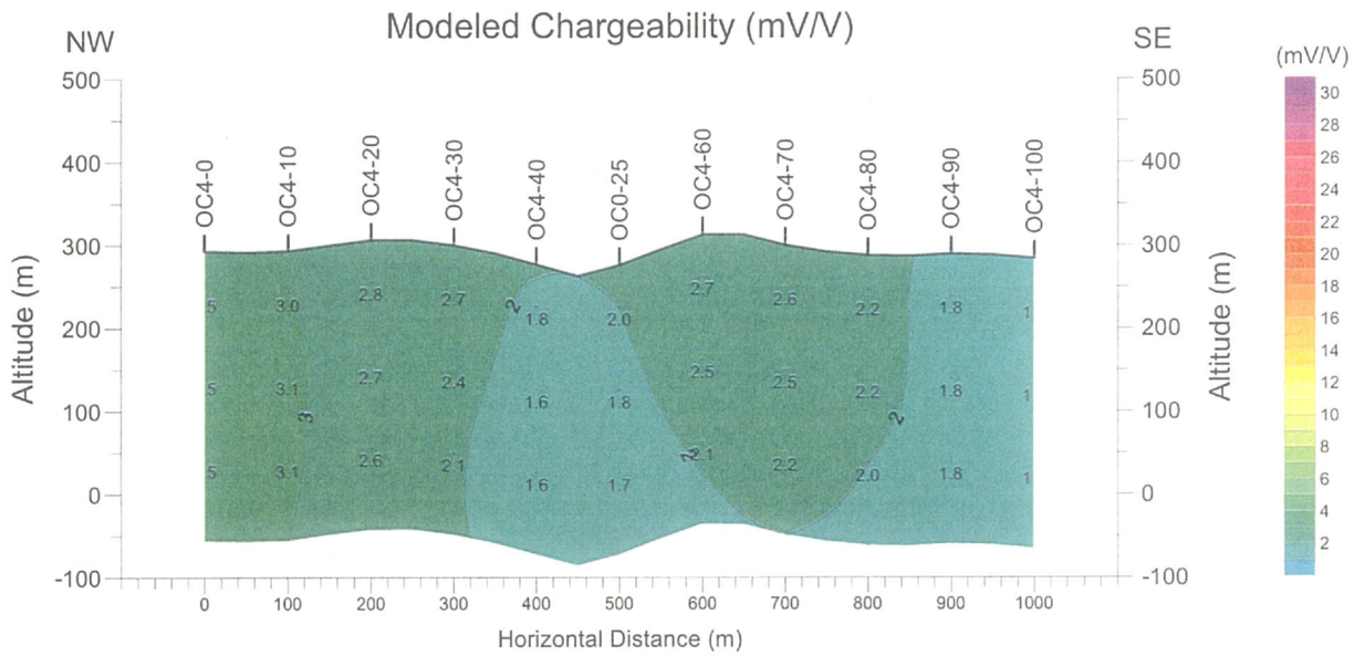
図 96 比抵抗・分極率シミュレーション断面図 (測線 OC4)
