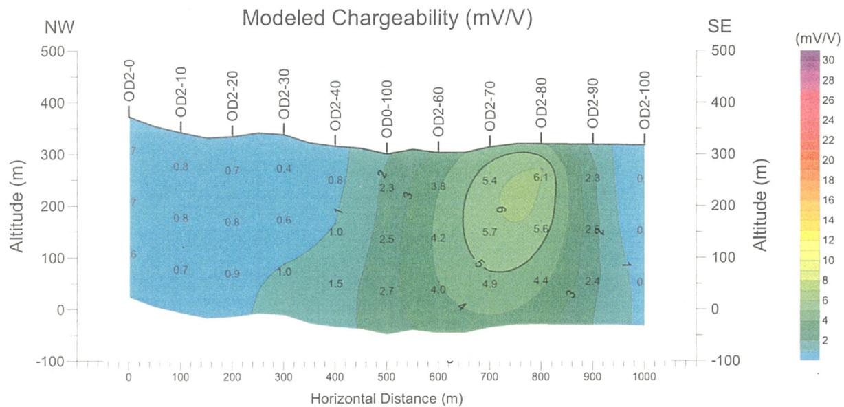
図 99 比抵抗・分極率シミュレーション断面図 (測線 OD2)
