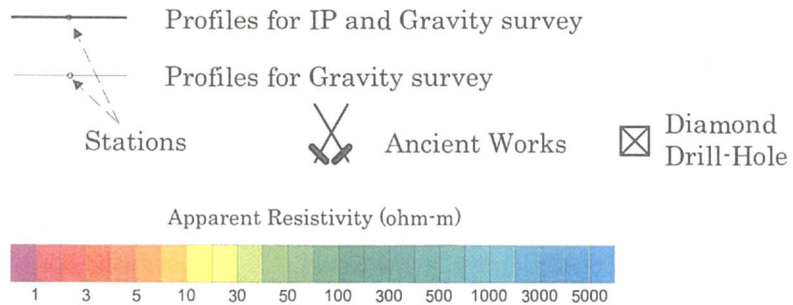
図 69 ウェド・ジェブス OB 地区見掛比抵抗平面図 (n=2)
