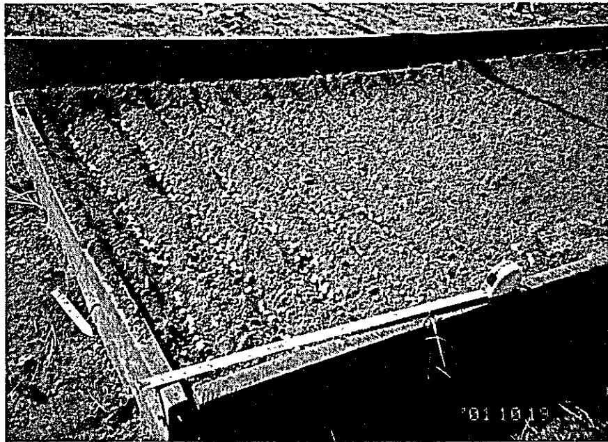
写真No.24 筋播き作業 (P.gigante の種子)
