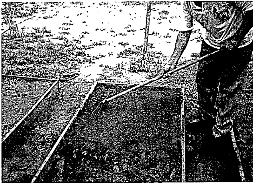
写真No.2 藩き付け床作り（枠平床）
