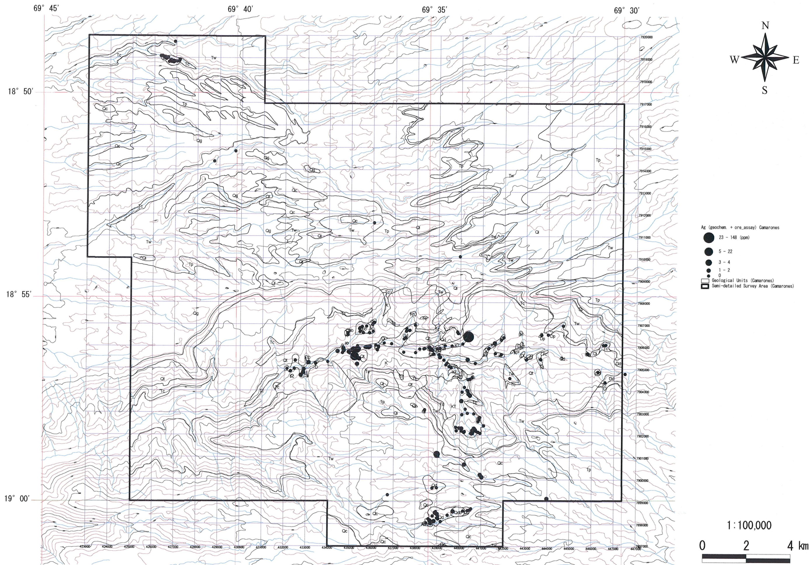
Fig. 2-2-43 (2) Geochemical Anomaly Map in the Camarones Area (Ag)
