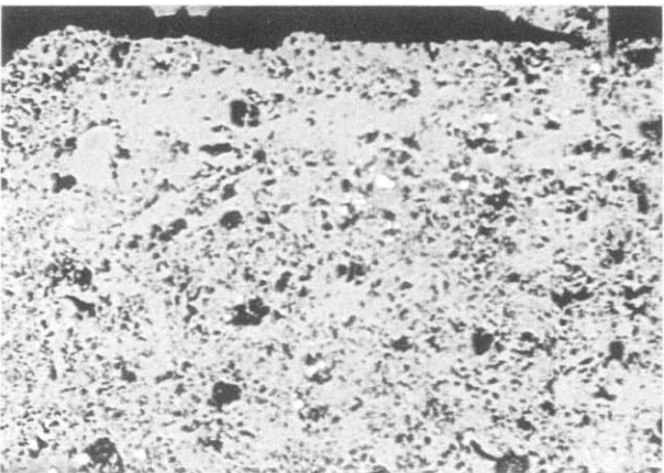
Ph 1 4 乾留品の顕微鏡写真(550°C)
