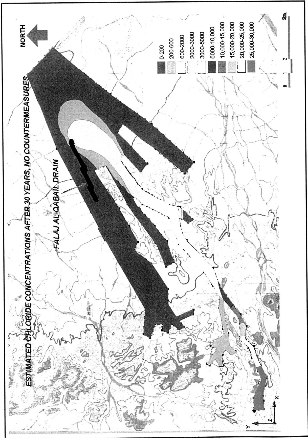
図 7.10 地下水シミュレーション結果：現状のままでの 30 年後の塩分濃度分布
