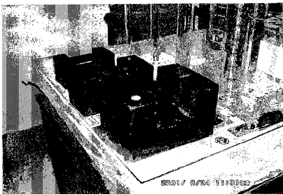
カンボジアMOI, 20kg, 10kg, 5kgの各標準機
