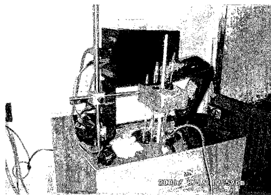
QUATEST-3 温度計校正試験
