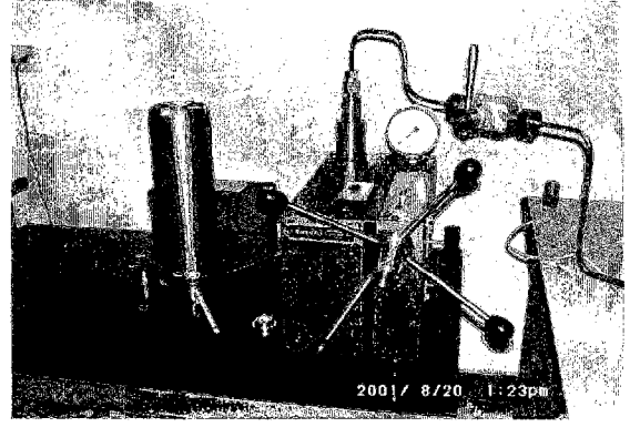
VMI、圧力標準機
