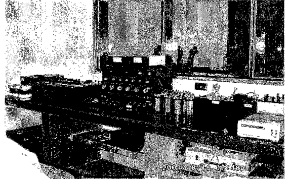
QUATEST-3 電気計測用抵抗器標準機
