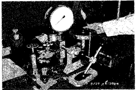
ミヤンマMOI, 圧力標準機
