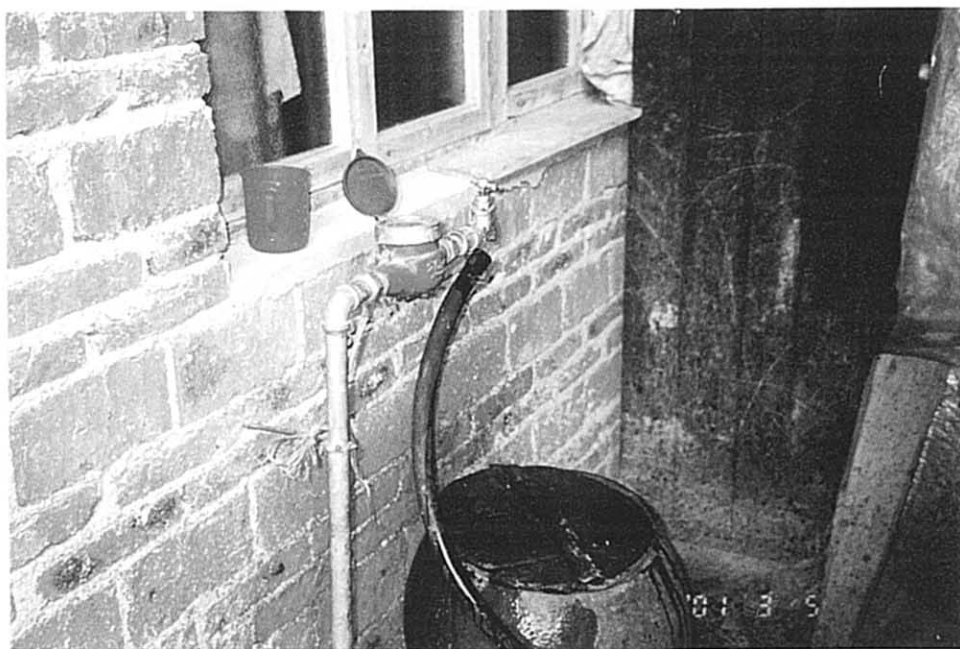
民家に設置された量水器と給水栓 要請内容は量水器までの材料となっている
