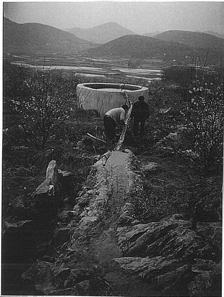
白宝郷 カルスト地形における湧水の水槽 (渇水期の補助供給用) への送水
