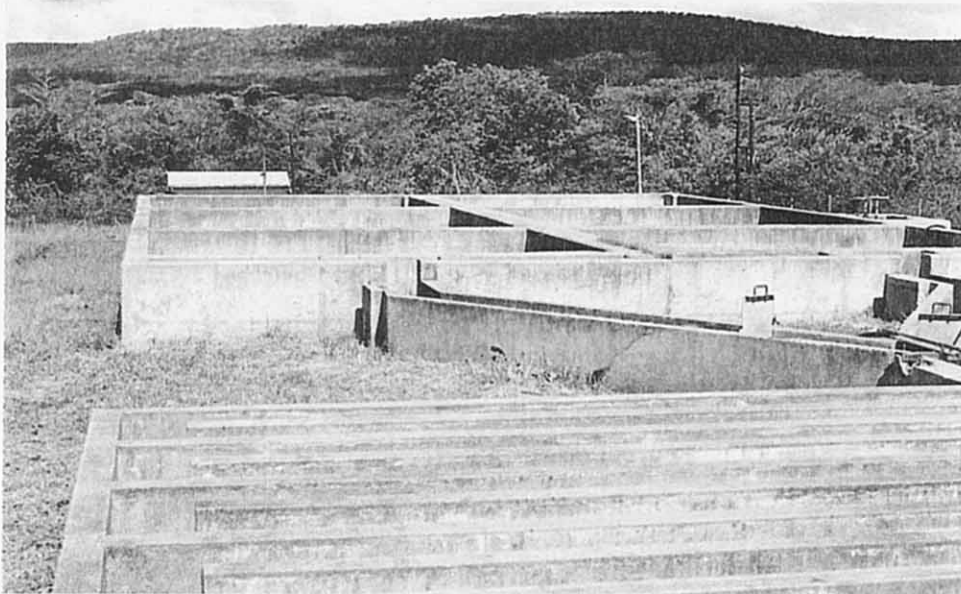
写真14 Mangedla 浄水場のフロック 形成池と沈でん池 (Water Service Corporation) Lubombo 県
