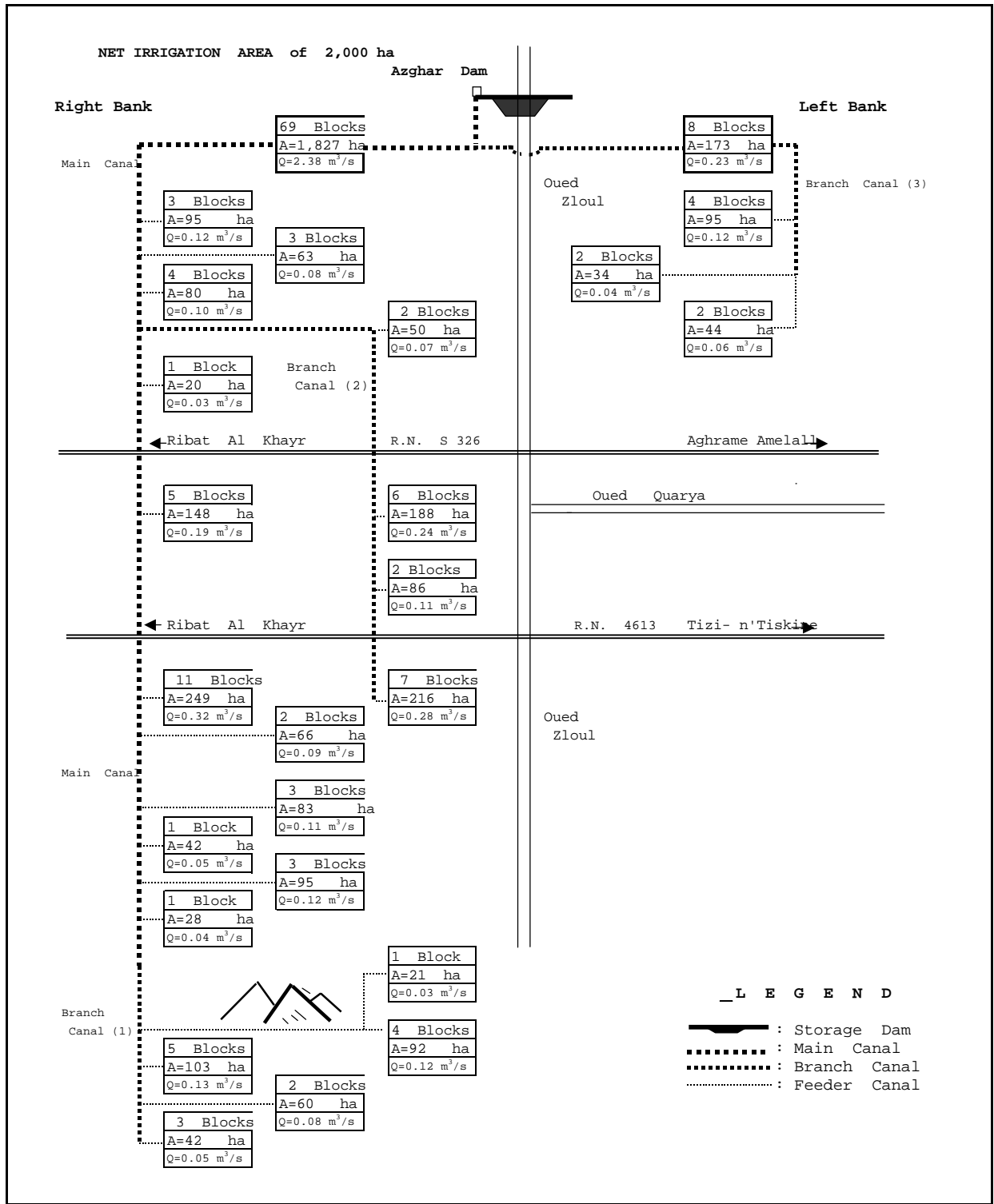
Figure 9.1.12 Diagramme des Systèmes d'Irrigation d'Azghar
