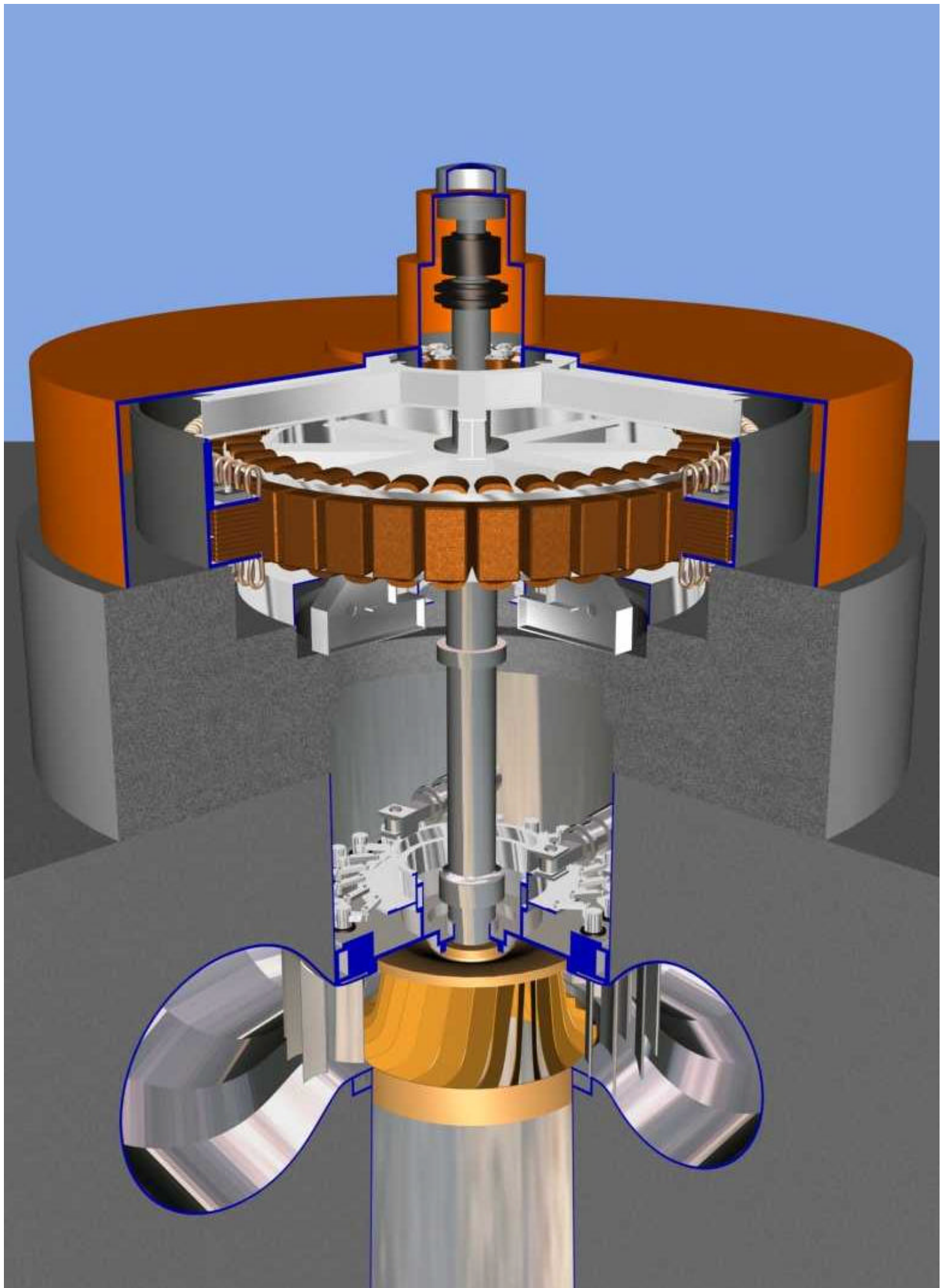
ナムグム第一水力発電所 水車発電機（1・2号機）
