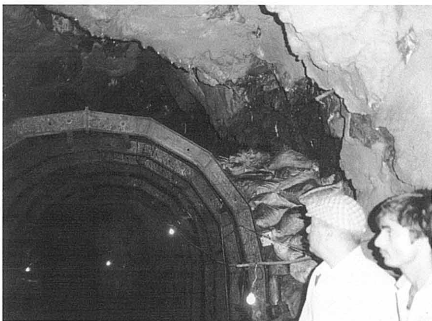
試掘横坑(内部)
