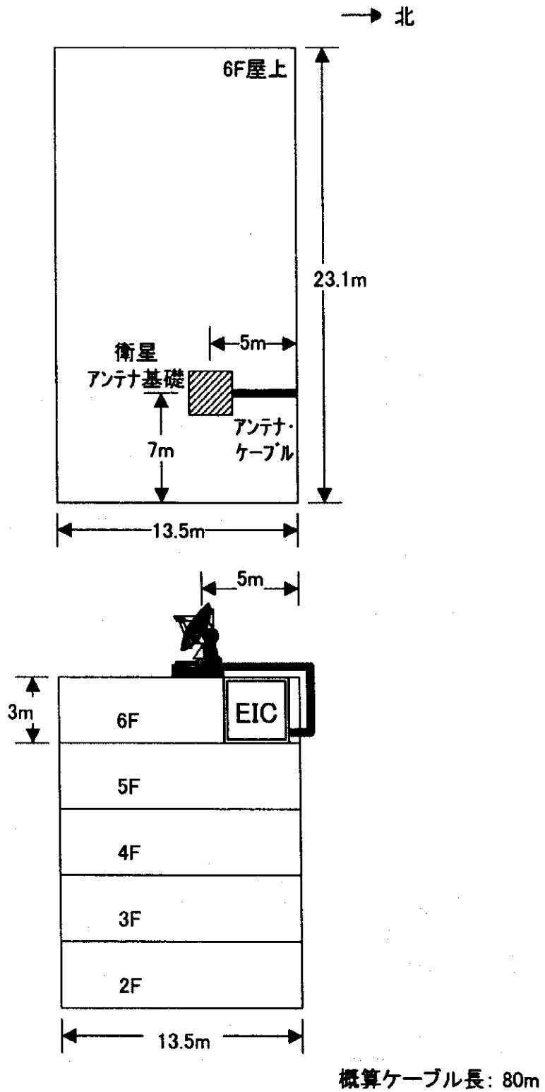
衛星通信用アンテナ配置図
