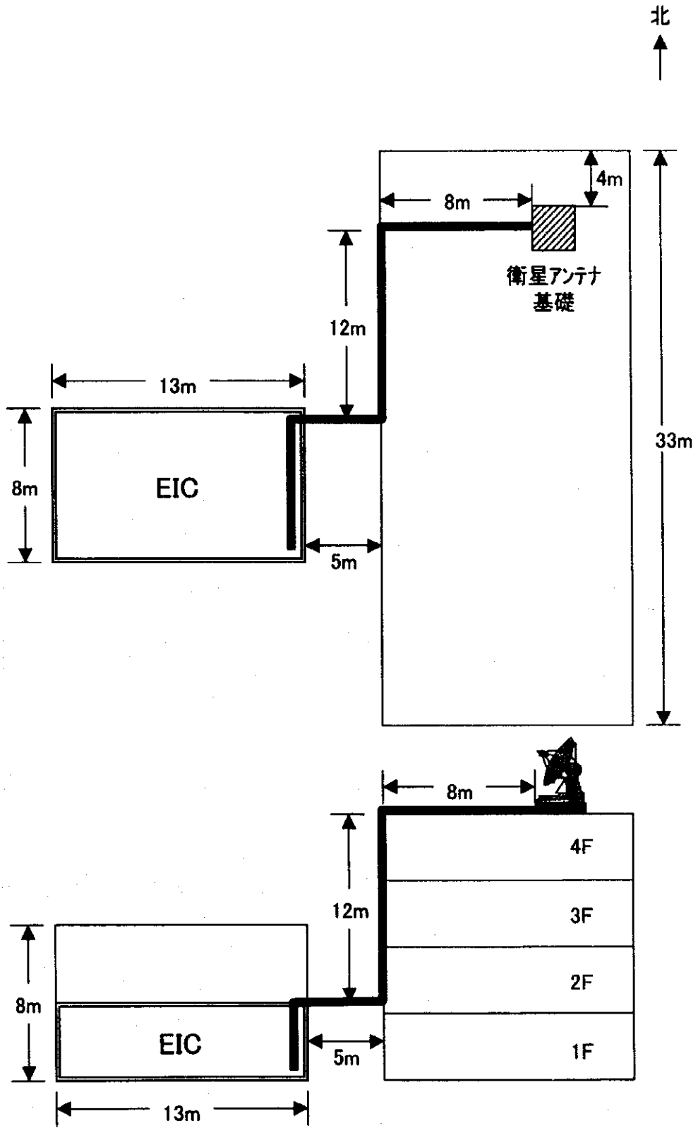
衛星通信用アンテナ配置図
