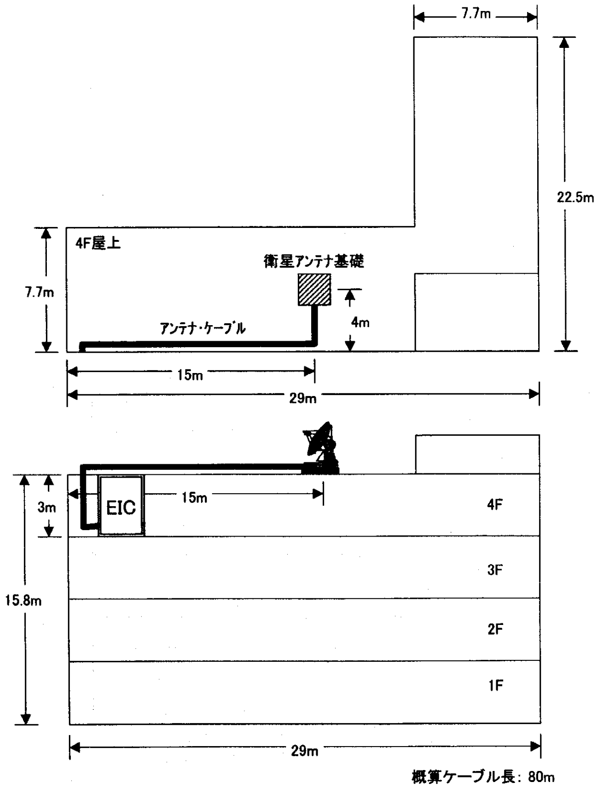
衛星通信用アンテナ配置図
