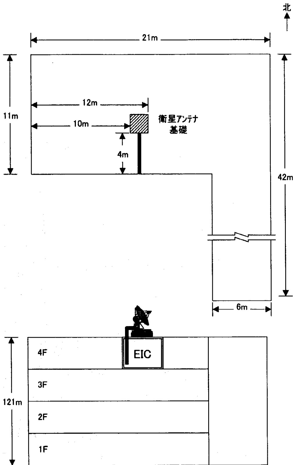
衛星通信用アンテナ配置図
