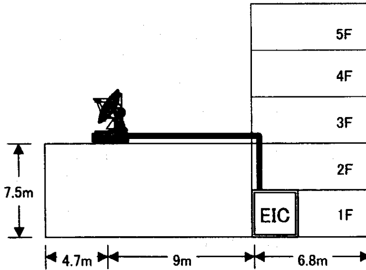
衛星通信用アンテナ配置図
