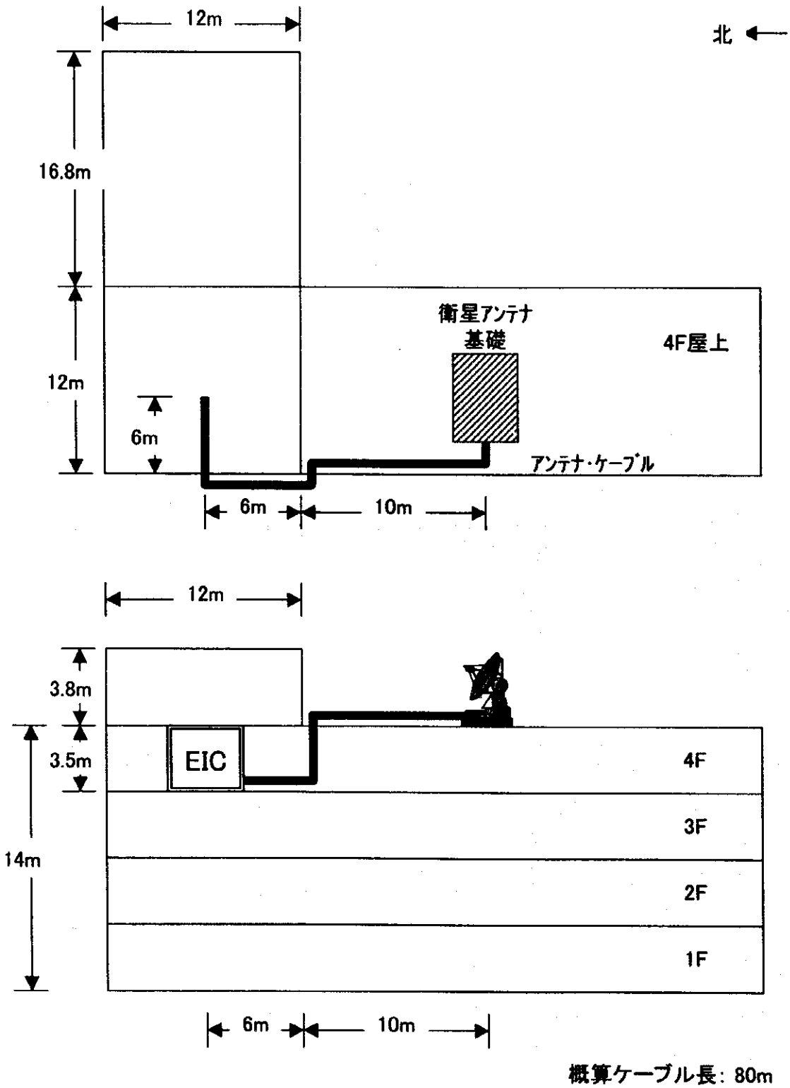
衛星通信用アンテナ配置図
