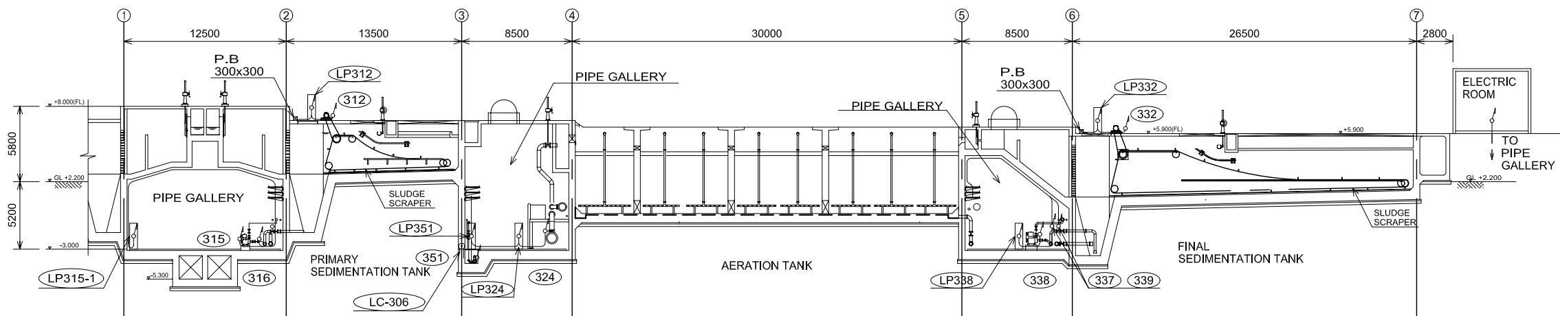
SECTION A-A
