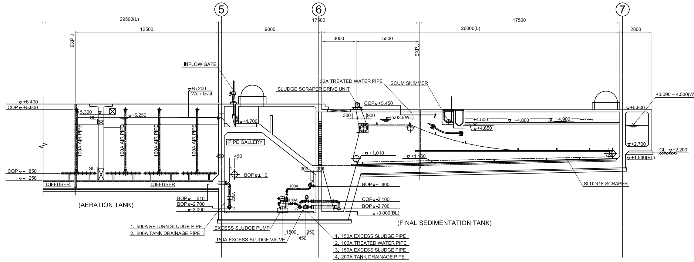
SECTION A-A
