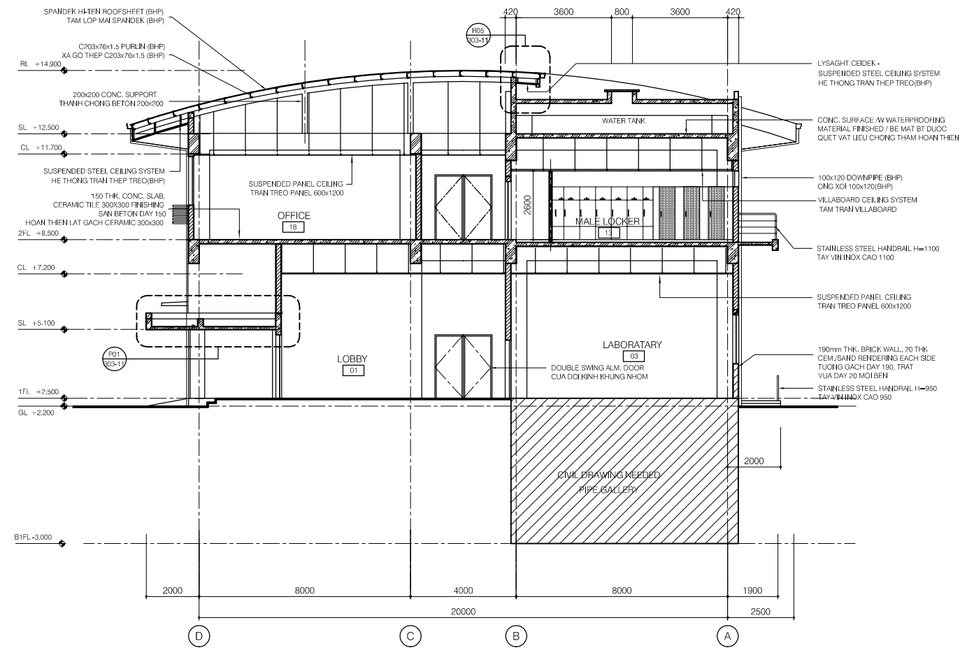
SECTION A-A
