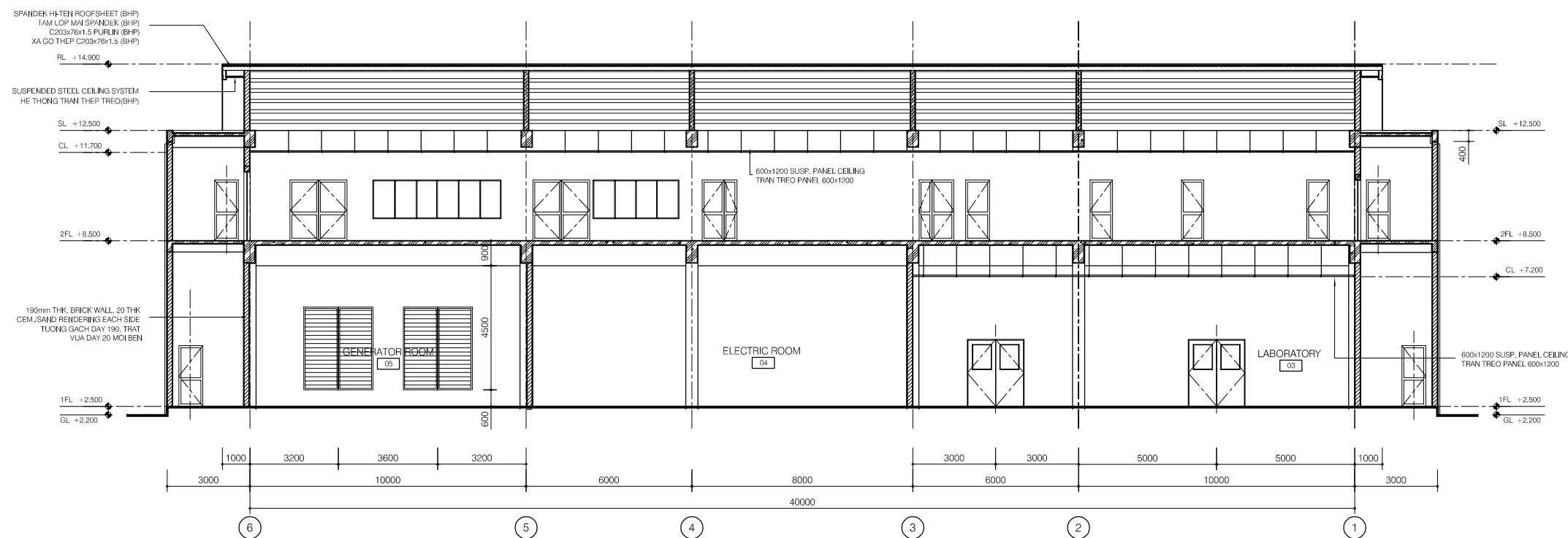
SECTION D-D
