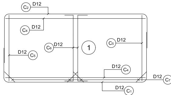
BAR SKELETON @125
