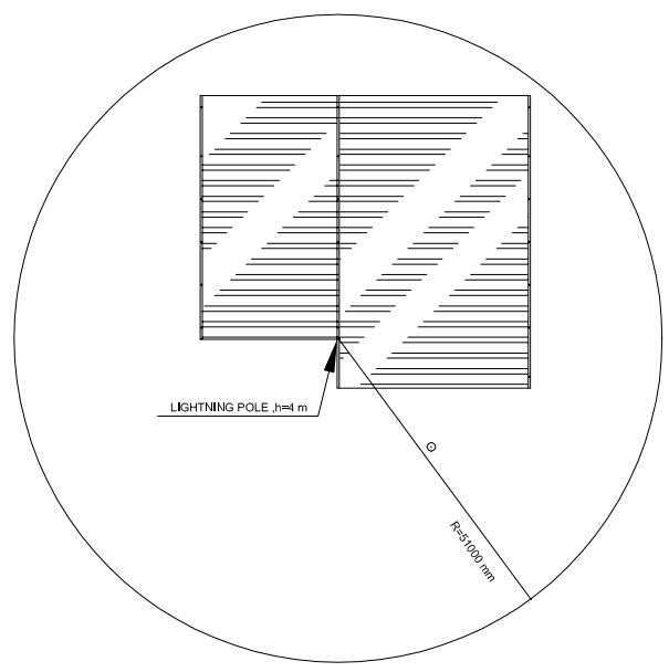
LIGHTNING PLAN N.T.S.
