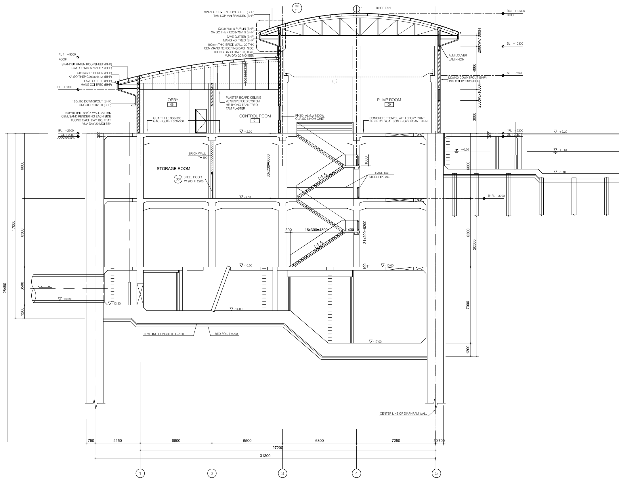
SECTION A-A
