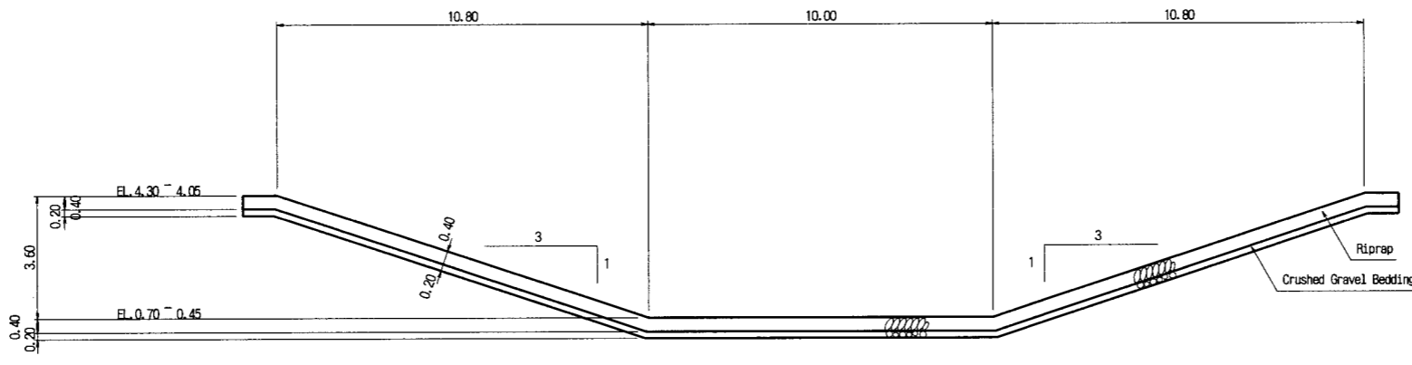
SECTION A-A SCALE 1:200
