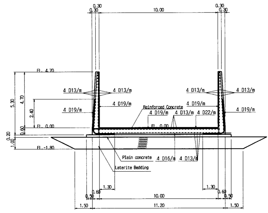
SECTION A-A SCALE 1:200
