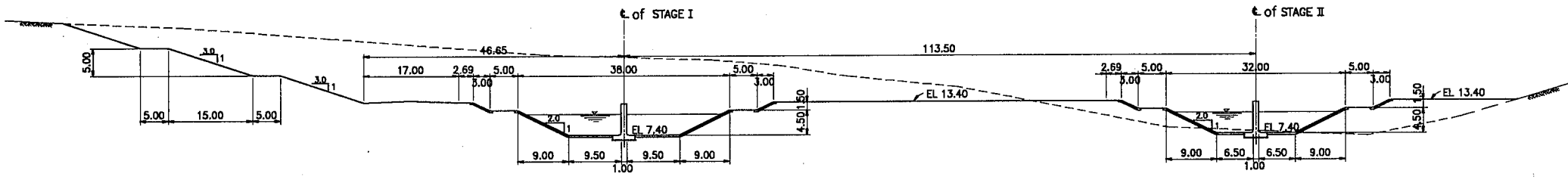
SECTION E - E S=1/1000
