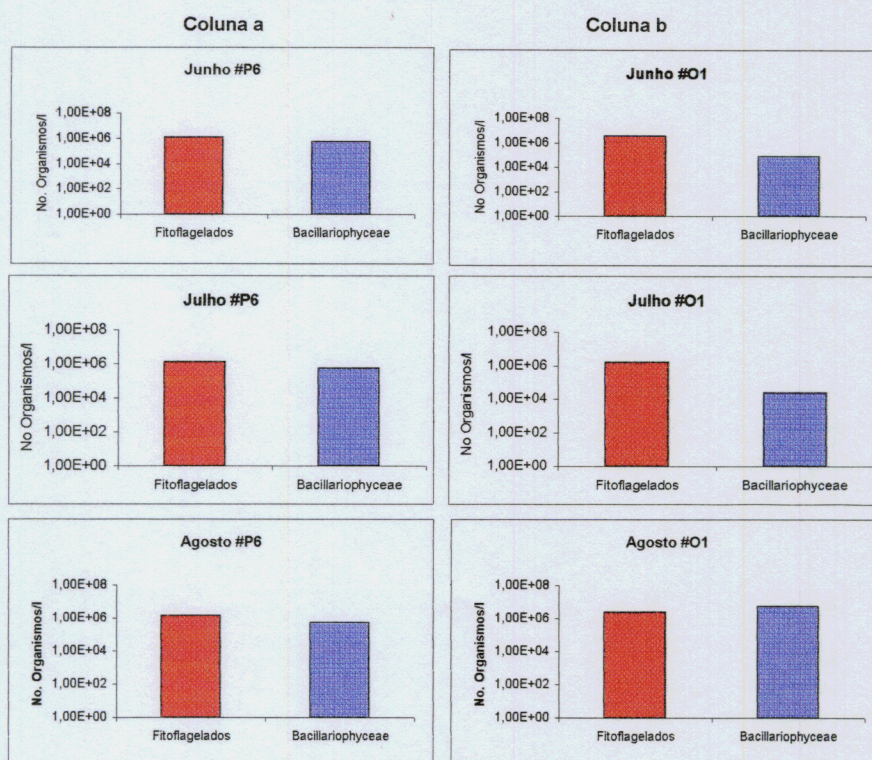
Figura 4 (cont): Número de fitoflagelados/l x No. de diatomáceas (Bacillariophyceae)/l nas estações P6 (coluna a) e para a estação O1 (coluna b) na superfície. Os fitoflagelados incluem, neste caso, as Classes Dynophyceae, Cryptophyceae, Prasinophyceae, Raphidophyceae, Dictyocophyceae, Euglenophyceae e Chrysophyceae.
