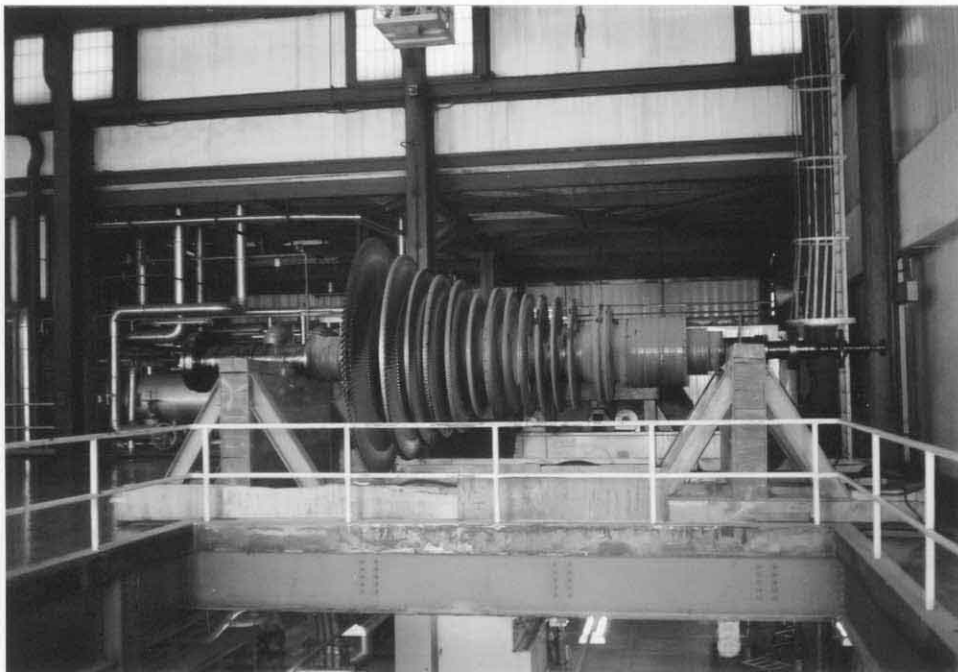
タービン
