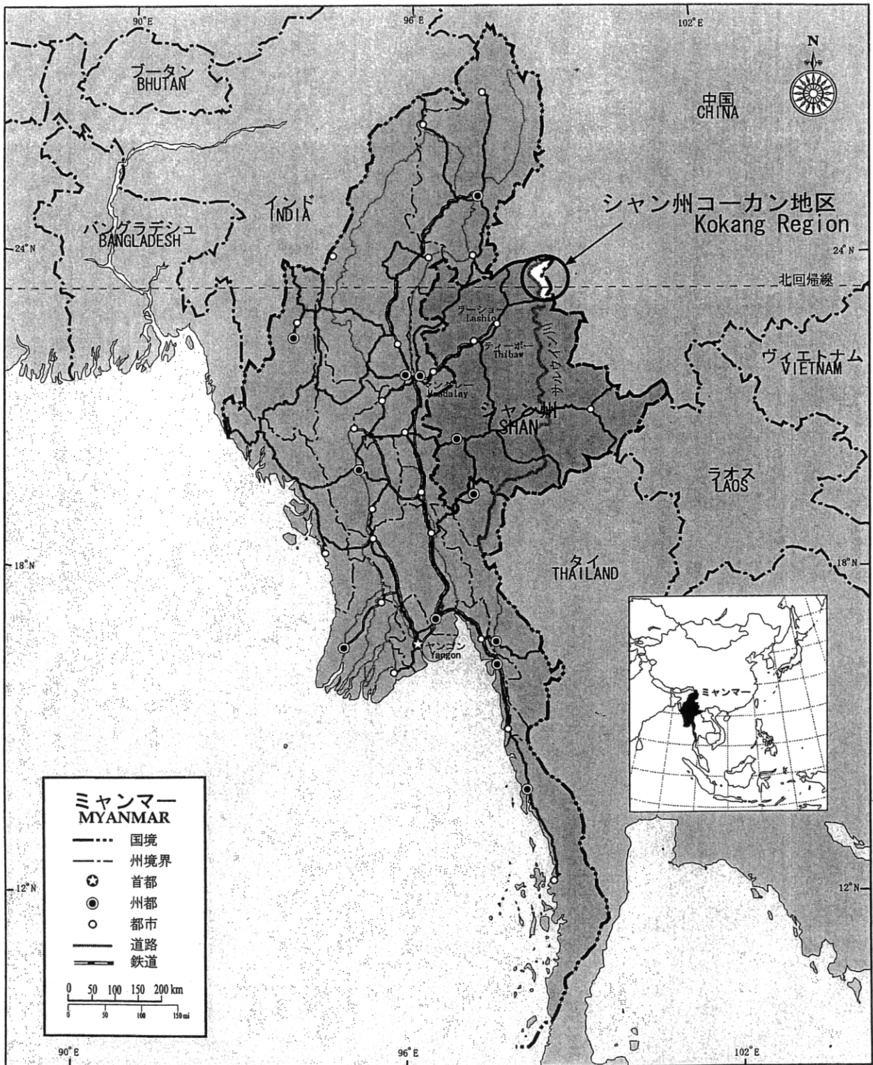
ミャンマー国シャン州コーカン地区位置図
