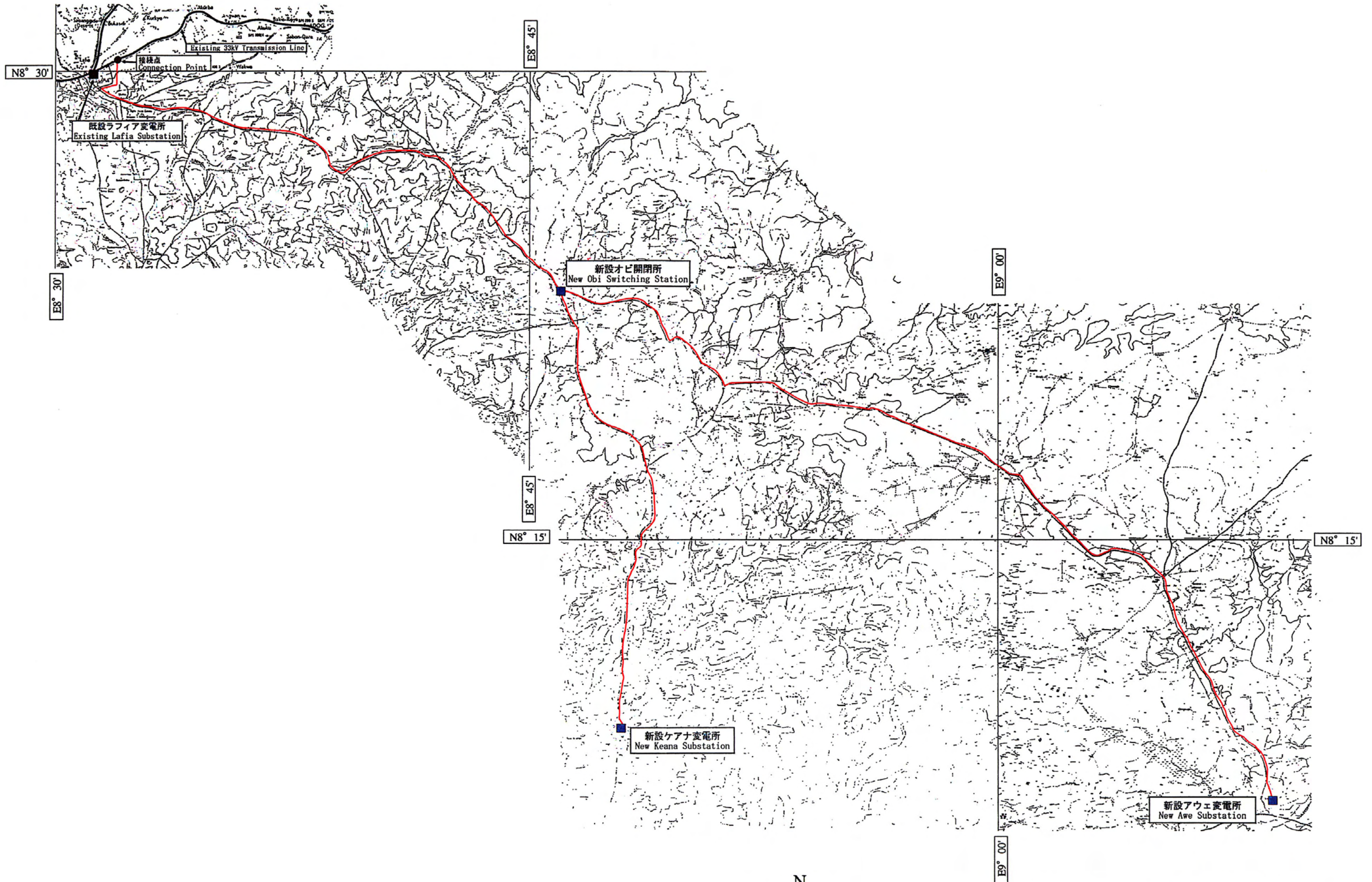
DWG. No. NAS-T3: 33kV送電線ルート全体図 [ナサラワ州 アウェ町、ケアナ町] Key Map of 33kV Transmission Line [Awe and Keana Towns in Nassarawa State]
