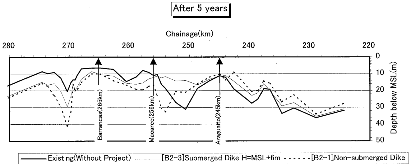
Fig. 7-3-8 Perfiles Longitudinales del Cambio en la Elevación del Lecho para [B2-1] y [B2-3]
