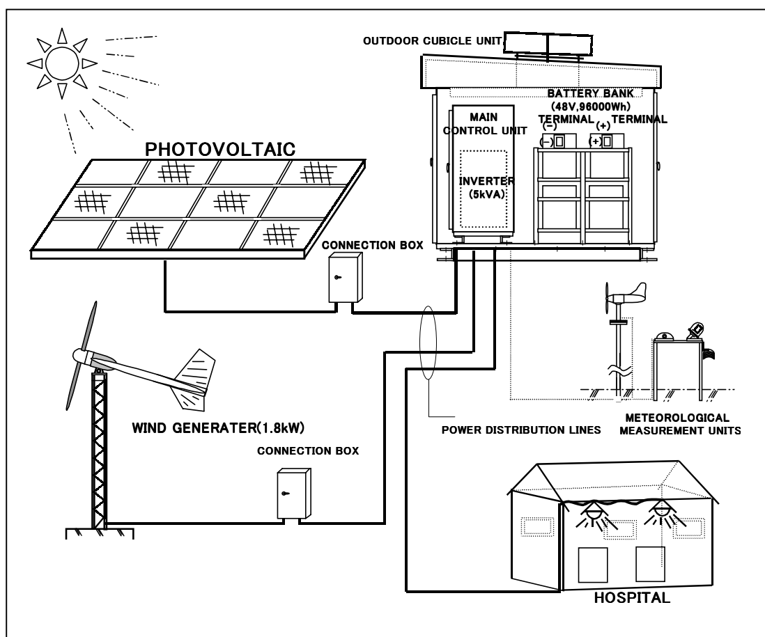
図Ⅱ.1.1 パイロット・プラントの構成図
