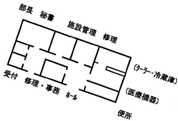
DIEMワークステーション棟 平面図 s 1:500
