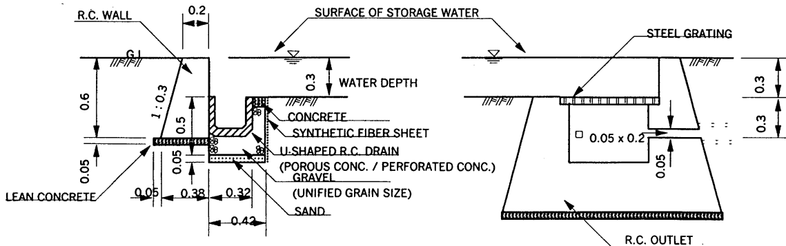
図 2-5 公共公益施設のオンサイト貯留概要図
