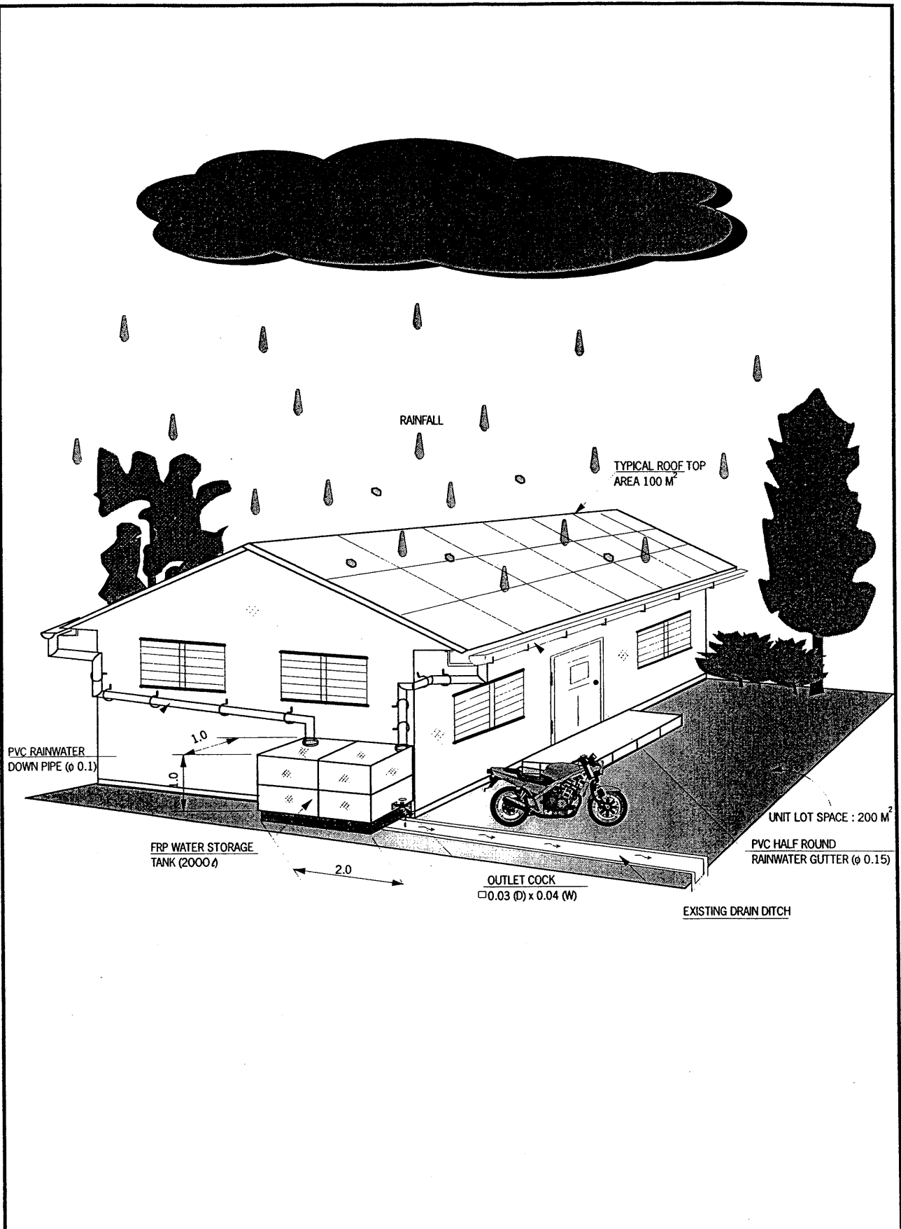
図 2-4 各戸貯留システム概念図
