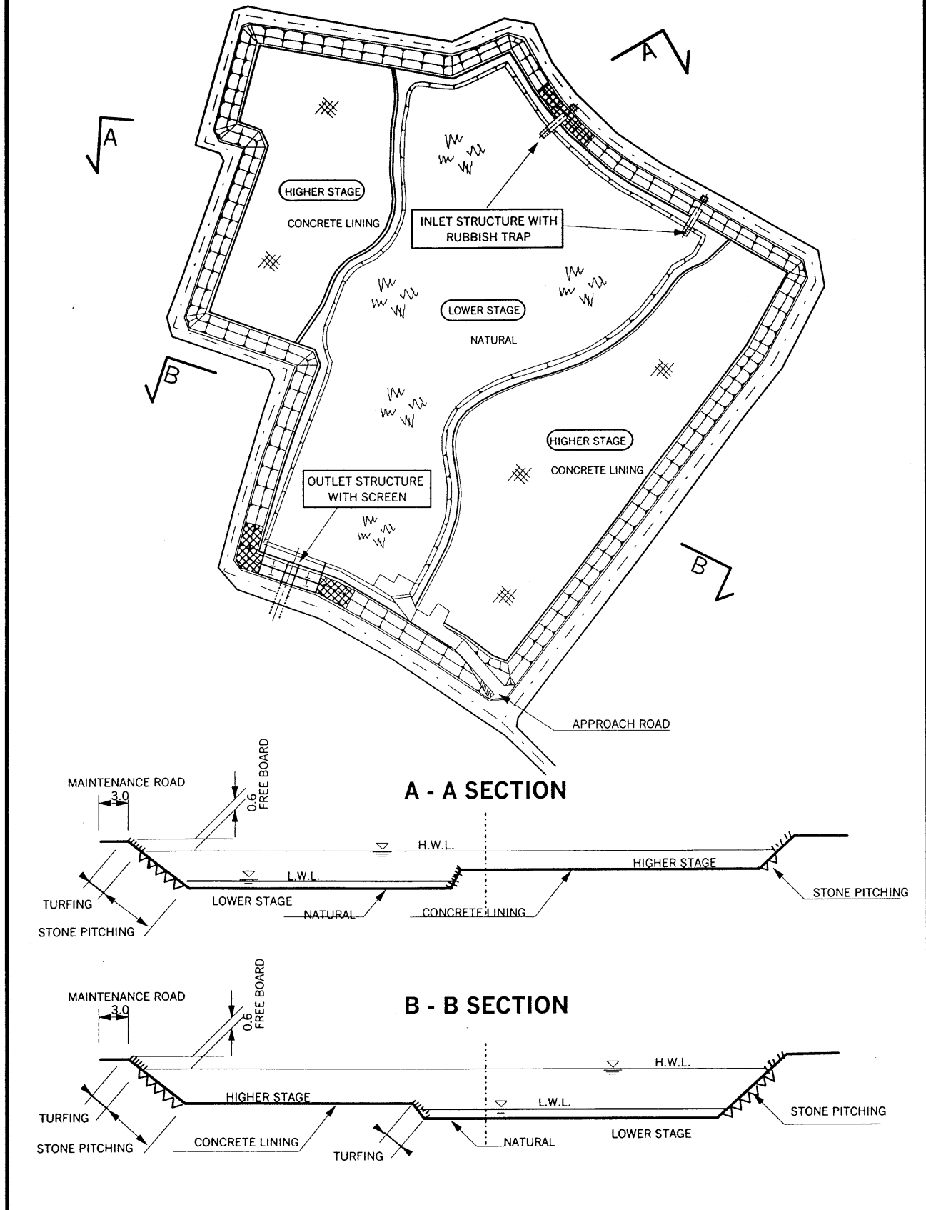
図 2-6 洪水調節池概要図
