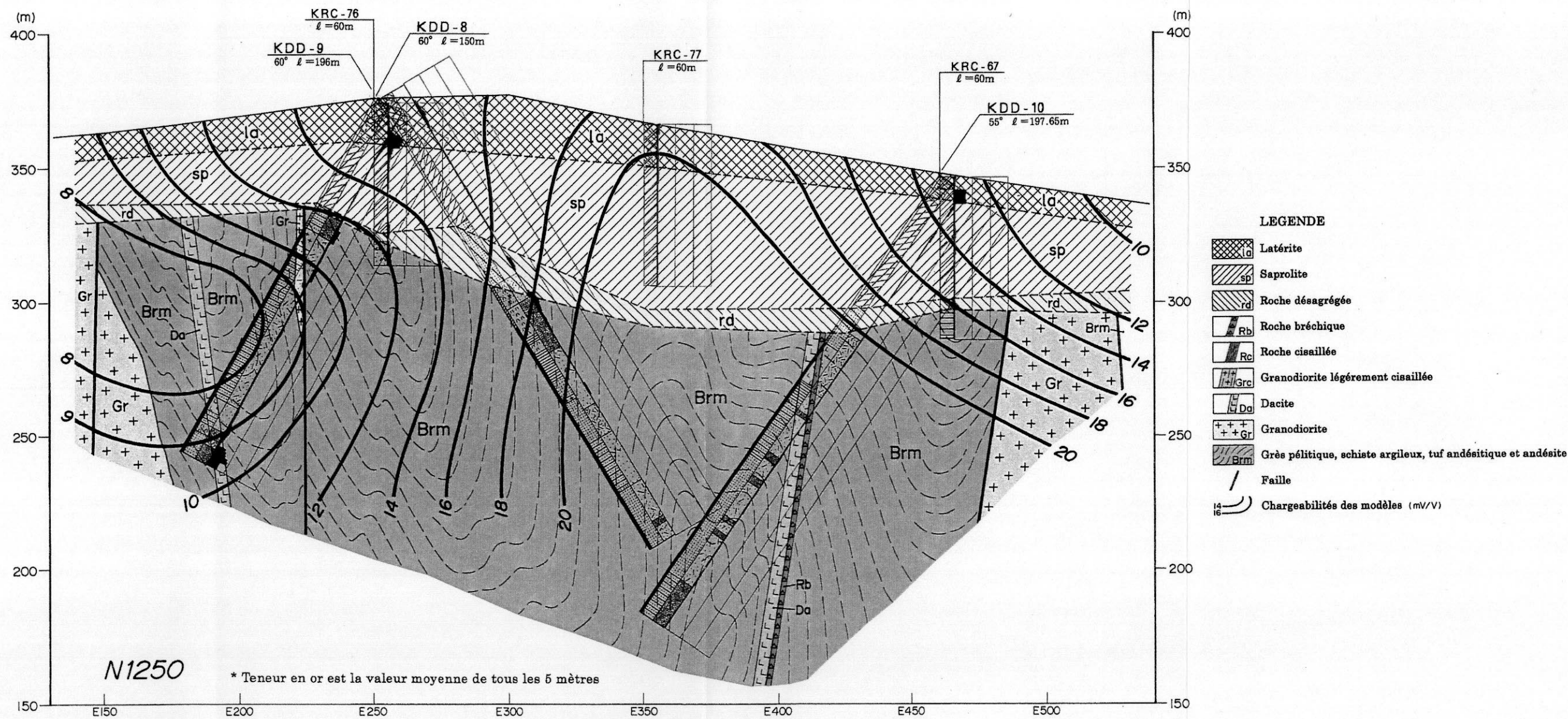
Fig.4-31 Coupe transversale à de la ligne N 1250 dans le Secteur de Kékoro
