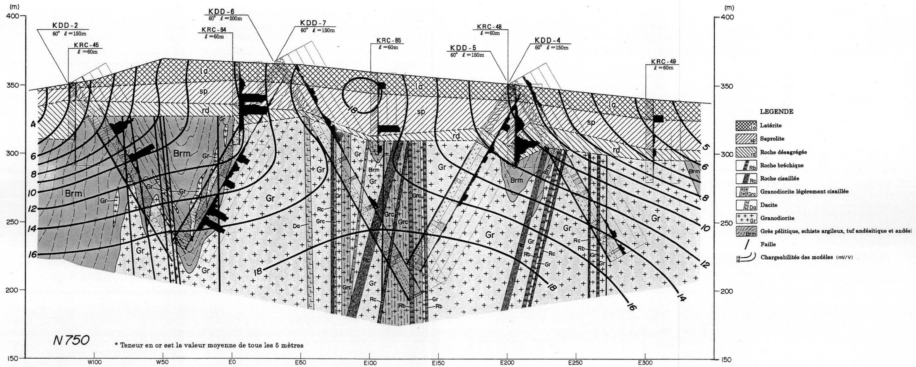
Fig.4-30 Coupe transversale à la ligne N 750 dans le Secteur de Kékoro
