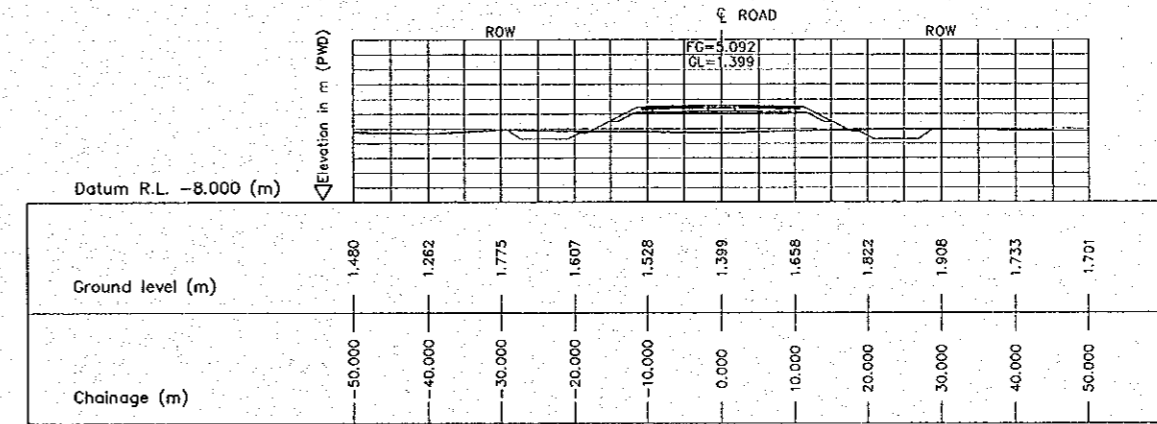
5 CROSS SECTION (STA. 6300.000) E-18 SCALE 1:500
