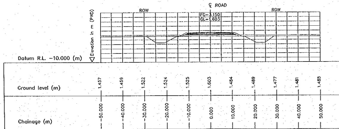
3 CROSS SECTION (STA. 3500.000) E-09 SCALE 1:500
