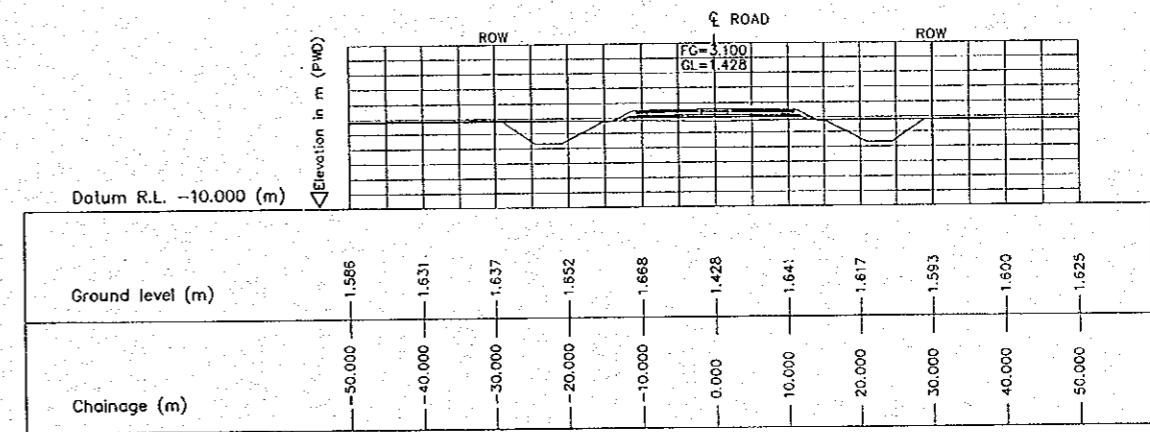
5 CROSS SECTION (STA. 1800.000) SCALE 1:500
