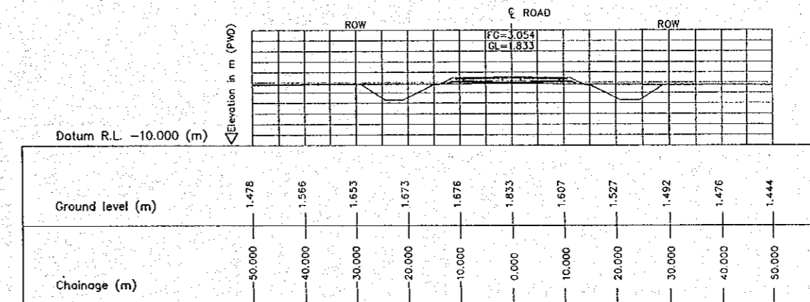
4 CROSS SECTION (STA. 3550.000) E-09 SCALE 1:500
