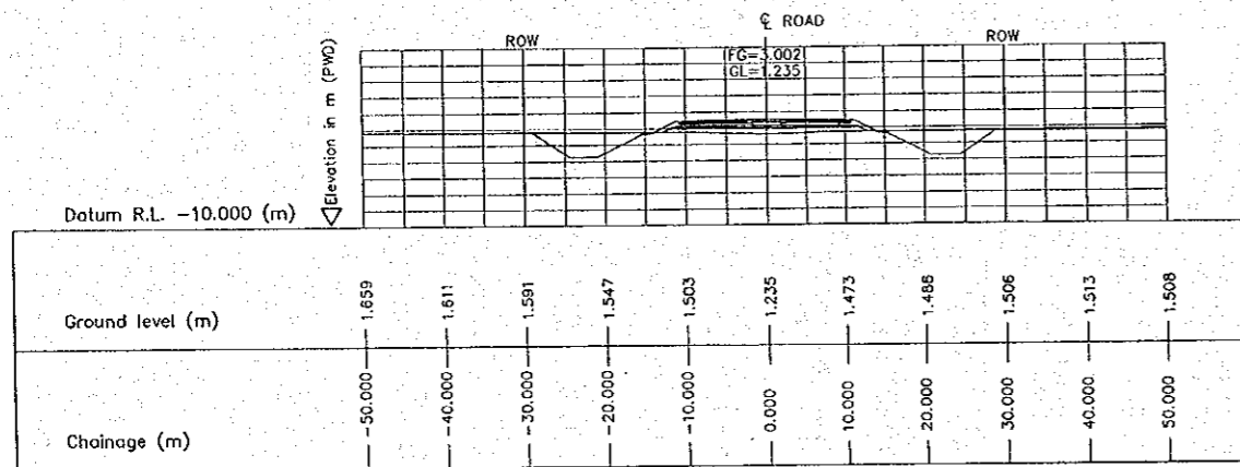
2 CROSS SECTION (STA. 1650.000) SCALE 1:500
