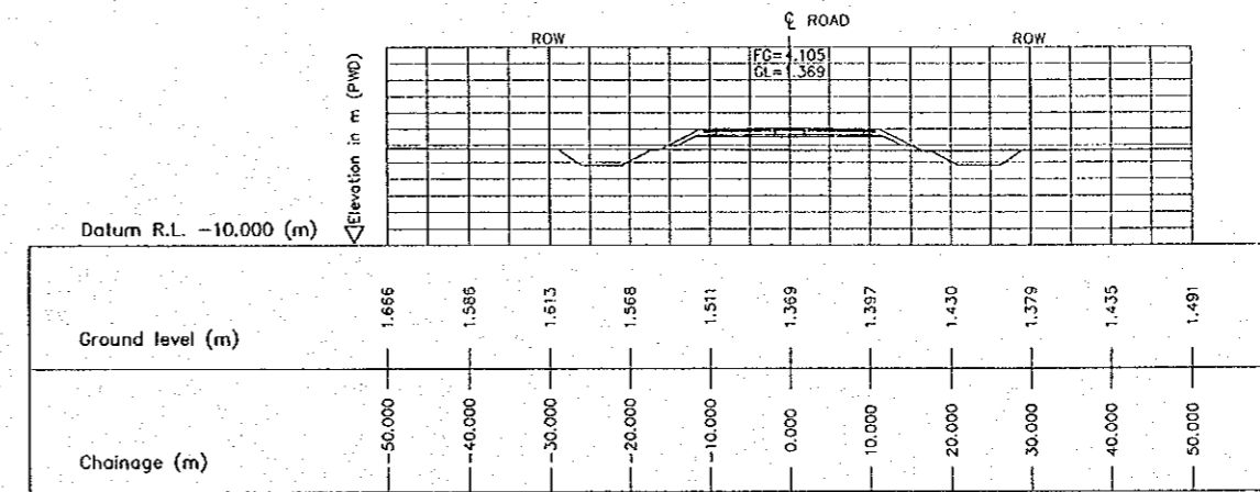
6 CROSS SECTION (STA. 5450.000) E-15 SCALE 1:500
