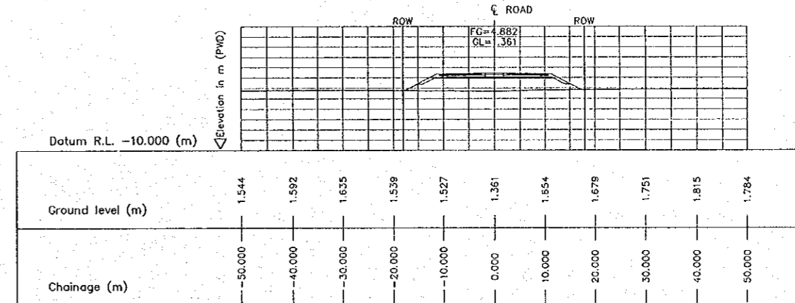
6 CROSS SECTION (STA. 6350.000) E-18 SCALE 1:500
