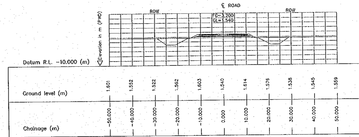
6 CROSS SECTION (STA. 1850.000) SCALE 1:500
