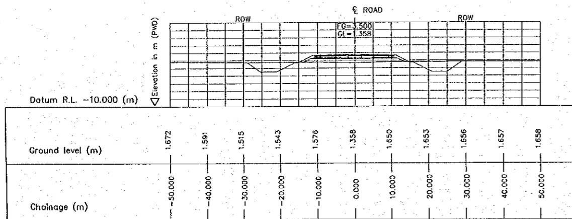
3 CROSS SECTION (STA. 2000.000) E-04 SCALE 1:500
