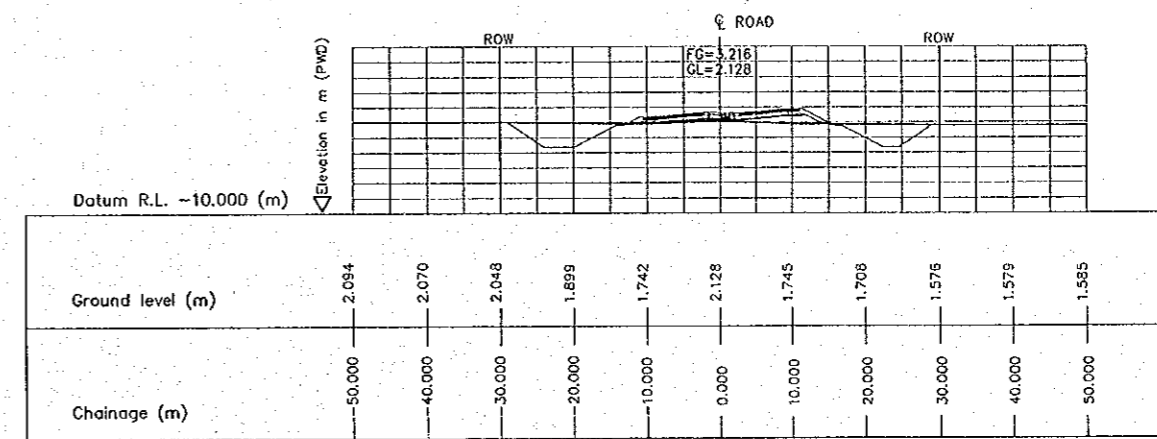
6 CROSS SECTION (STA. 2450.000) E-05 SCALE 1:500
