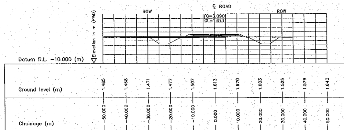
1 CROSS SECTION (STA. 4300.000) E-12 SCALE 1:500
