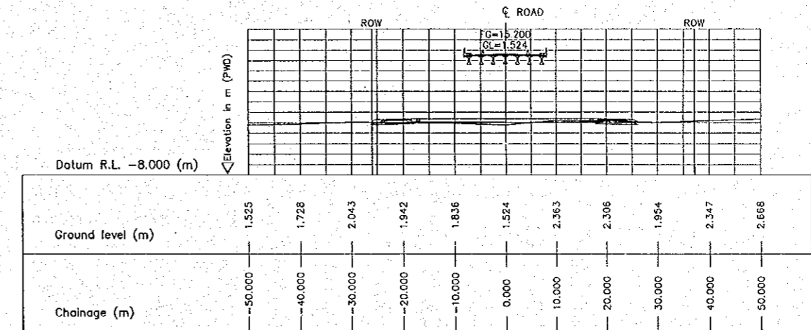
5 CROSS SECTION (STA. 7200.000) E-21 SCALE 1:500
