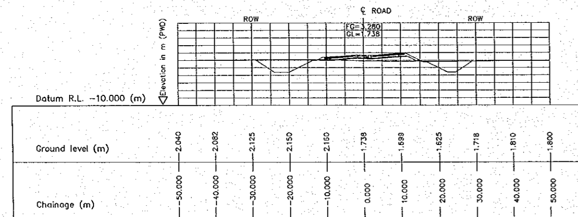
1 CROSS SECTION (STA. 2500.000) E-06 SCALE 1:500
