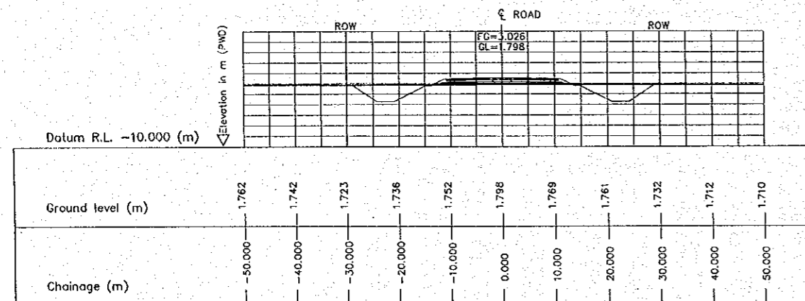
1 CROSS SECTION (STA. 3100.000) E-08 SCALE 1:500
