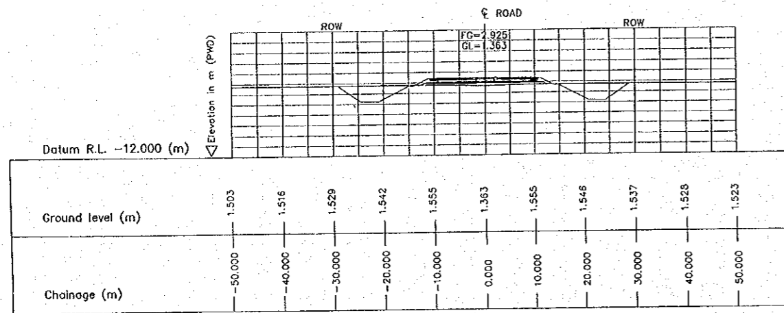
3 CROSS SECTION (STA. 1700.000) SCALE 1:500
