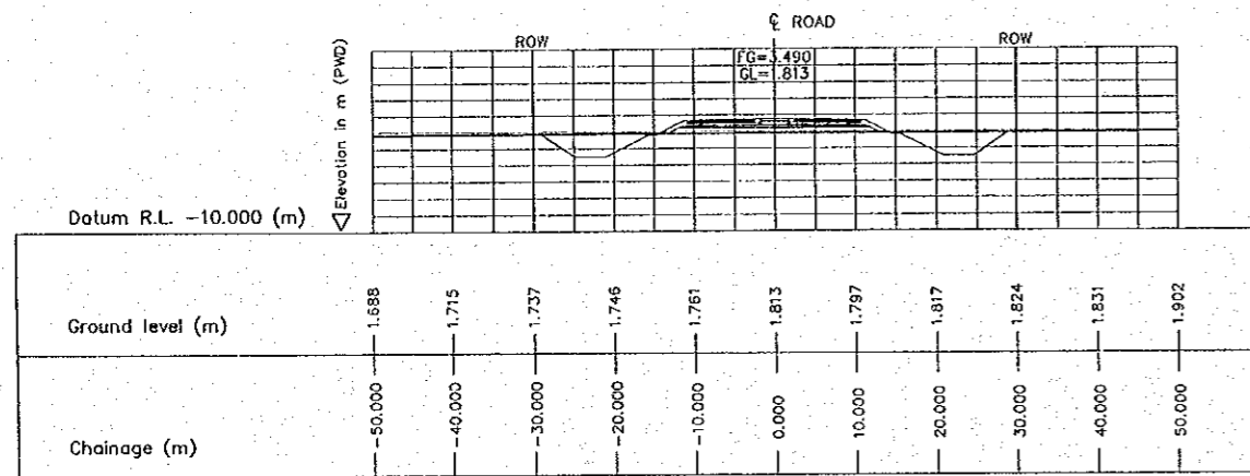
3 CROSS SECTION (STA. 3800.000) E-10 SCALE 1:500
