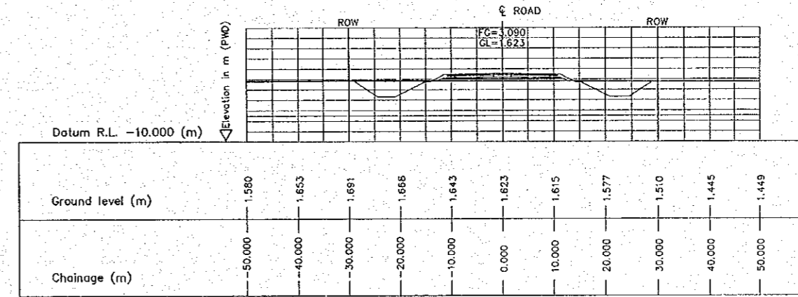
5 CROSS SECTION (STA. 3600.000) E-09 SCALE 1:500
