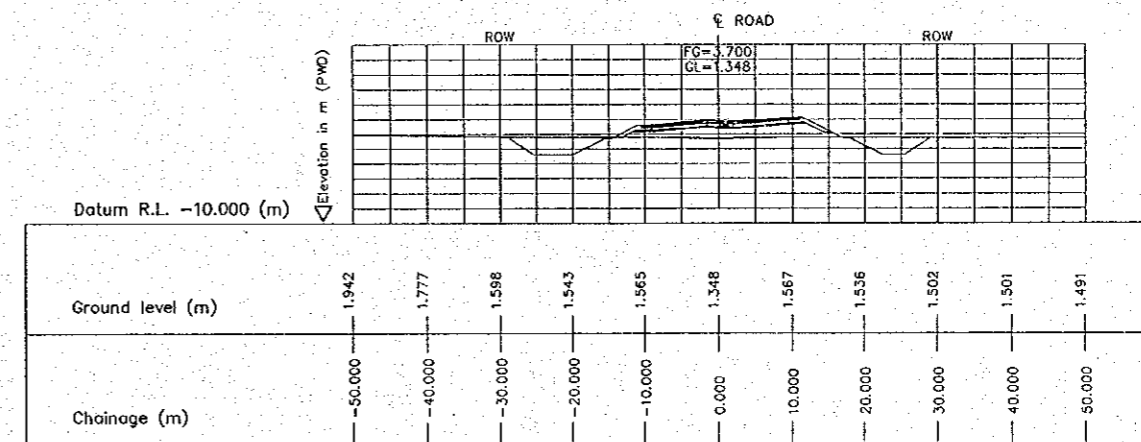
6 CROSS SECTION (STA. 2150.000) E-04 SCALE 1:500
