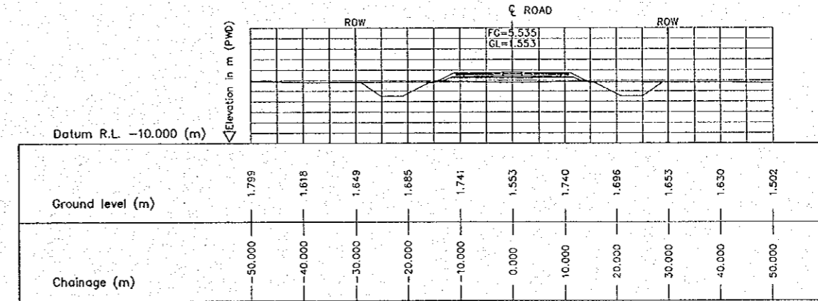
5 CROSS SECTION (STA. 6000.000) E-17 SCALE 1:500
