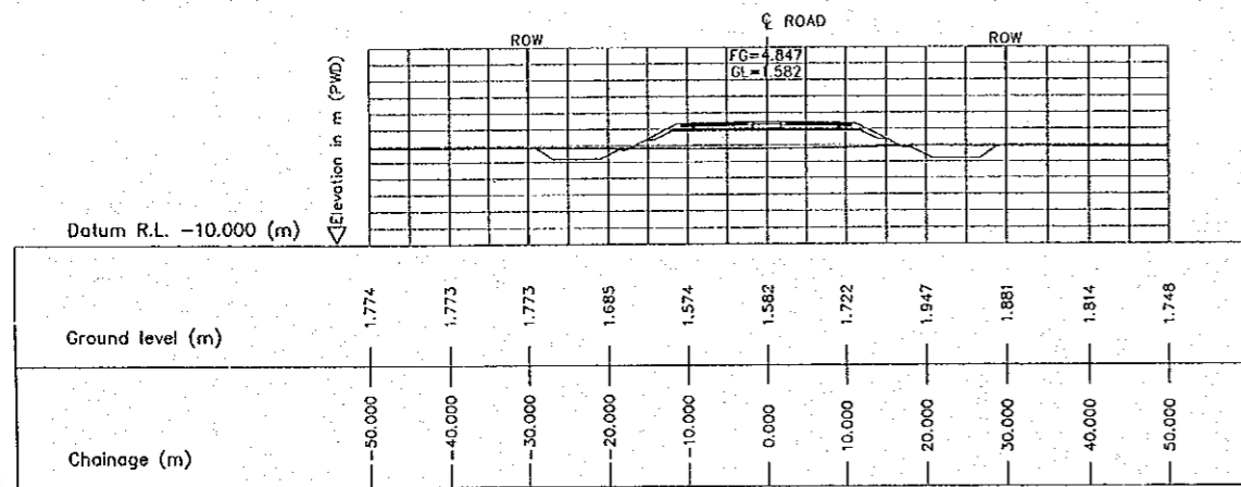
3 CROSS SECTION (STA. 5900.000) E-17 SCALE 1:500
