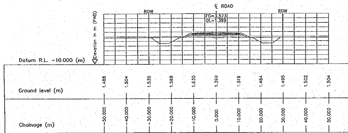
3 CROSS SECTION (STA. 5300.000) E-15 SCALE 1:500
