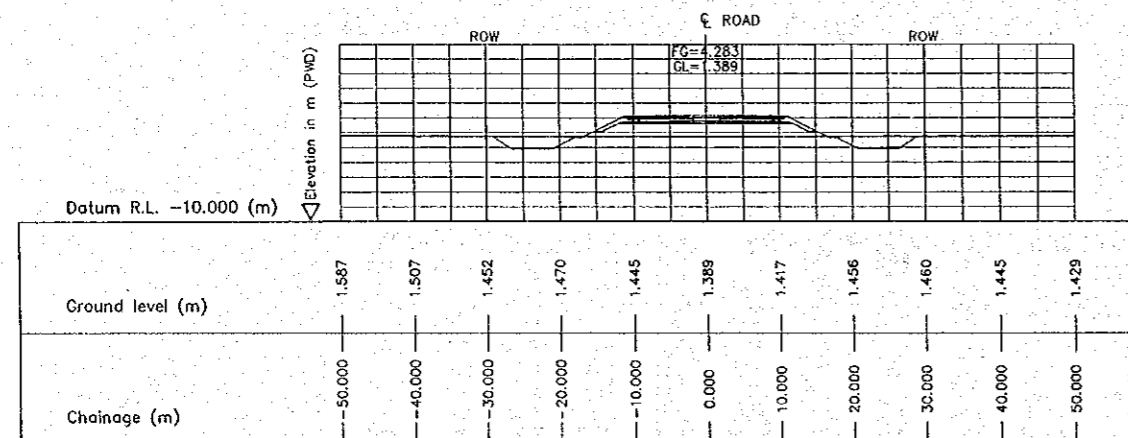
1 CROSS SECTION (STA. 5500.000) E-16 SCALE 1:500
