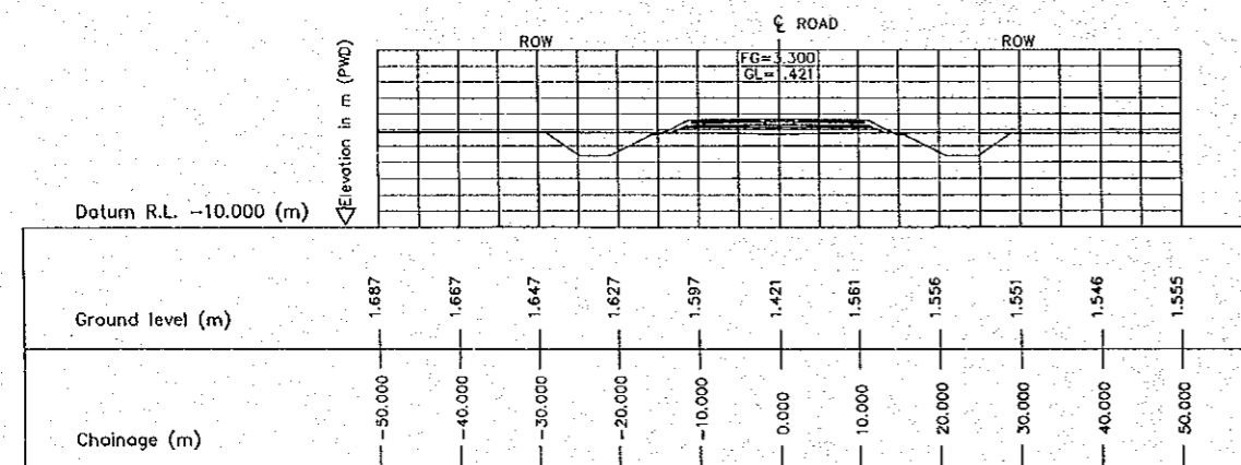
1 CROSS SECTION (STA. 1900.000) E-04 SCALE 1:500
