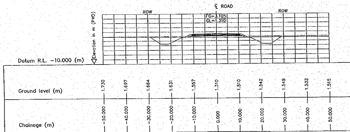
1 CROSS SECTION (STA. 1600.000) SCALE 1:500
