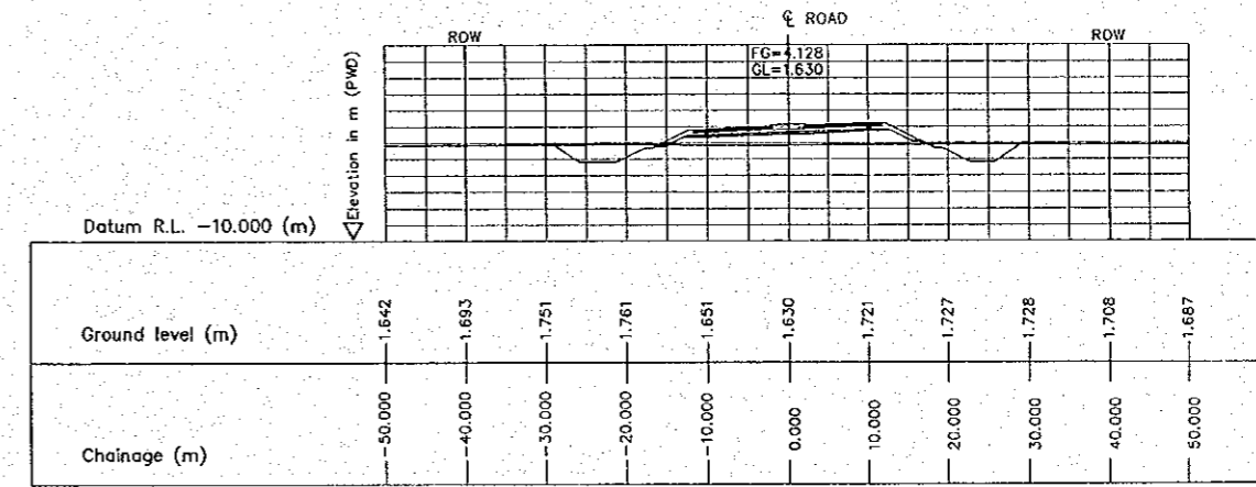
6 CROSS SECTION (STA. 2750.000) E-06 SCALE 1:500
