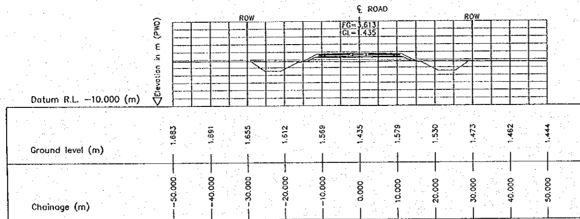
3 CROSS SECTION (STA. 5000.000) E-14 SCALE 1:500
