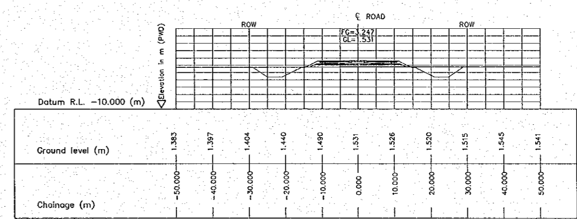
5 CROSS SECTION (STA. 1200.000) E-01 SCALE 1:1000
