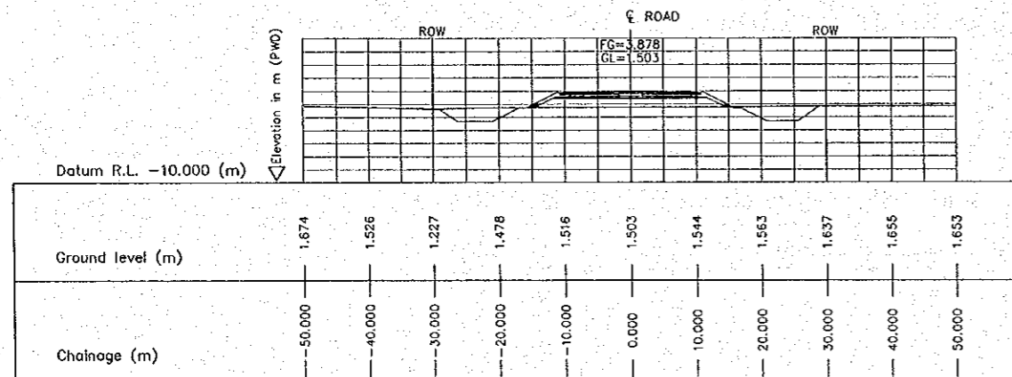
2 CROSS SECTION (STA. 6150.000) E-18 SCALE 1:500
