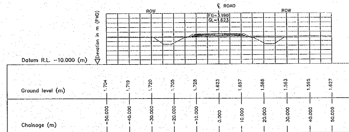
6 CROSS SECTION (STA. 3650.000) E-09 SCALE 1:500
