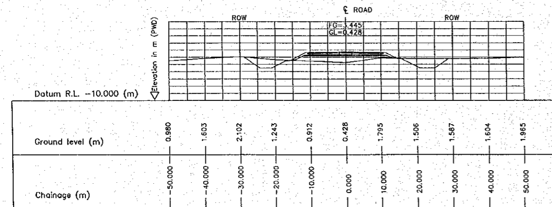
1 CROSS SECTION (STA. 1300.000) SCALE 1:1000
