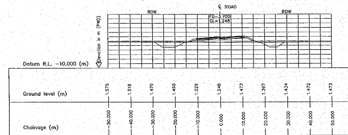
1 CROSS SECTION (STA. 2200.000) E-05 SCALE 1:500
