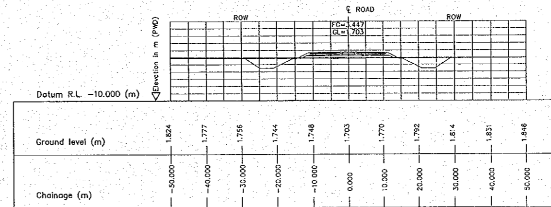
5 CROSS SECTION (STA. 3300.000) E-08 SCALE 1:500
