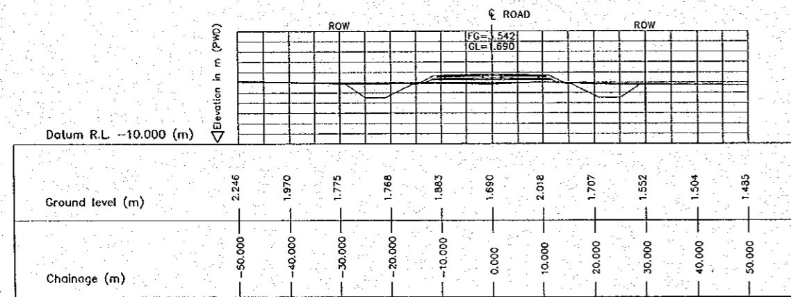
2 CROSS SECTION (STA. 1350.000) SCALE 1:1000
