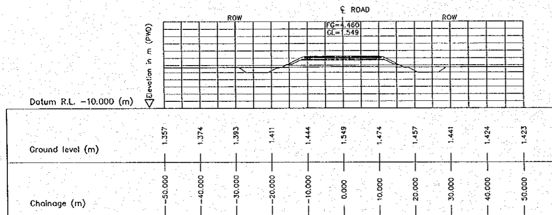
2 CROSS SECTION (STA. 5550.000) E-16 SCALE 1:500
