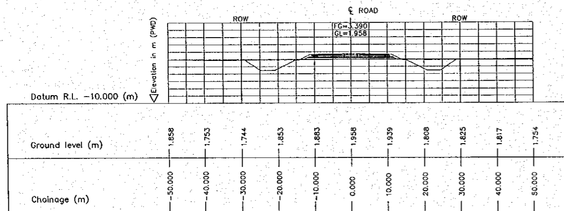
2 CROSS SECTION (STA. 3750.000) E-10 SCALE 1:500
