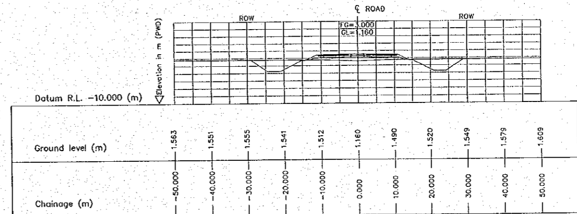
4 CROSS SECTION (STA. 1750.000) SCALE 1:500
