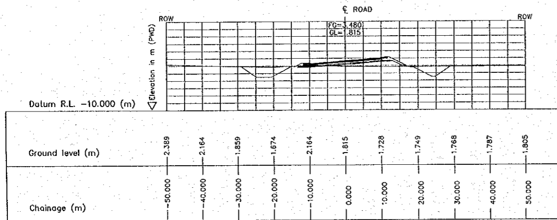
3 CROSS SECTION (STA. 2600.000) E-06 SCALE 1:500
