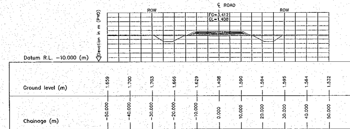
4 CROSS SECTION (STA. 1450.000) SCALE 1:1000
