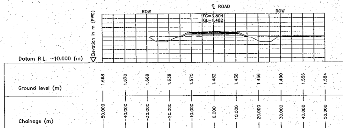
2 CROSS SECTION (STA. 4950.000) E-14 SCALE 1:500
