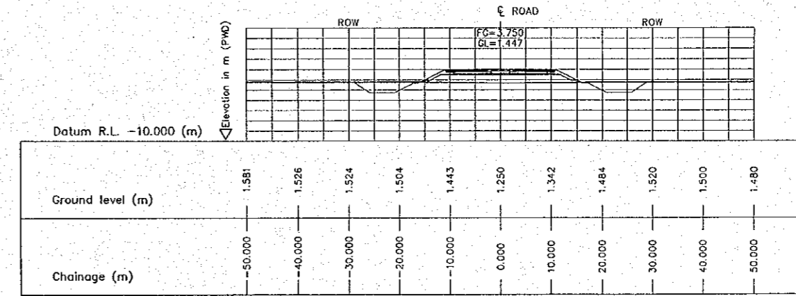
5 CROSS SECTION (STA. 5400.000) E-15 SCALE 1:500
