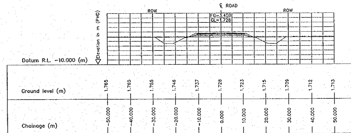
6 CROSS SECTION (STA. 3350.000) E-08 SCALE 1:500
