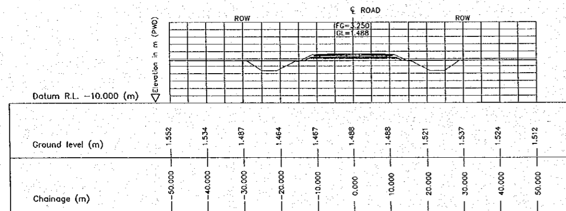
2 CROSS SECTION (STA. 3450.000) E-09 SCALE 1:500
