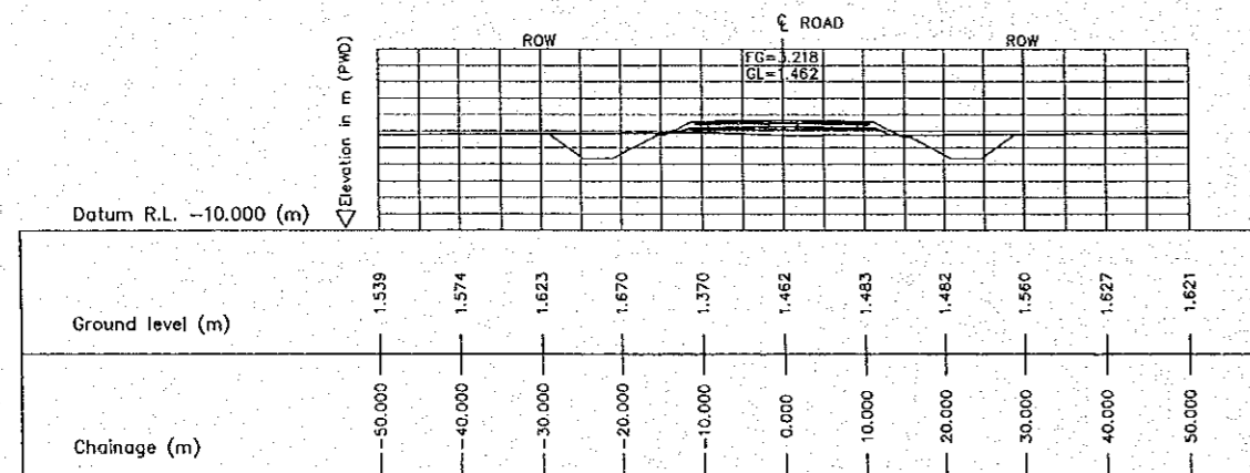
1 CROSS SECTION (STA. 5200.000) E-15 SCALE 1:500
