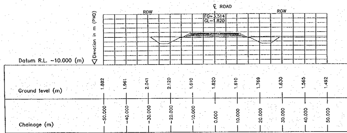
3 CROSS SECTION (STA. 1400.000) SCALE 1:1000
