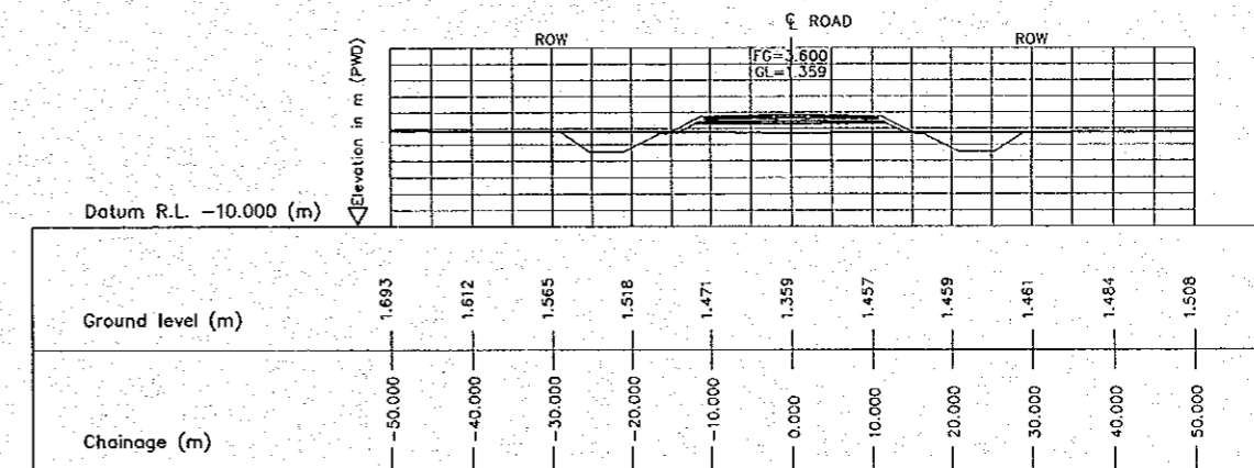
4 CROSS SECTION (STA. 2050.000) E-04 SCALE 1:500
