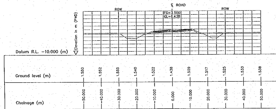
3 CROSS SECTION (STA. 2300.000) E-05 SCALE 1:500
