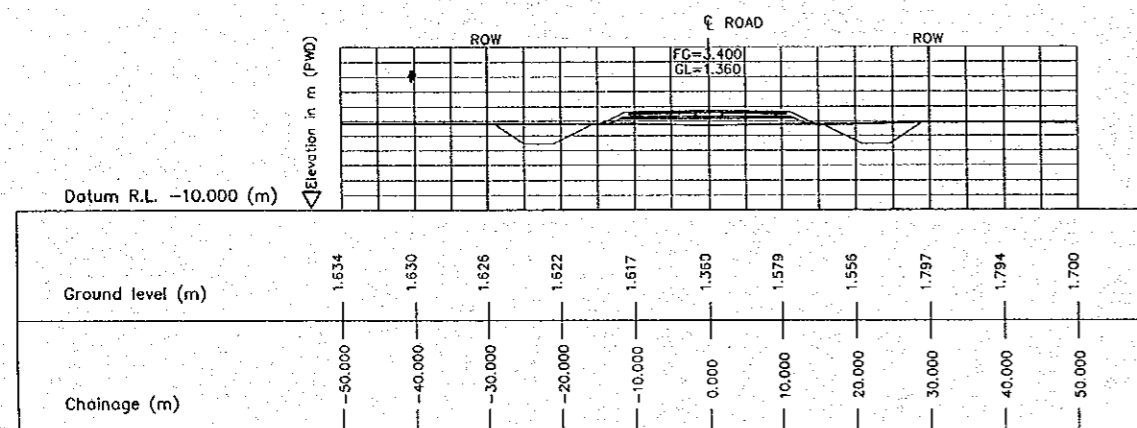
2 CROSS SECTION (STA. 1950.000) E-04 SCALE 1:500
