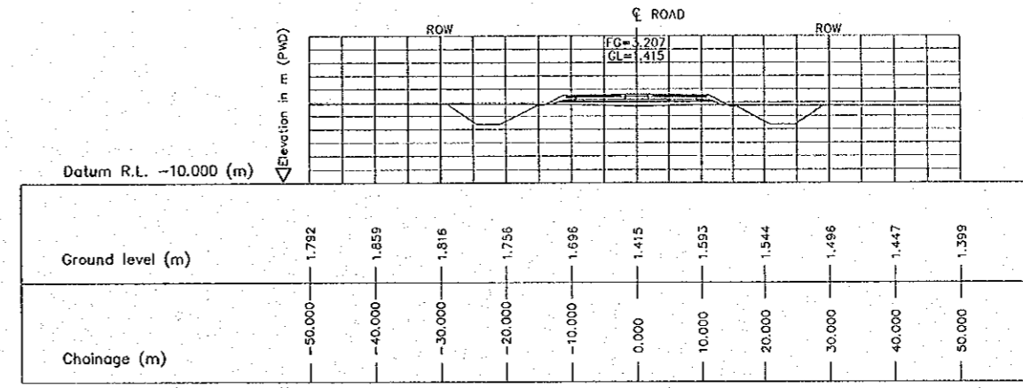
6 CROSS SECTION (STA. 1550.000) SCALE 1:1000
