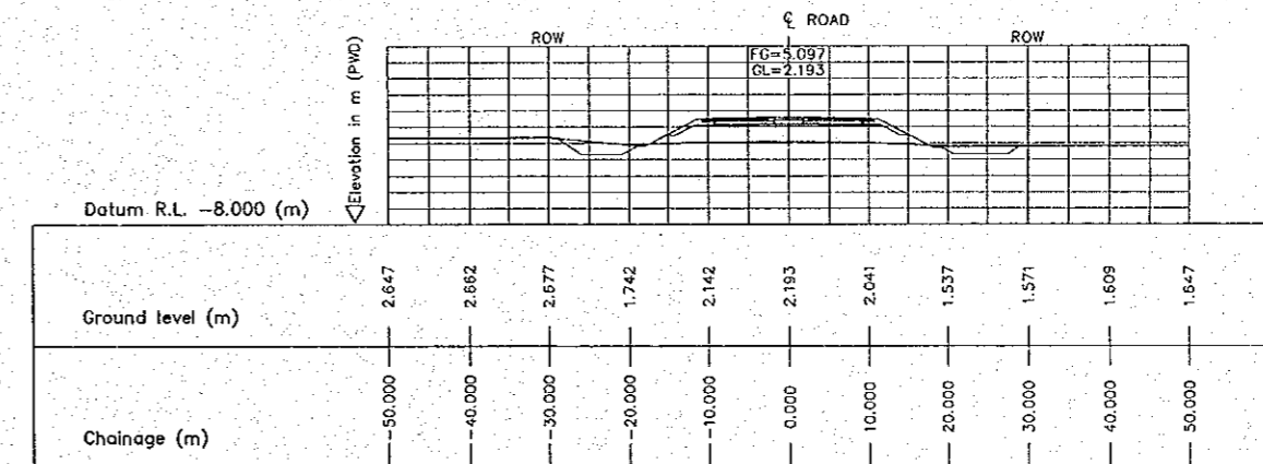
4 CROSS SECTION (STA. 6250.000) E-18 SCALE 1:500
