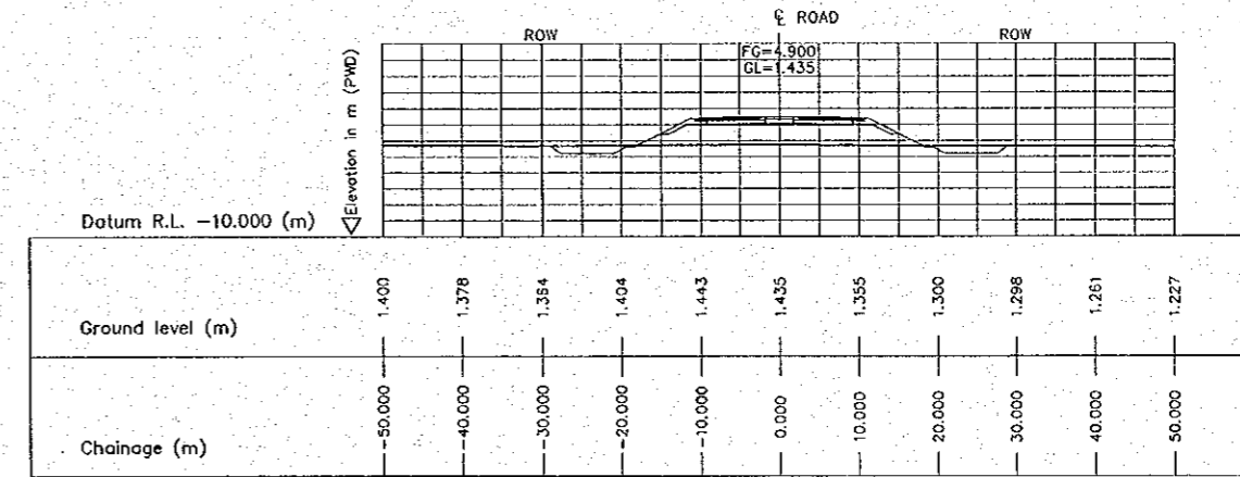
5 CROSS SECTION (STA. 5700.000) E-16 SCALE 1:500
