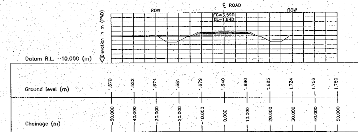
4 CROSS SECTION (STA. 3850.000) E-10 SCALE 1:500
