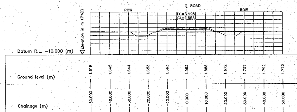
1 CROSS SECTION (STA. 4900.000) E-14 SCALE 1:500
