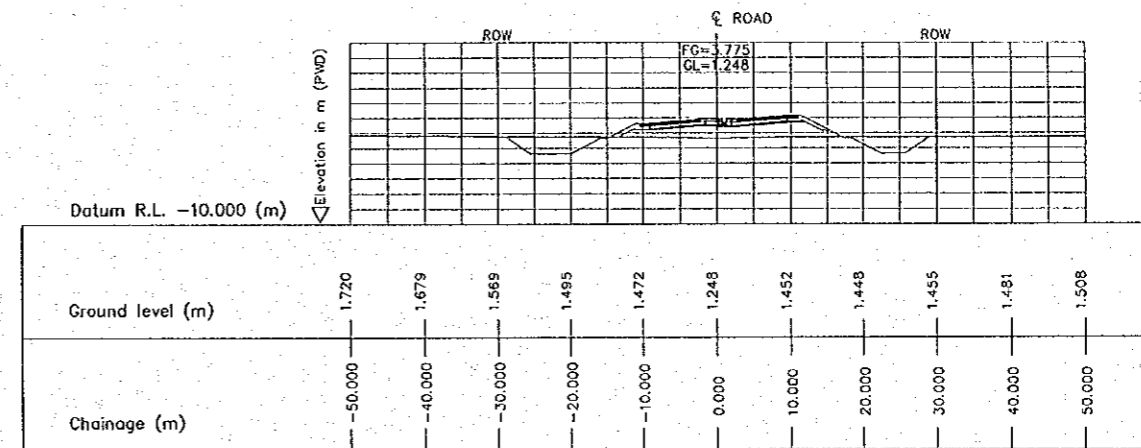
6 CROSS SECTION (STA. 2150.000) E-04 SCALE 1:500
