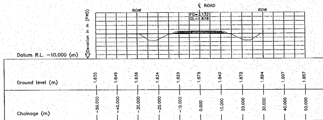
2 CROSS SECTION (STA. 3150.000) E-08 SCALE 1:500
