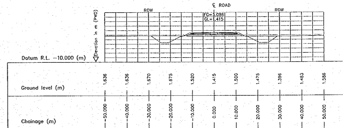
6 CROSS SECTION (STA. 5150.000) E-14 SCALE 1:500
