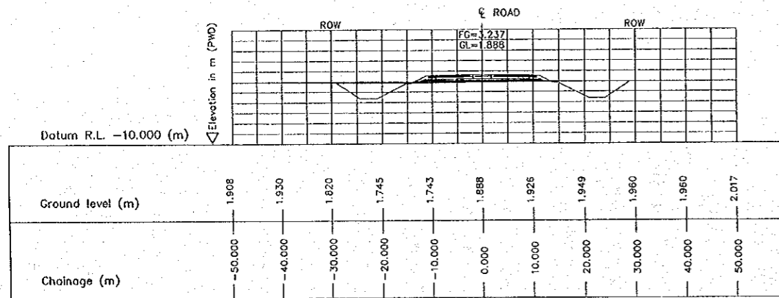
3 CROSS SECTION (STA. 3200.000) E-08 SCALE 1:500
