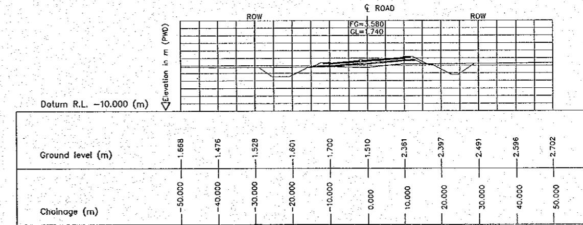
4 CROSS SECTION (STA. 2650.000) E-06 SCALE 1:500
