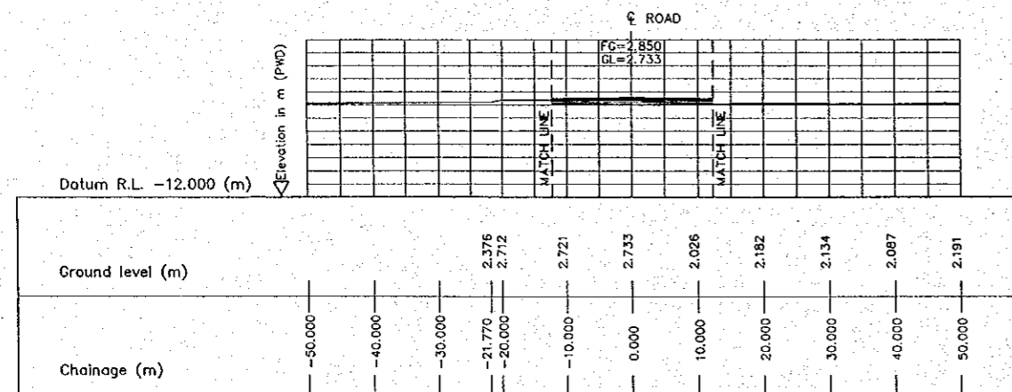
1 CROSS SECTION (STA. 1000.000) E-01 SCALE 1:1000
