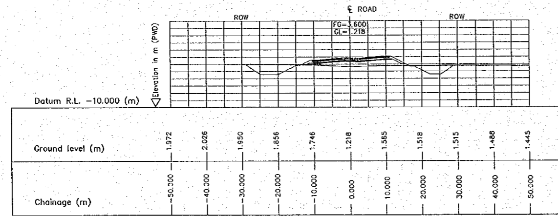
2 CROSS SECTION (STA. 2250.000) E-05 SCALE 1:500
