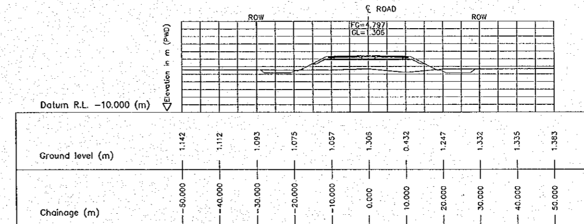
4 CROSS SECTION (STA. 5650.000) E-16 SCALE 1:500
