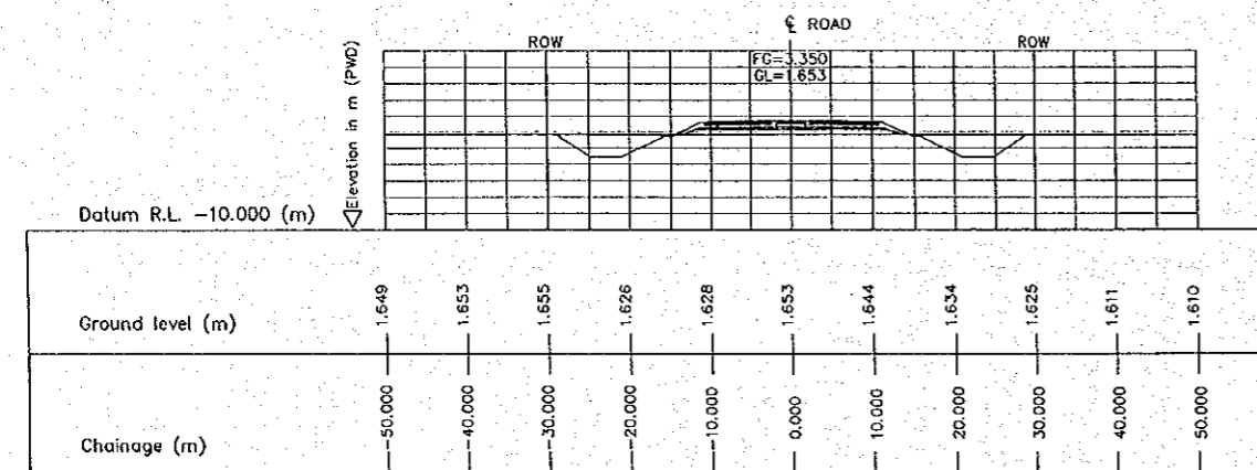
1 CROSS SECTION (STA. 3400.000) E-09 SCALE 1:500
