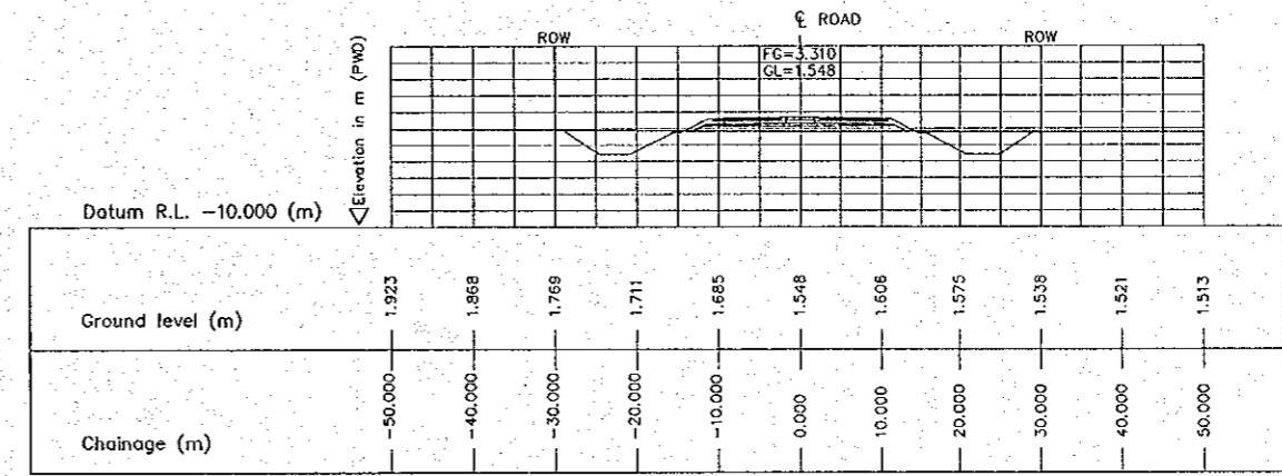
5 CROSS SECTION (STA. 1500.000) SCALE 1:1000
