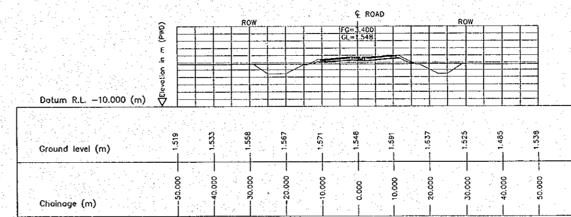
4 CROSS SECTION (STA. 2350.000) E-05 SCALE 1:500
