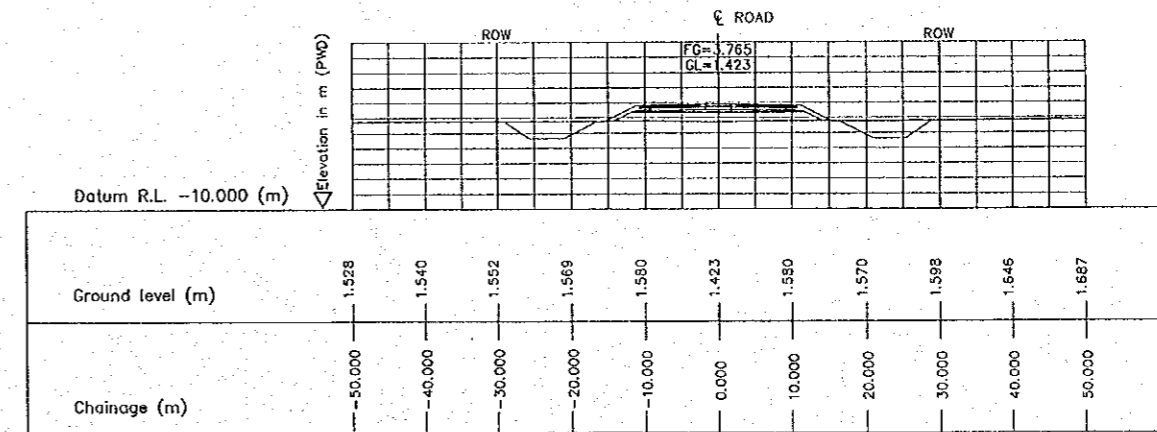
6 CROSS SECTION (STA. 3950.000) E-10 SCALE 1:500
