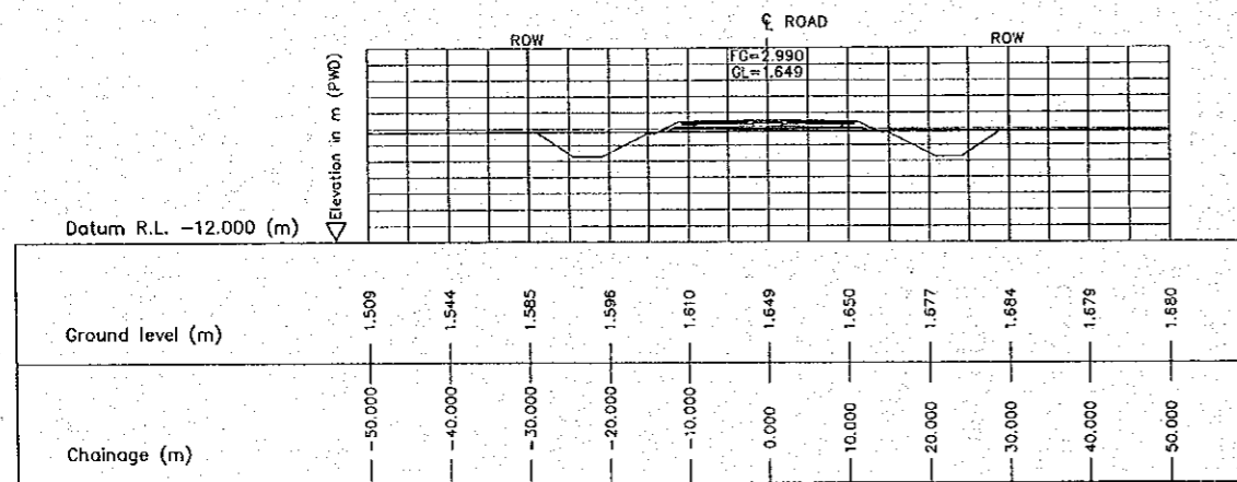
3 CROSS SECTION (STA. 4400.000) E-12 SCALE 1:500
