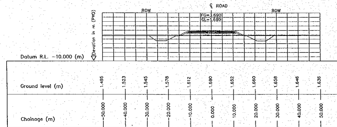
1 CROSS SECTION (STA. 4000.000) E-11 SCALE 1:500
