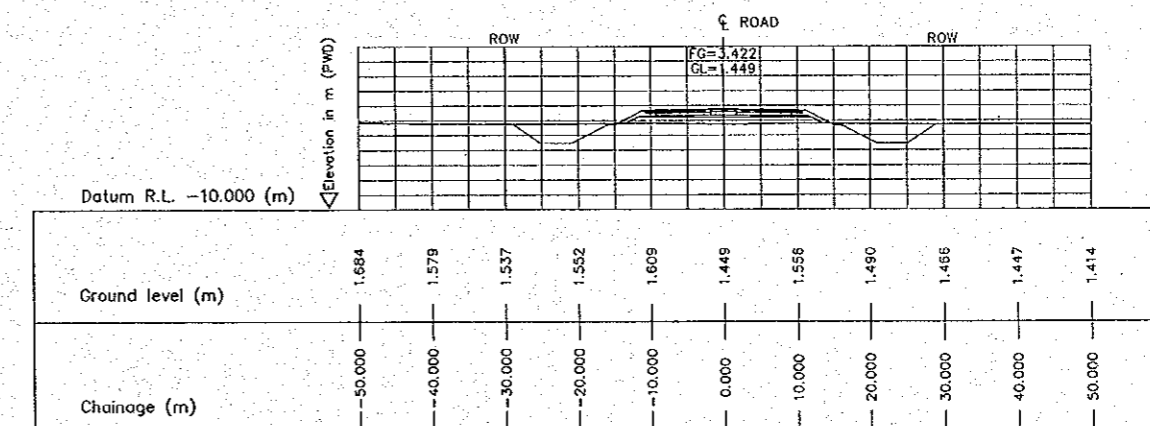
4 CROSS SECTION (STA. 5050.000) E-14 SCALE 1:500
