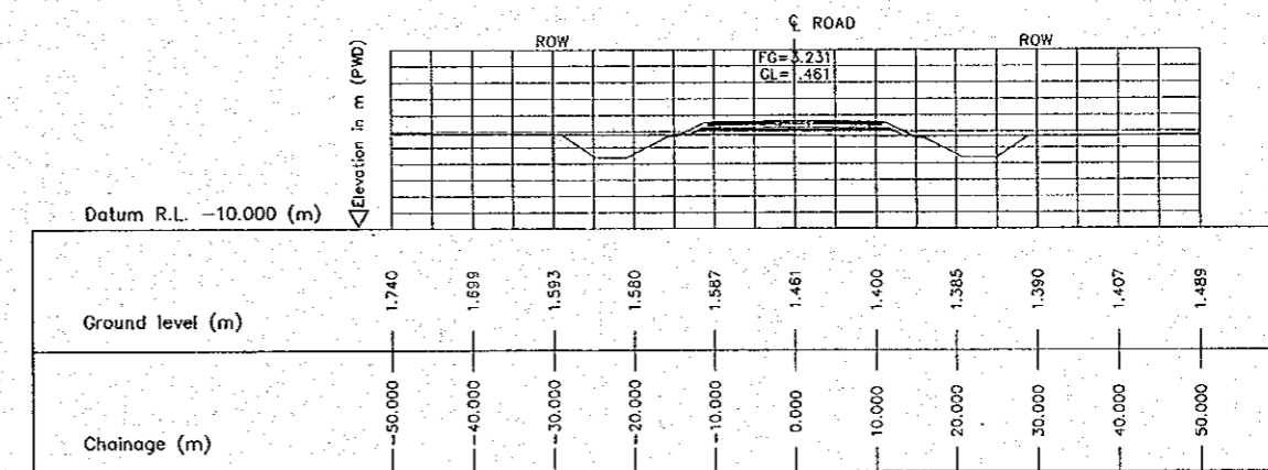
5 CROSS SECTION (STA. 5100.000) E-14 SCALE 1:500
