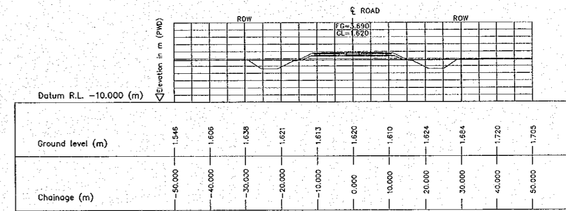
5 CROSS SECTION (STA. 3900.000) E-10 SCALE 1:500
