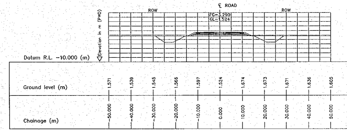
5 CROSS SECTION (STA. 4200.000) E-11 SCALE 1:500
