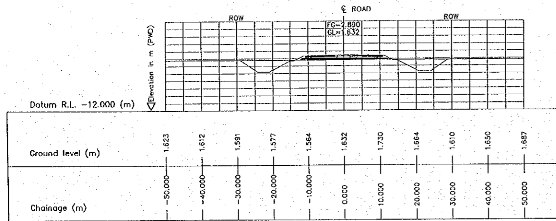
3 CROSS SECTION (STA. 4400.000) E-12 SCALE 1:500
