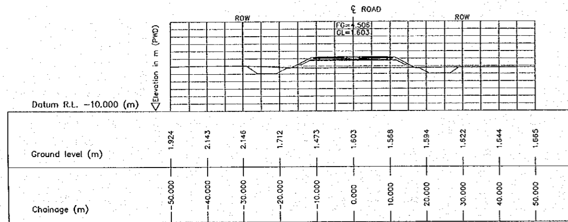
3 CROSS SECTION (STA. 6200.000) E-18 SCALE 1:500
