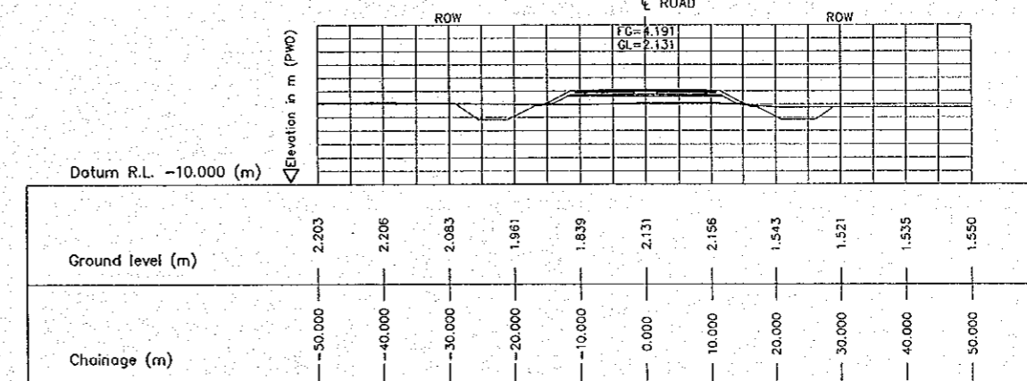
4 CROSS SECTION (STA. 5950.000) E-17 SCALE 1:500
