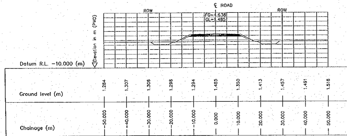
3 CROSS SECTION (STA. 5600.000) E-16 SCALE 1:500
