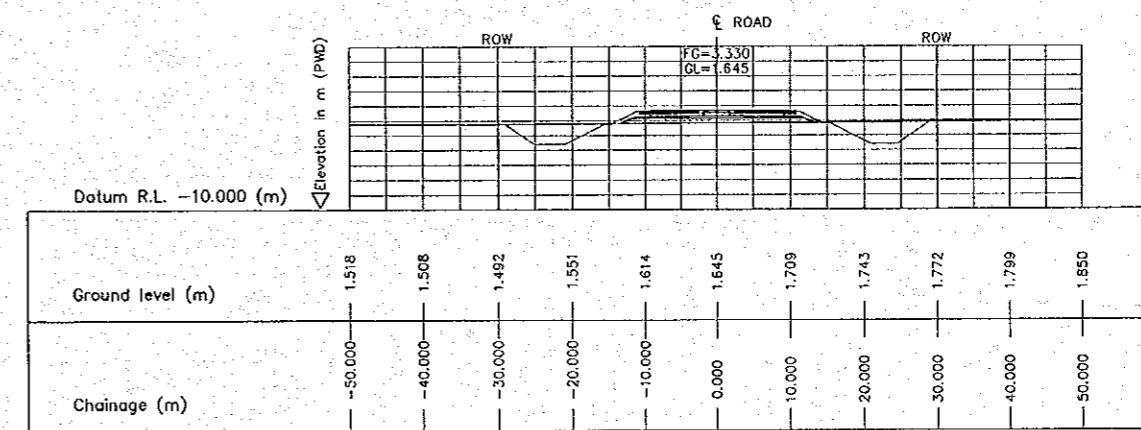
5 CROSS SECTION (STA. 4500.000) E-12 SCALE 1:500
