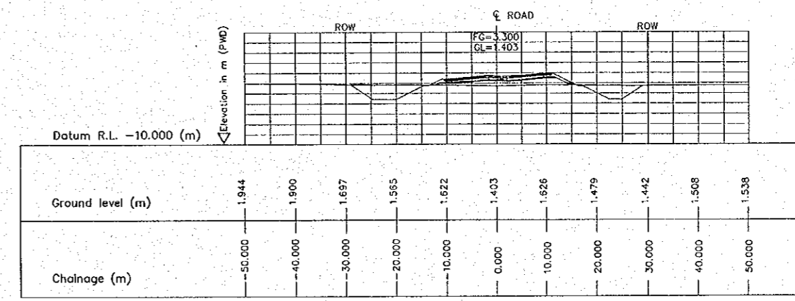
5 CROSS SECTION (STA. 2400.000) E-05 SCALE 1:500
