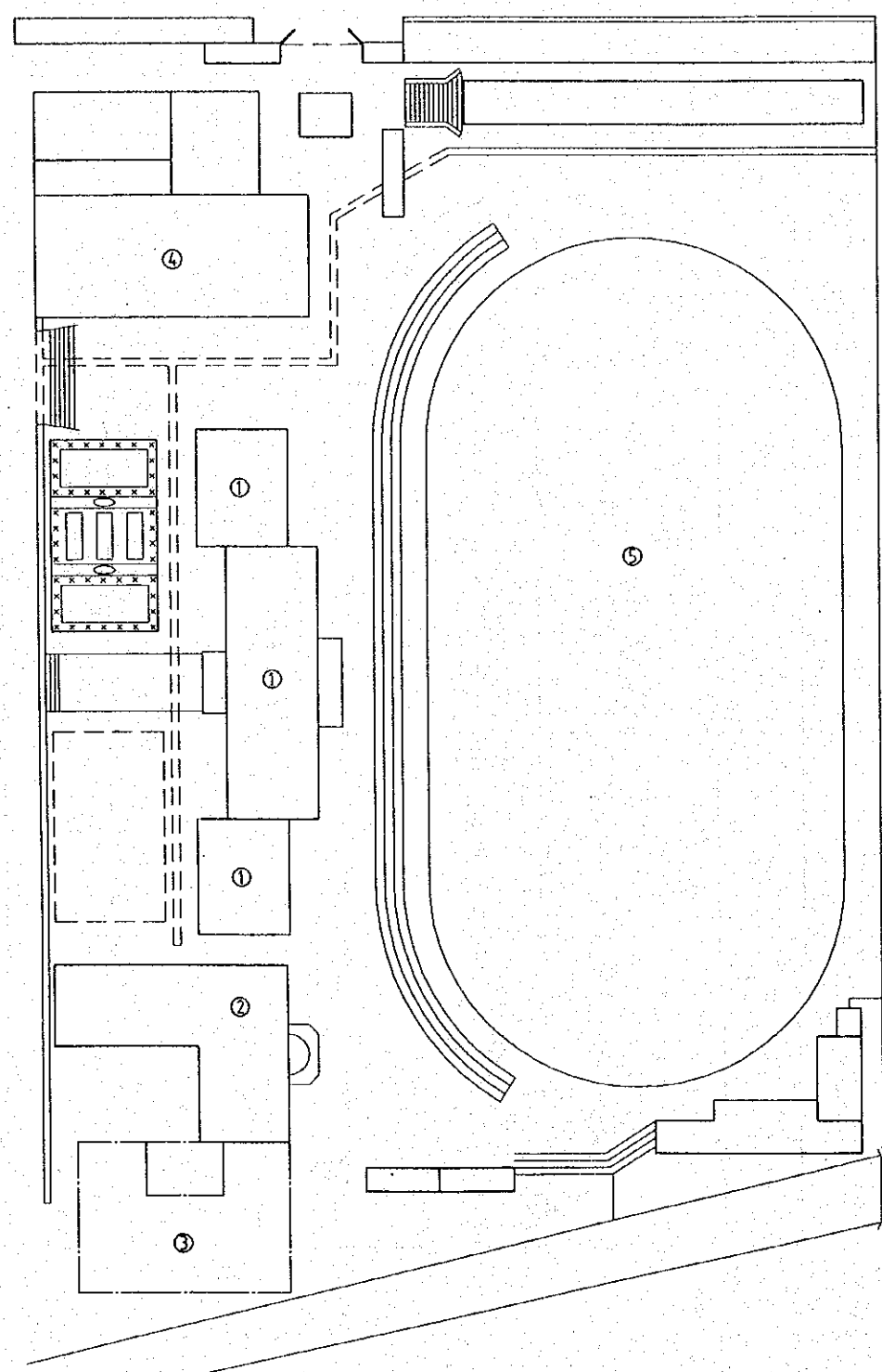
困場満族モンゴル族自治区民族中学（高級中学）全体配置図
