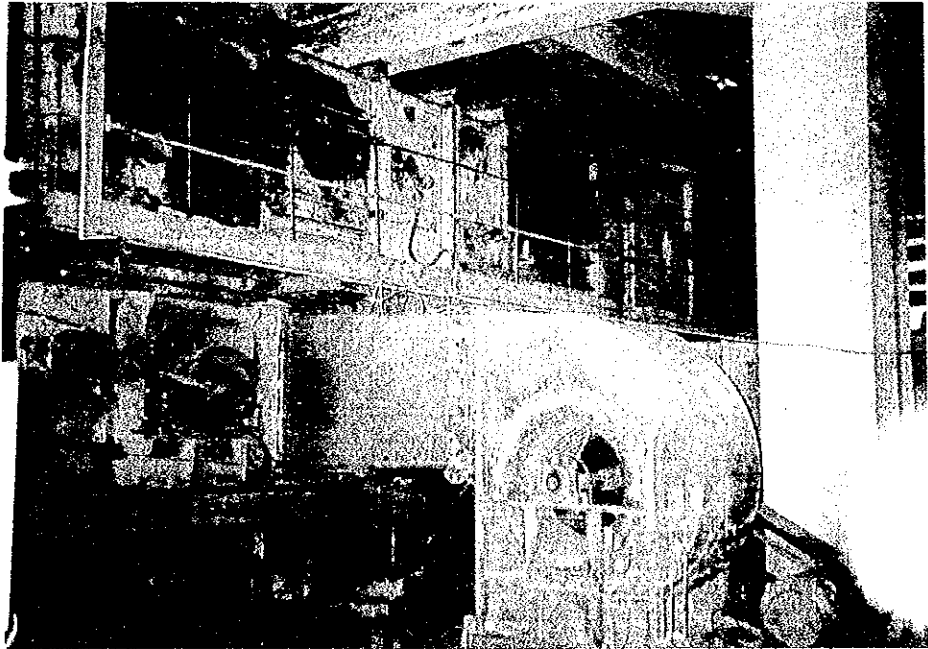
(写真-20) No.4, 5 クリカケーラ(グレート式)
