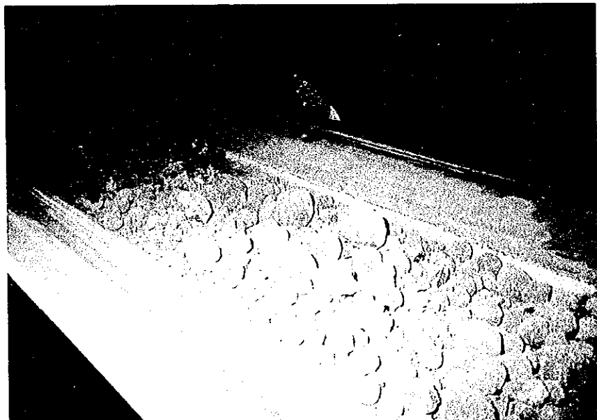
(写真-2 2) クリンカ送り ベルトコンベヤ (No.4, 5キルン)
