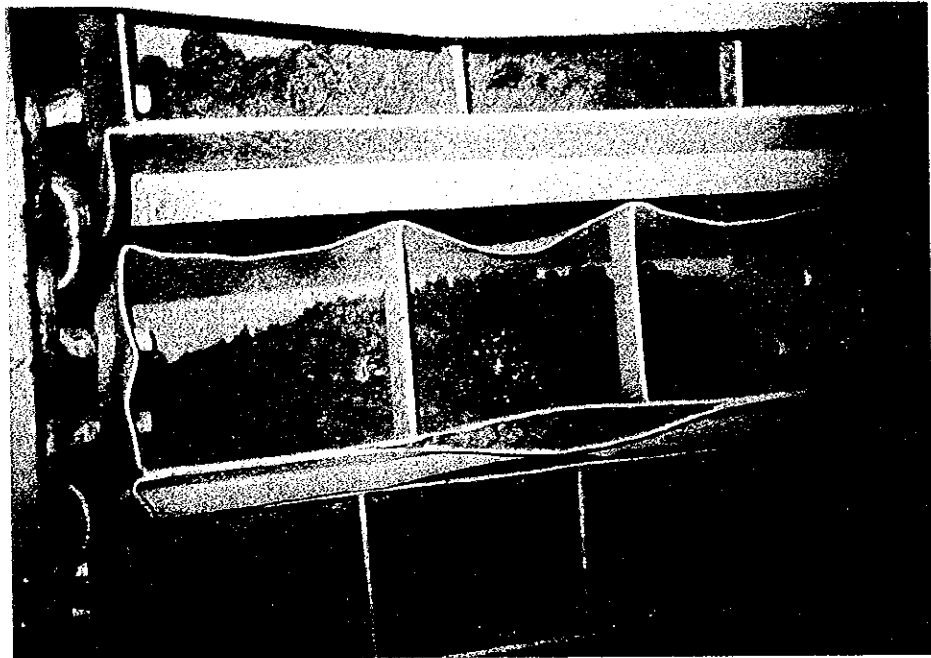
(写真-2 1) クリンカ送り バケットコンベヤ (No.1~3キルン) 粒度が大きく赤い塊がある
