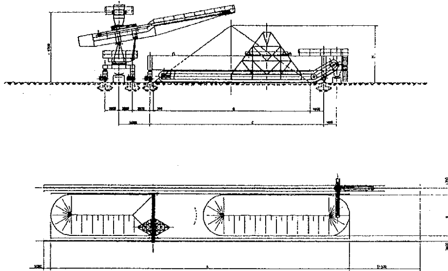
図 7.1.2 スタッカ/リクレーマ(石灰石)
