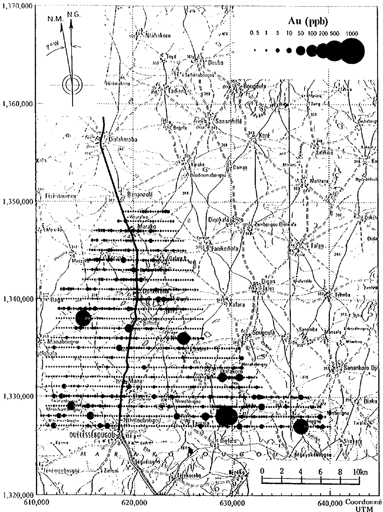
Apc.7-1 Résultat d'analyse géochimique (Au, Secteur Ouest)
