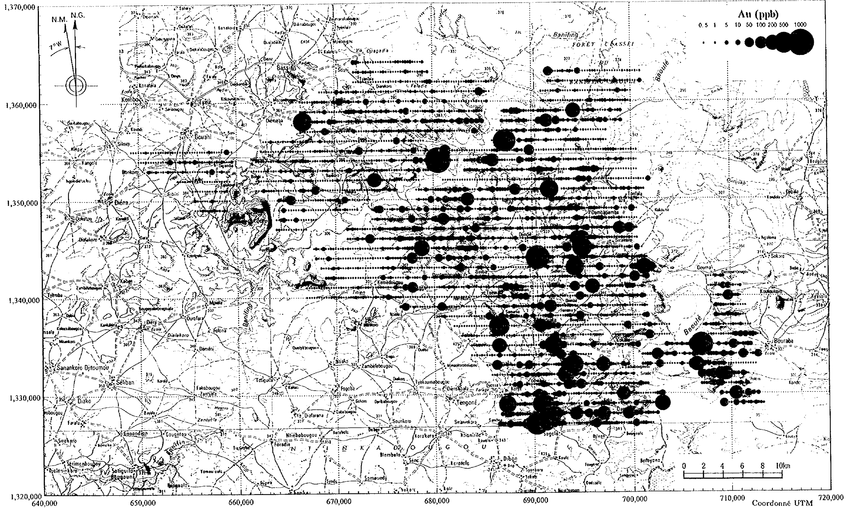
Apc.6-1 Résultat d'analyse géochimique (Au, Secteur Est)
