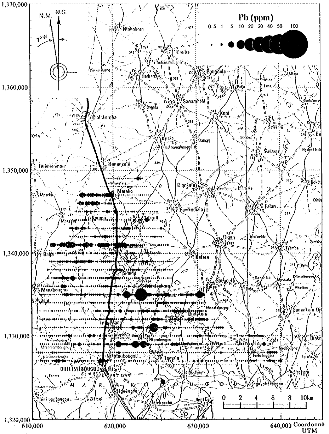
Apc.7-4 Résultat d'analyse géochimique (Pb, Secteur Ouest)
