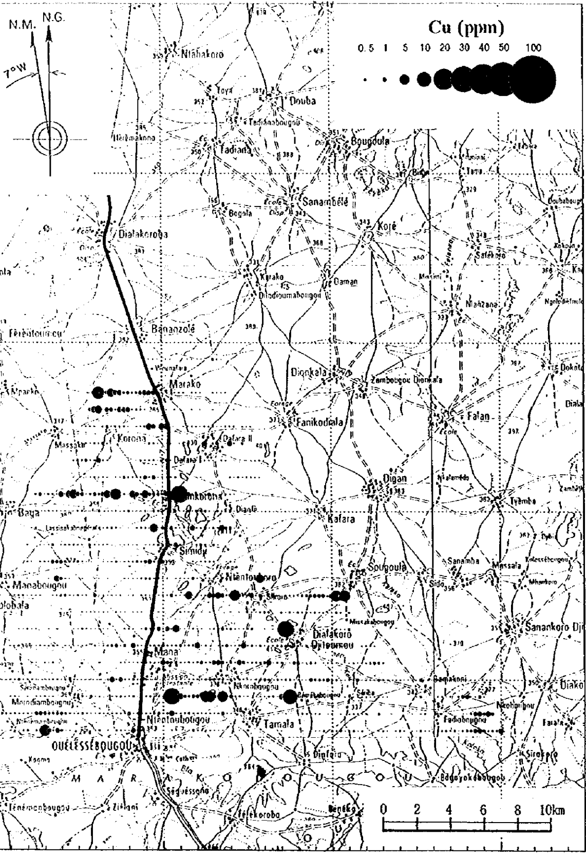
Apc.7-3 Résultat d'analyse géochimique (Cu, Secteur Ouest)
