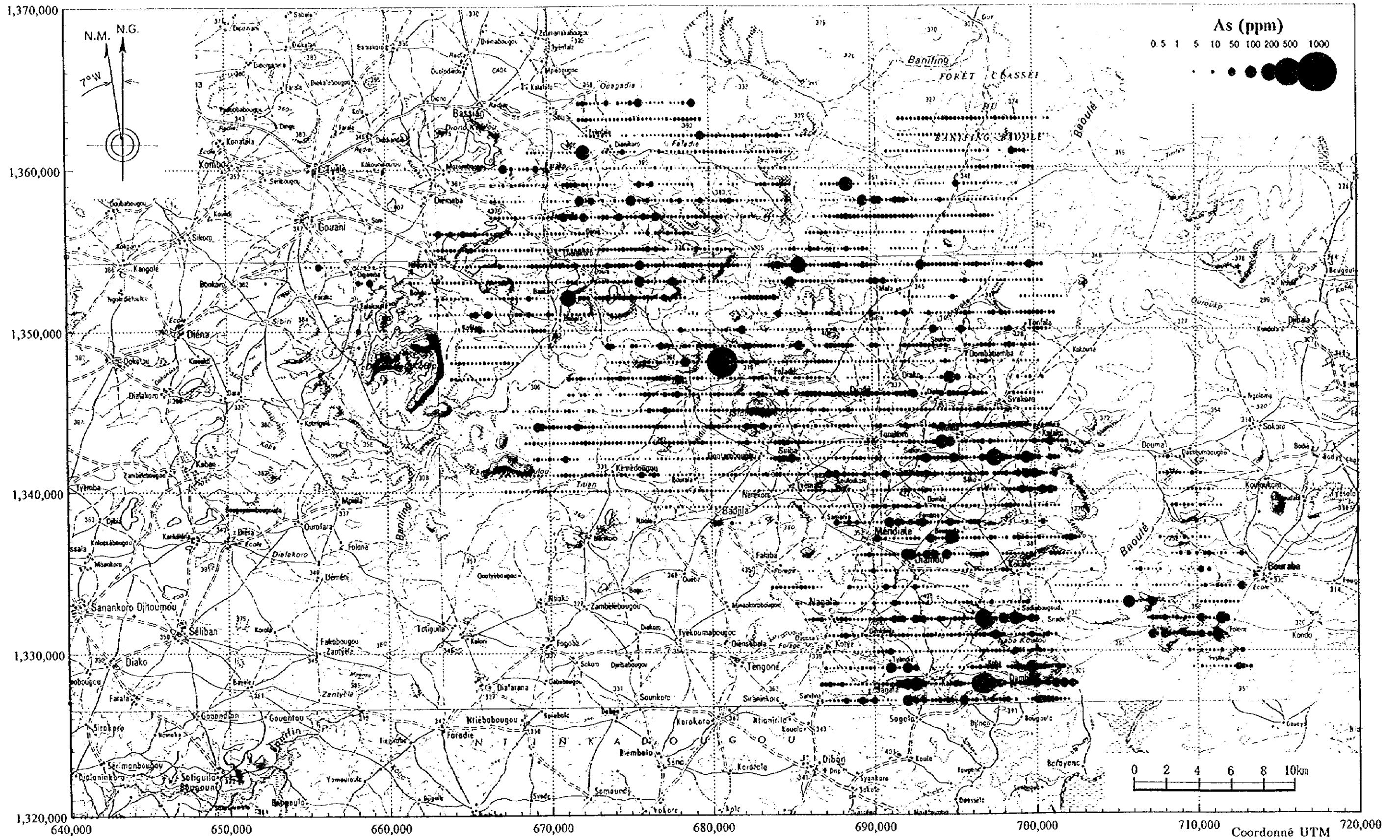
Apc.6-2 Résultat d'analyse géochimique (As, Secteur Est)
