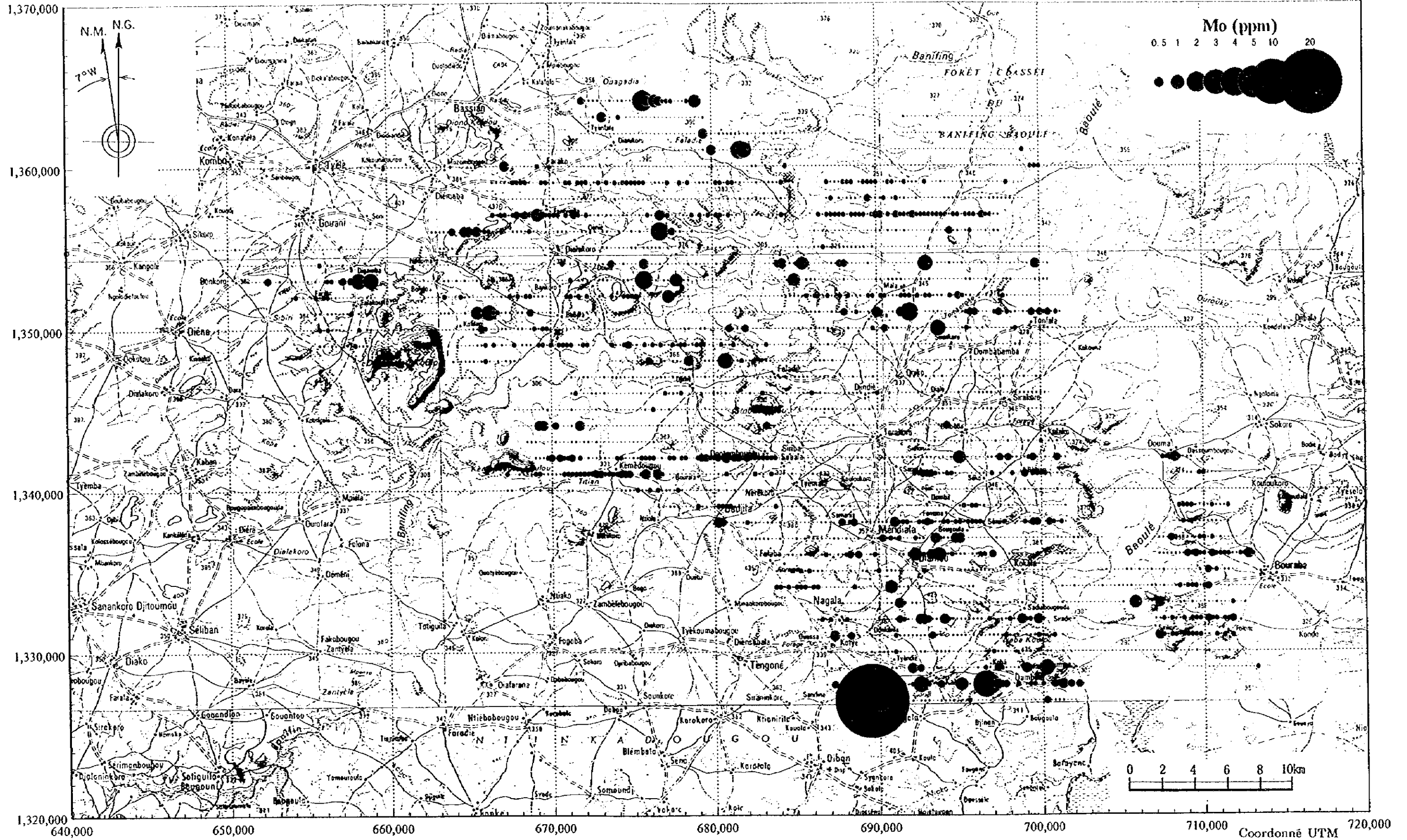
Apc.6-6 Résultat d'analyse géochimique (Mo, Secteur Est)
