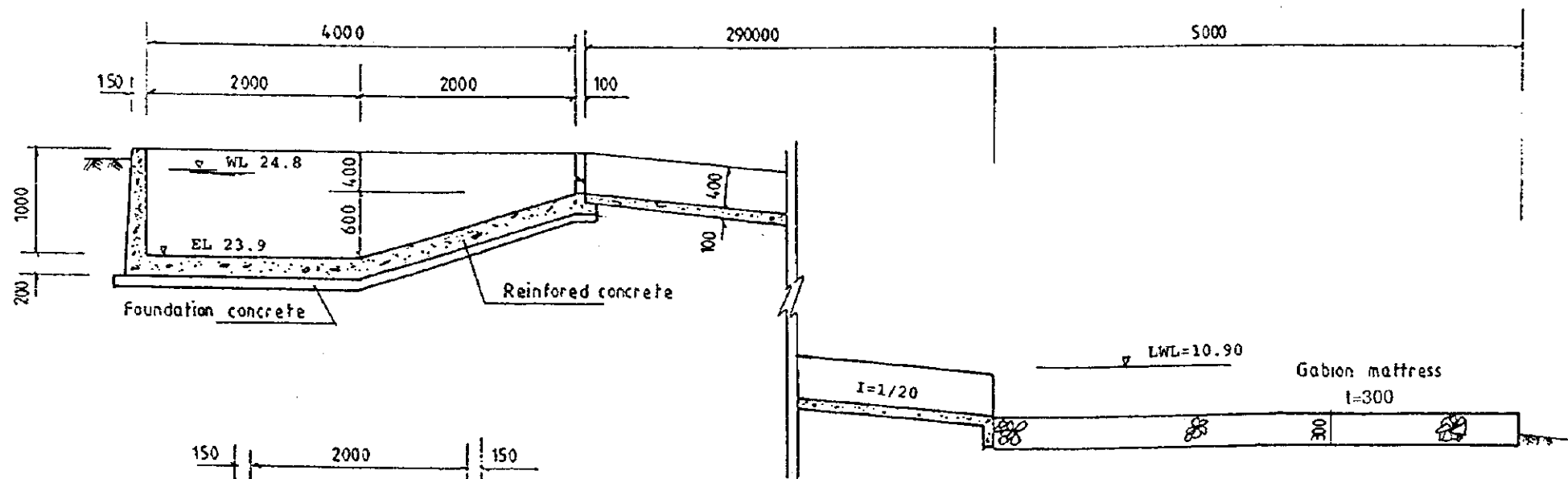
SECTION A-A
