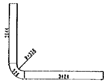
(V1) 15-D32 x 6 600
