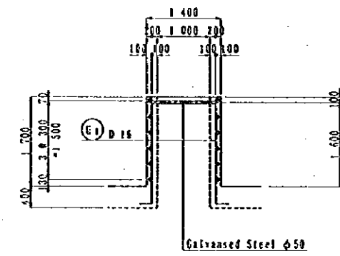
A-A S=1/100
