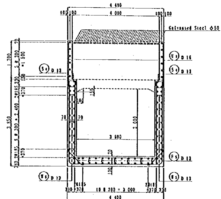
A-A S=1/100
