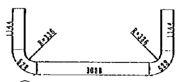
(V1) 10-D32 x 6 440
