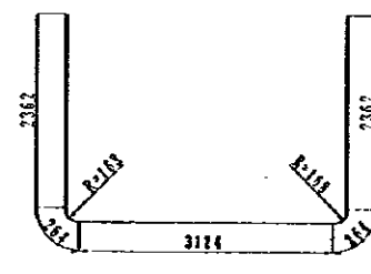
(V11) 7-D16 x 8 380
