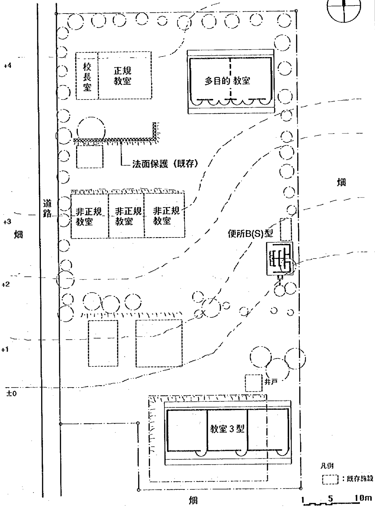
配置図
