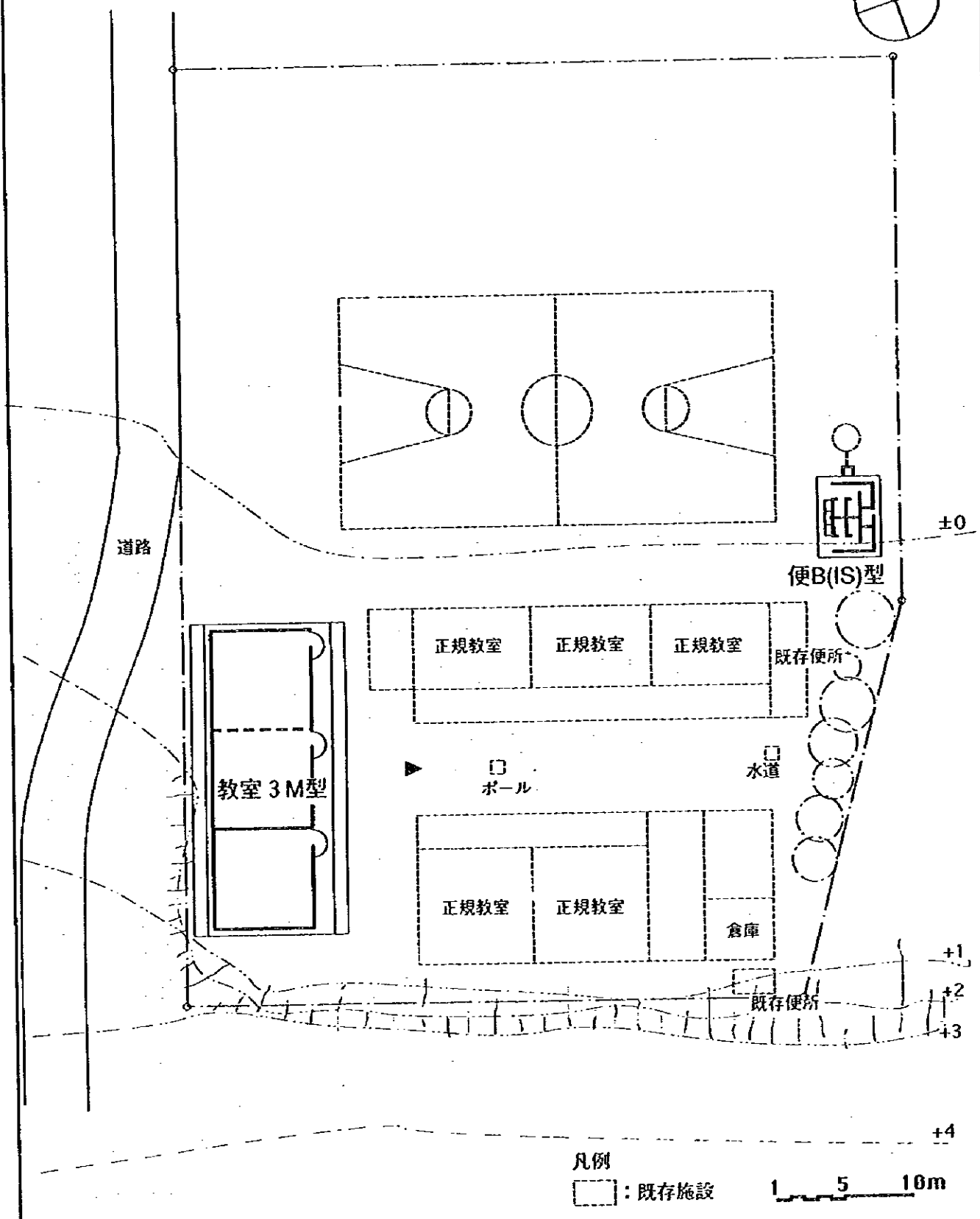
配置図
