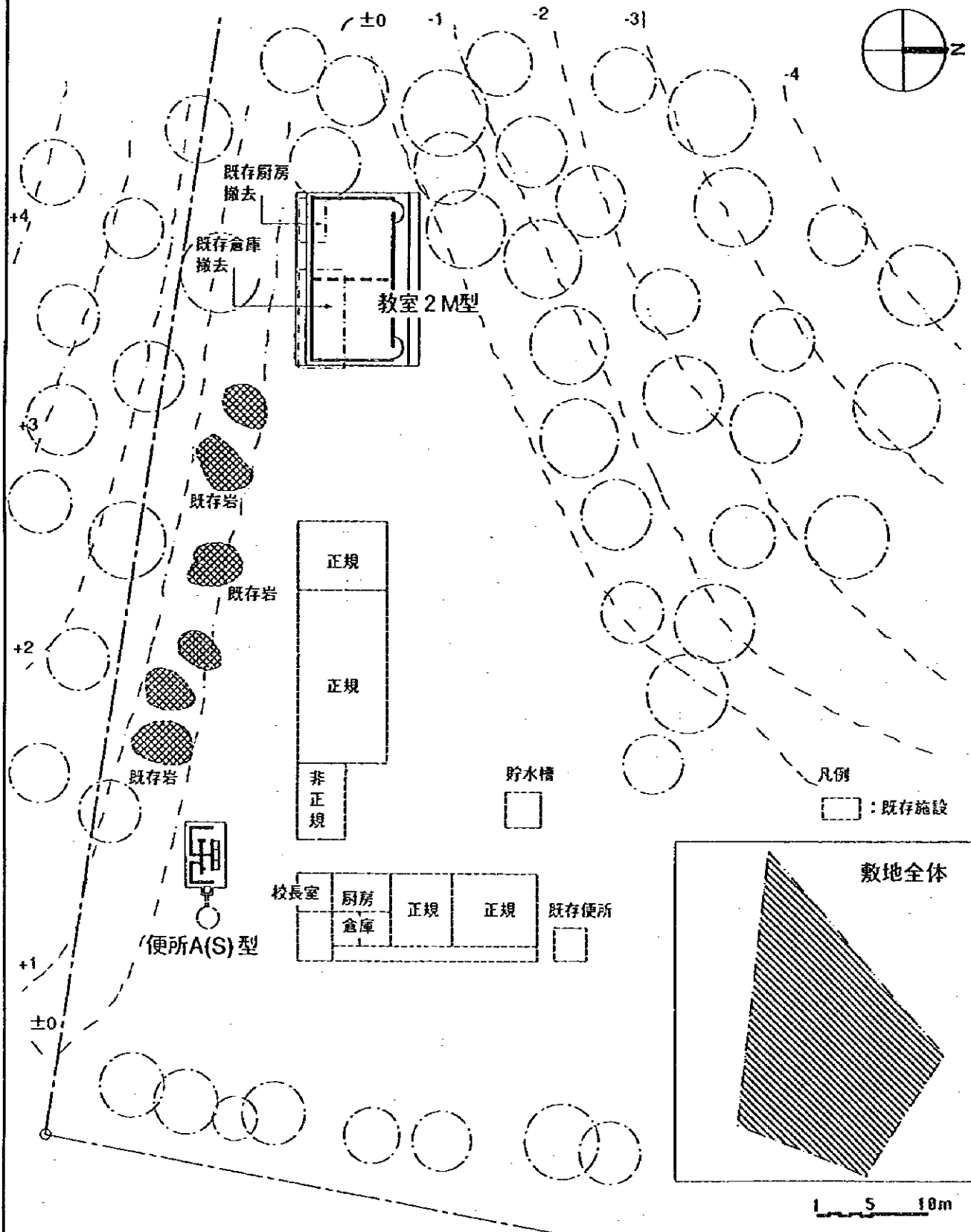
配置図
