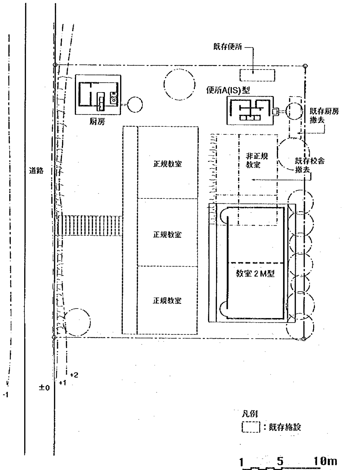
配置図
