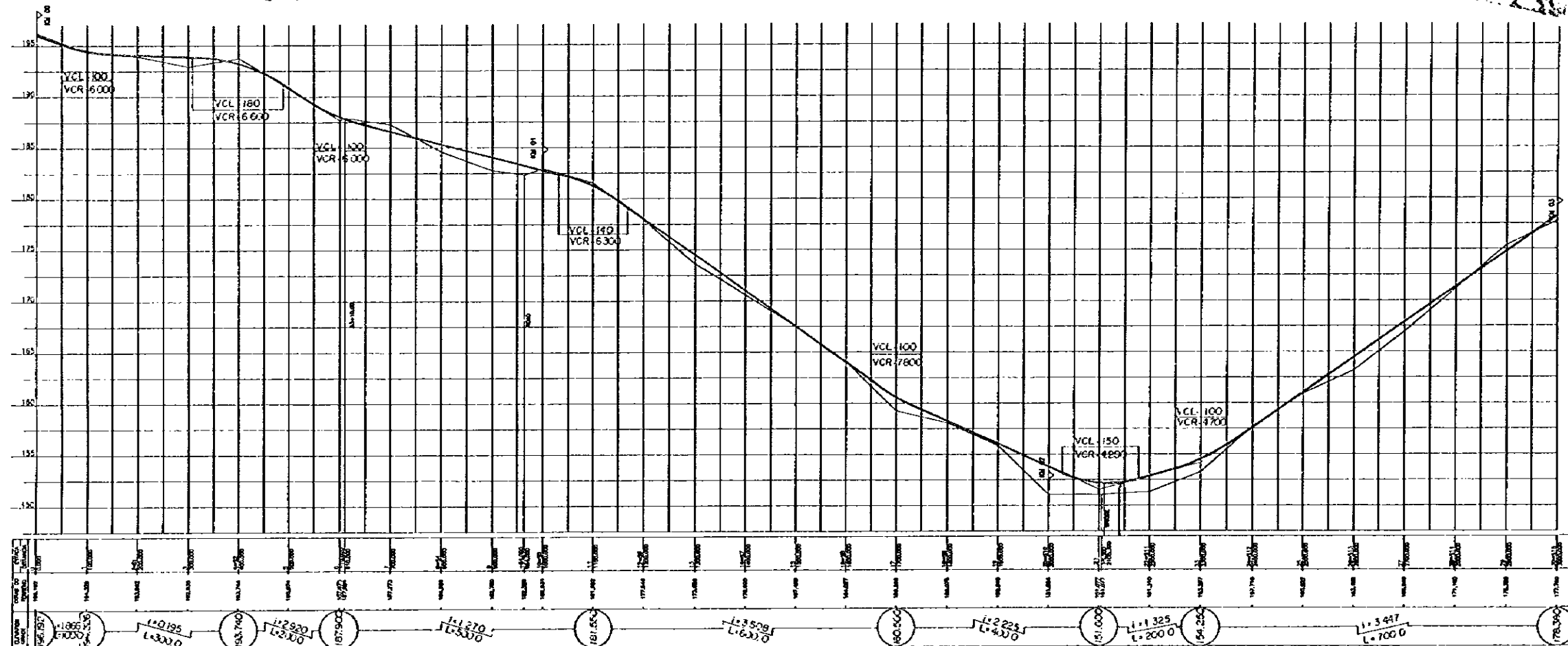
PERFIL PROFILE
