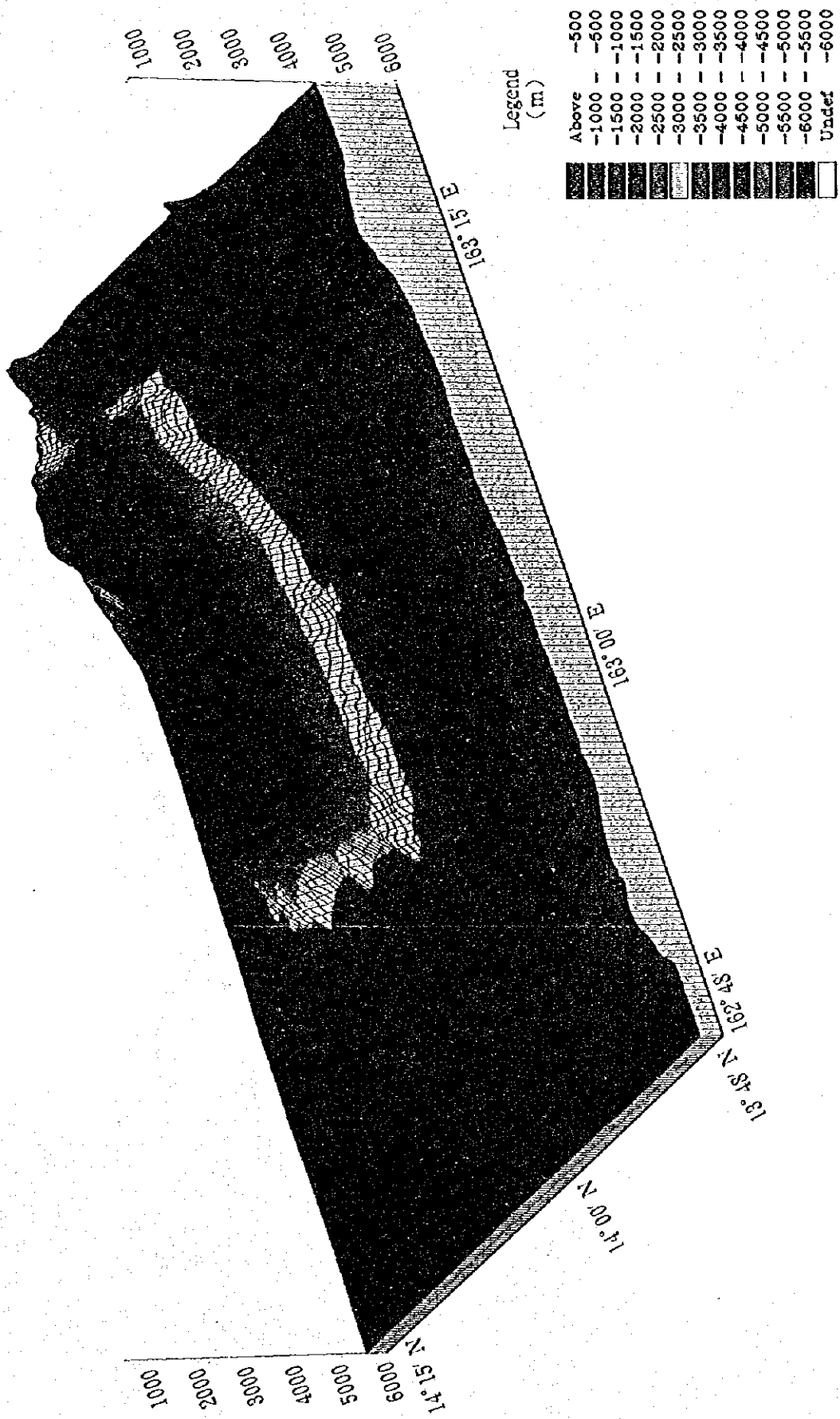
付帯 第3図(2) MS02海山海底地形3次元表現図
