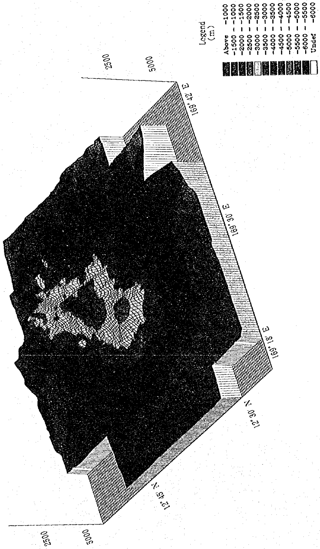
付帯 第3図(7) MS07 海山海底地形3次元表現図
