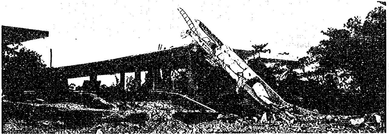
全壊したモスク（於 ビアク市内）
