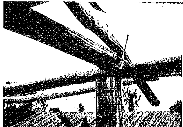
ネルムヌ小学校の仮設校舎の小屋組。近くの山から伐採した丸太の掘立柱で、斧や鋸があれば、誰でもこの程度の工事をする技量をもつ。
