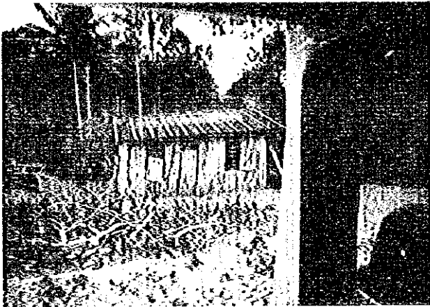
ビアク市～コレム間 内陸部の振動により傾いた木造民家。貫と板壁が転倒を防いでいる。
