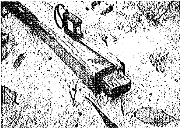
北岸のアモイ村の近くで、流壊した住宅の柱。厚さ1寸、幅2寸、長2寸弱のホゾが刻まれている。
