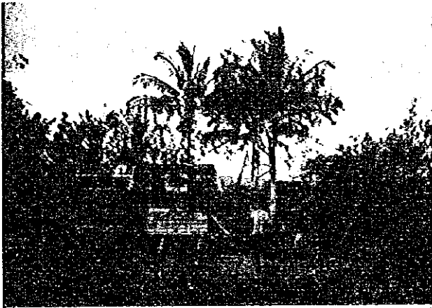
ビアク市～コレム間 内陸部振動により基礎だけが傾いた木造民家。掘立杭の基礎はある種の素朴な免震構造を実現している。
